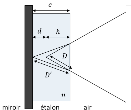
FIGURE 5.17 : Réfraction du faisceau sonde dans l'étalon du VISAR.
