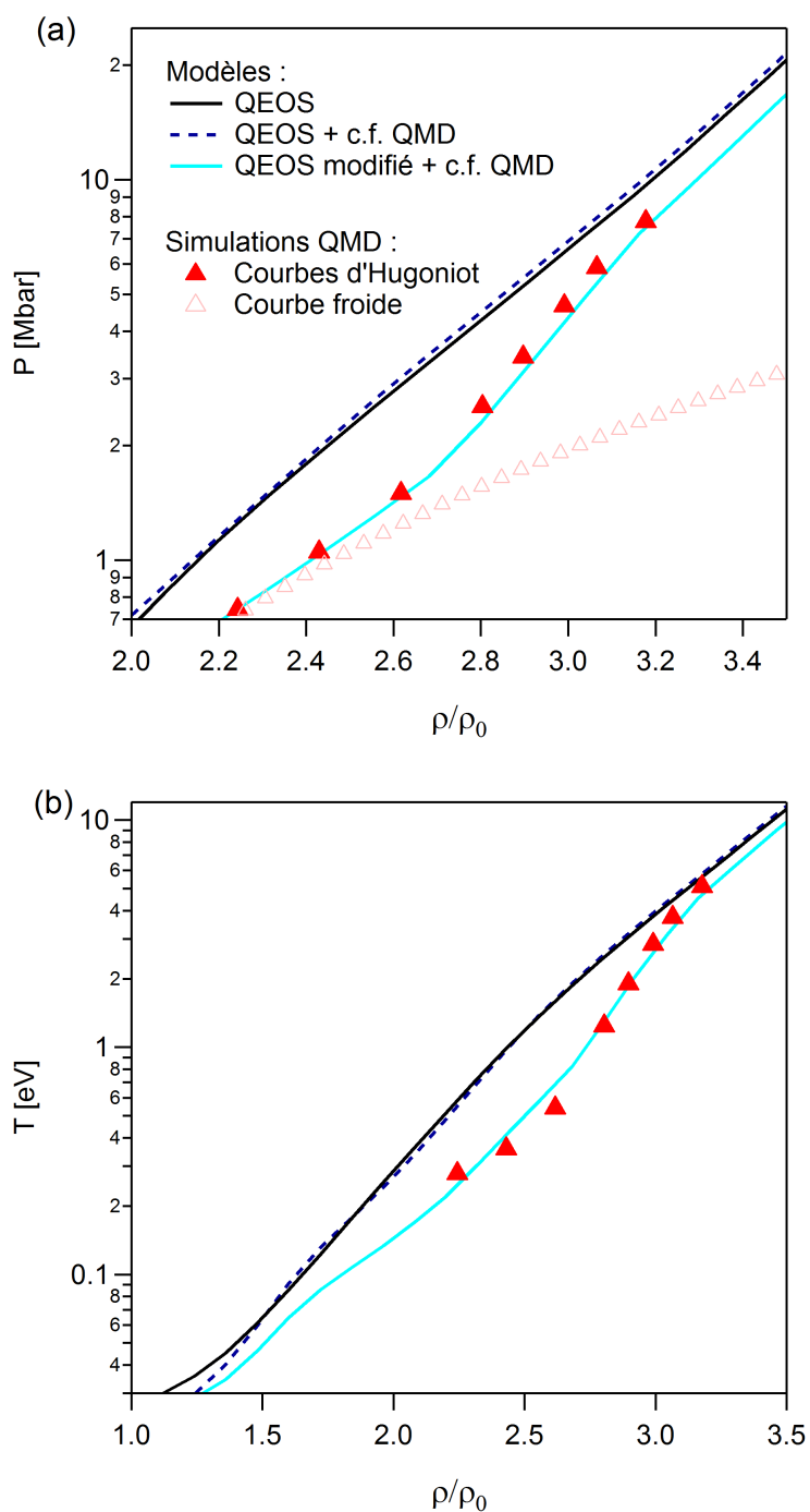
FIGURE 4.18 : Courbes d'Hugoniot de l'ablateur CHO dans le plan pression-compression (a), et le plan température-compression (b). La courbe noire correspond au modèle semi-empirique QEOS sans modification. Les courbes bleues correspondent aux deux modifications apportées à QEOS : en pointillé bleu foncé, l'isotherme à 300 K calculée par QMD a été ajoutée, en bleu clair, l'isotherme à 300 K et le coefficient de Grüneisen effectif ont été ajoutés. Cette dernière modification restitue les valeurs de la QMD sur l'Hugoniot.
