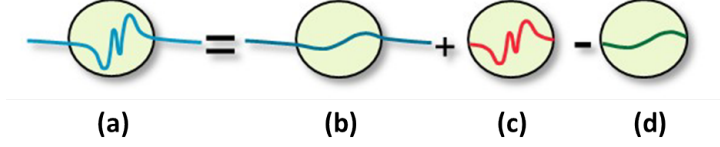
FIGURE 3.9 : Principe de la méthode PAW : la fonction d'onde exacte du système tous électrons (a) est obtenue en calculant une pseudofonction d'onde dans tout l'espace (b). Une transformation remplace ensuite la partie autour du noyau (d) par la fonction d'onde réelle (c) calculée à l'aide d'une base locale.
