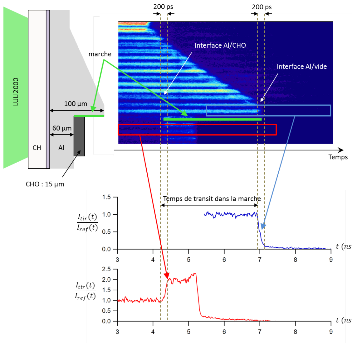
FIGURE 6.2 : Configuration expérimentale et image VISAR correspondante (en haut). Les rapports d'intensité moyennée dans les deux rectangles sont présentés en fonction du temps (en bas).
