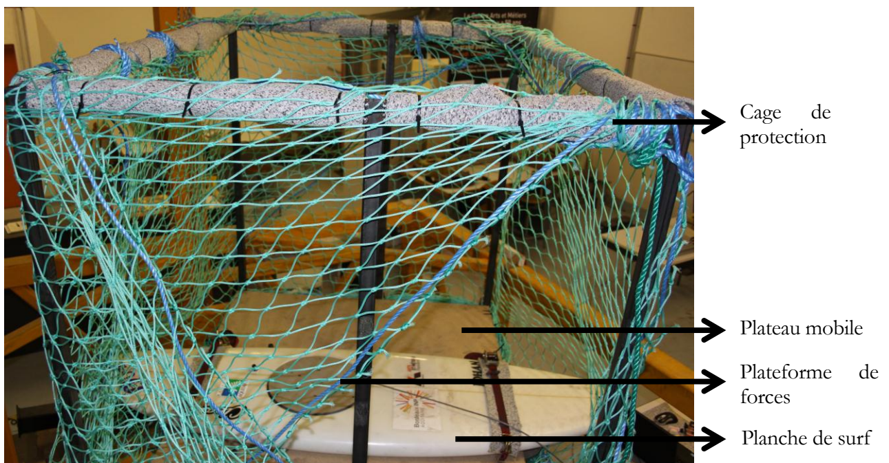
Figure 97 : Environnement « surf » du simulateur
