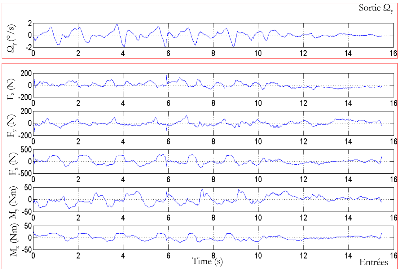
Figure 80 : Exemple de données brutes enregistrées sur une vague pour identifier la sortie \Omega_y en fonction des entrées ( F_x , F_y , F_z , M_x , M_y )
