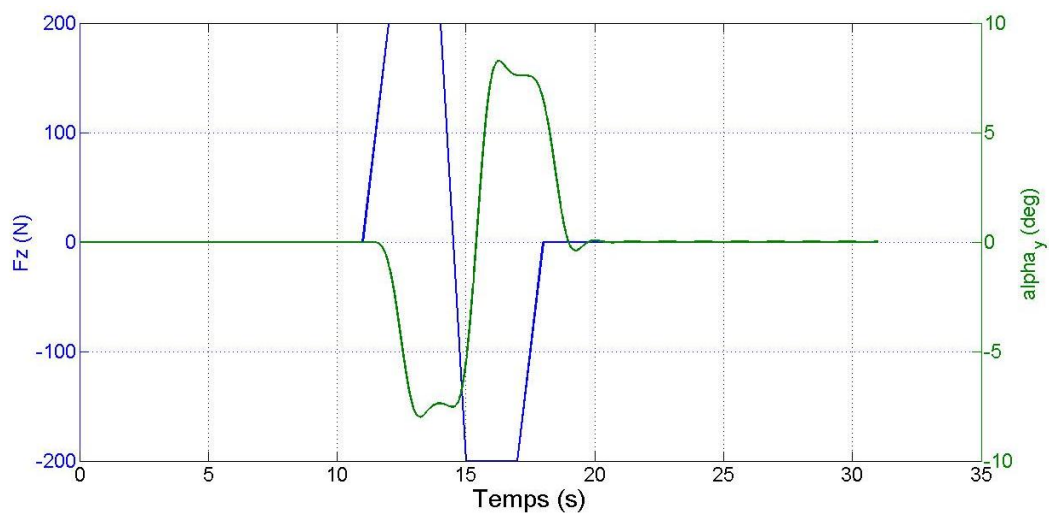
Figure 119 : Simulation numérique d'interactions entre l'appui F_z de l'utilisateur et la trajectoire angulaire de l'hexapode \alpha_y
