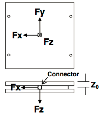
Figure 40 : Plateforme AMTI pour évaluer les étendues de mesure en laboratoire
