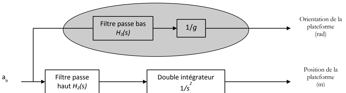
Figure 14: Architecture d'un ARI classique pour une translation longitudinale
