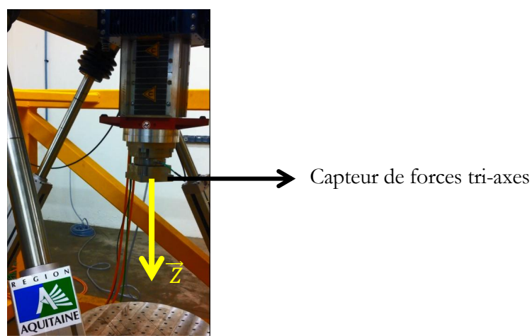
Figure 27 : Capteur de forces tri-axes placé à l'extrémité du 7 ème vérin
