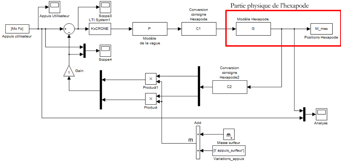
Figure 108 : Modélisation de l'architecture de commande sous Matlab/Simulink
