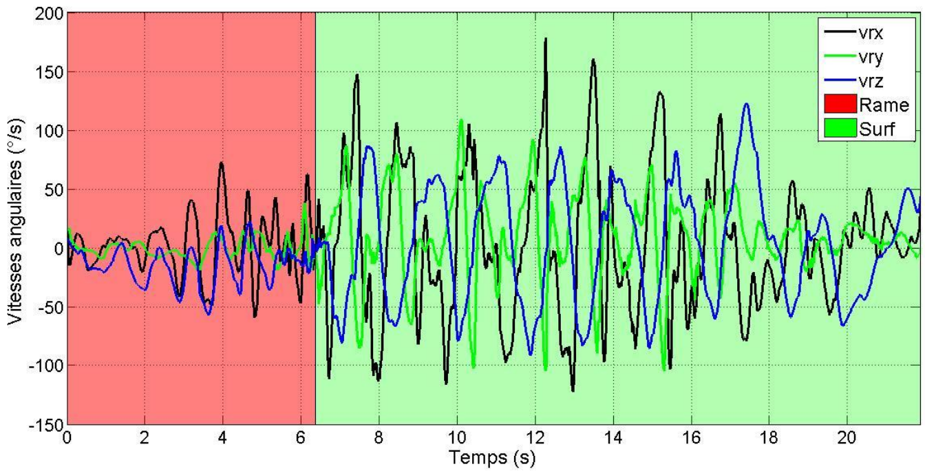
Figure 85 : Vitesses angulaires brutes enregistrées sur une vague de référence
