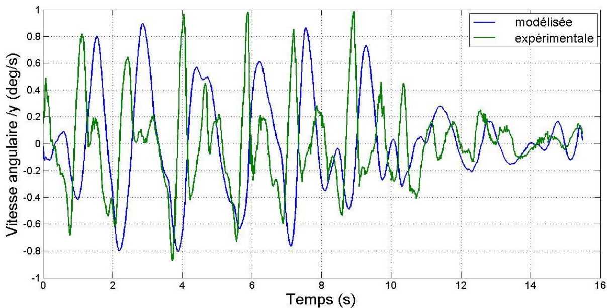
Figure 106 : Comparaison entre la vitesse angulaire \Omega_y expérimentale et modélisée
