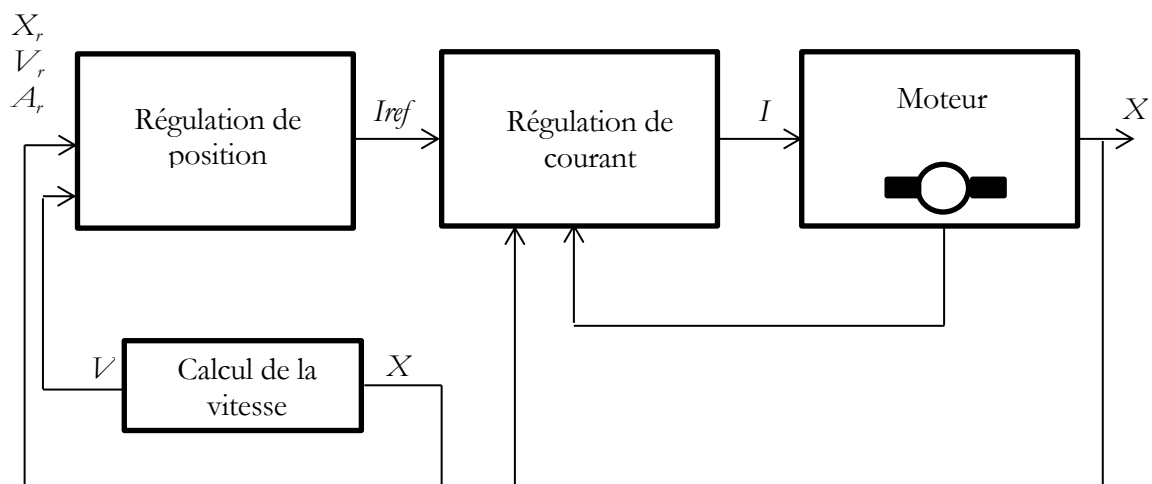
Figure 18 : Principe du contrôleur ETEL (Etel Motion Technologie, 2011)
