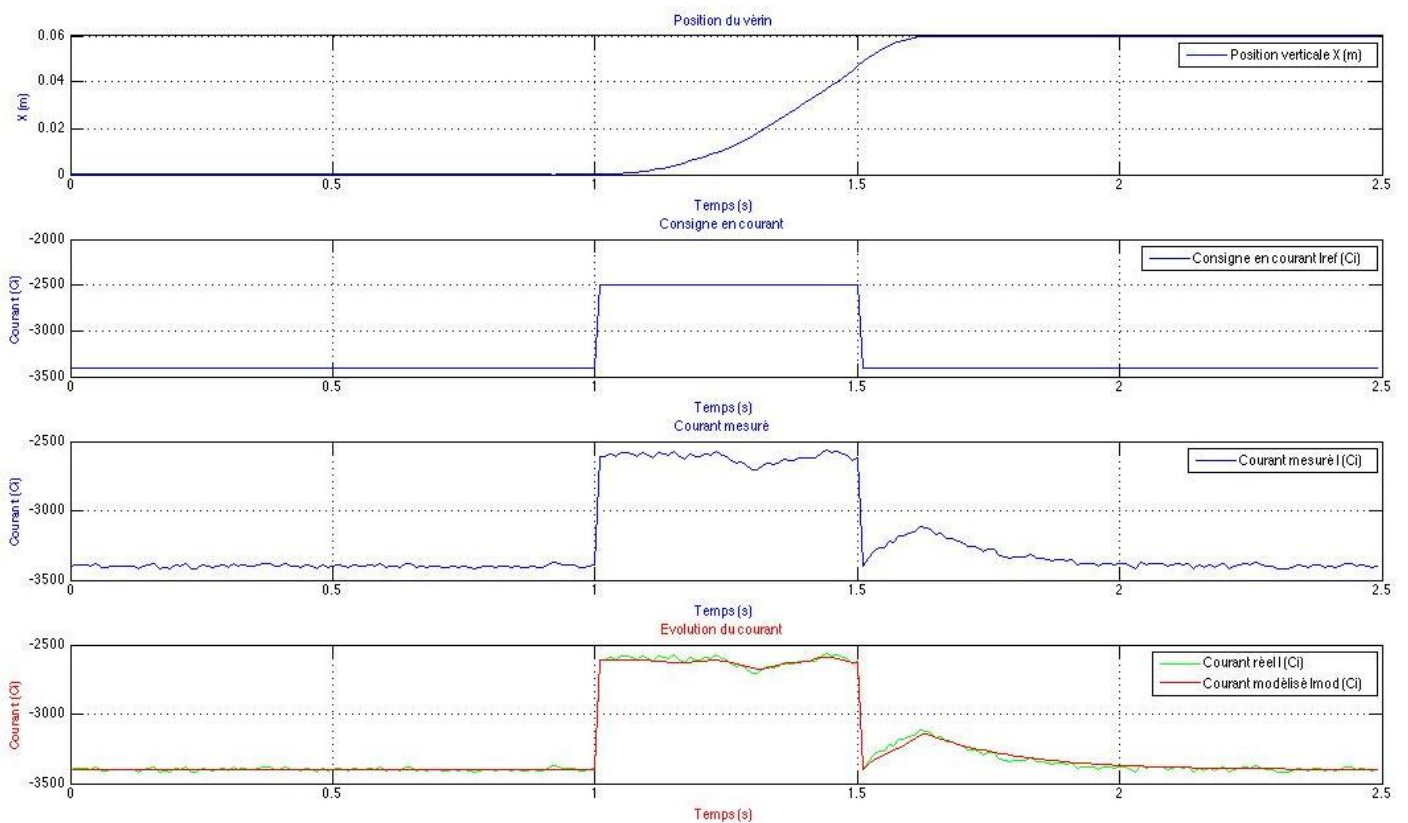
Figure 23 : Comparaison « Courant mesuré » et « Courant modélisé »
