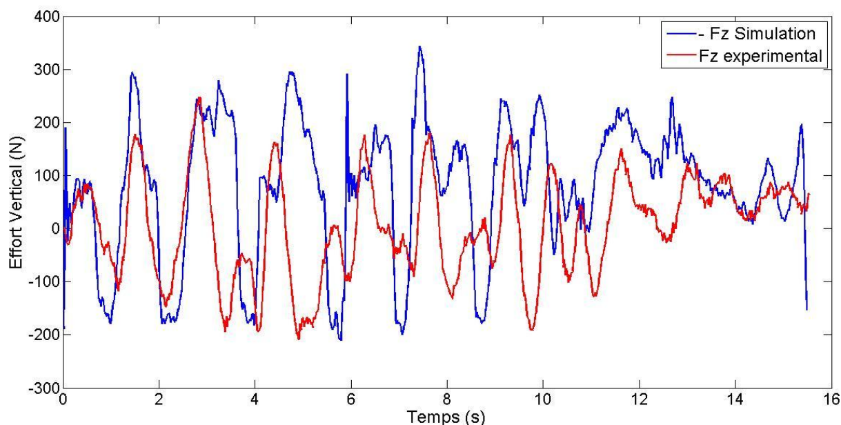
Figure 98 : Comparaison effort vertical en mode suivi de trajectoires en rotation
