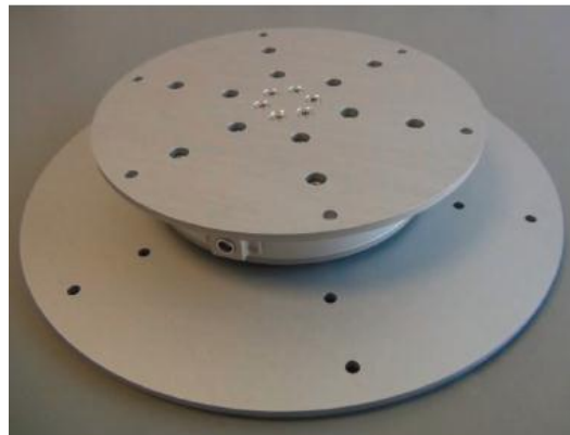
Figure 44 : Photo de la plateforme de force SENSIX
