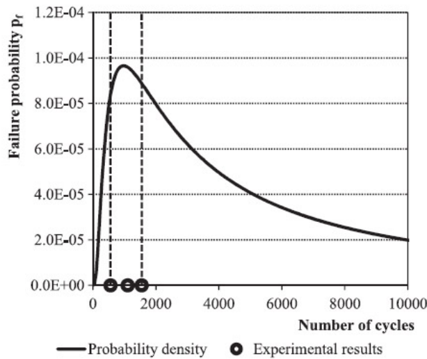
FIGURE 1.22 – Fonction densité de probabilité de durée de vie calculée à partir de la distribution de défauts, Charkaluk et al. [2014].
