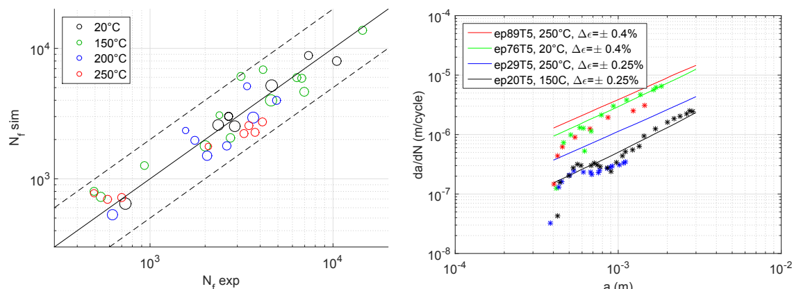
(a) Corrélation expérimentale de la durée de vie simulée et observée pour les éprouvettes sans défauts artificiels. (b) Corrélation de la vitesse de propagation de fissure
