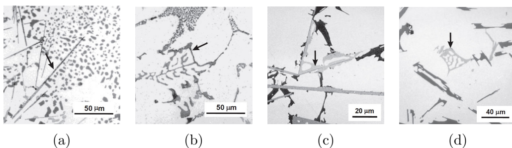
FIGURE 1.5 – Exemples d'intermétalliques dans un alliage AS5U1G ( Taylor [2012] ) (a) plaquelettes \beta - \text{Al}_5\text{FeSi} ; (b) écritures chinoises \alpha - \text{Al}_8\text{FeMg}_3\text{Si}_6 ; (c) phase \pi - \text{Al}_8\text{FeMg}_3\text{Si}_6 ; (d) phase \pi en écriture chinoises
