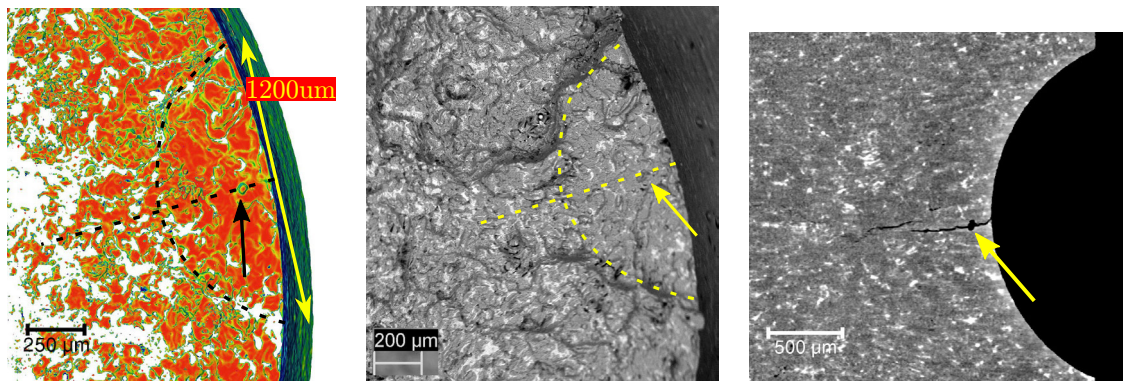
(a) Reconstruction de la fissure basée sur la tomographie.
