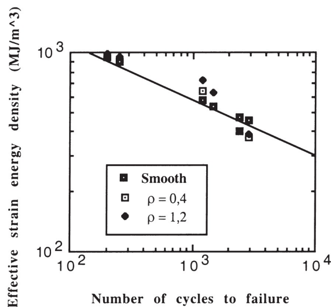
FIGURE 6.36 – Nombre de cycles à rupture en fonction de l'énergie de déformation plastique calculée (énergie effective dans les cas d'éprouvettes entaillées. Le trait plein correspond à la régression sur les essais sur éprouvettes lisses, Bentachfine [1999] )
