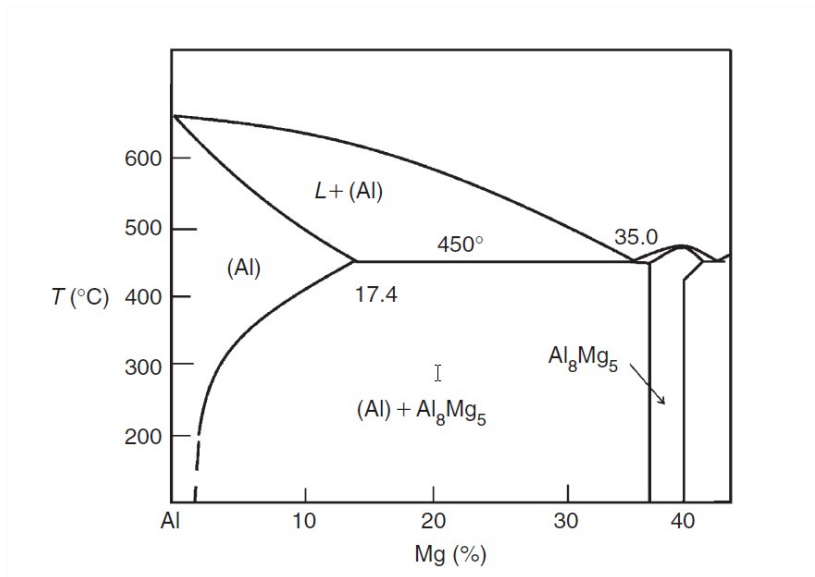
FIGURE 1.4 – Diagramme de Phases du système Al-Mg Zolotarevsky et al. [2007]
