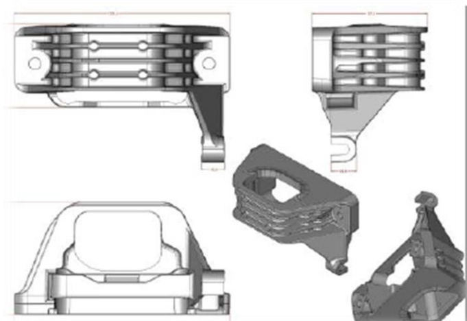
Figure 27: Pièce coulée
