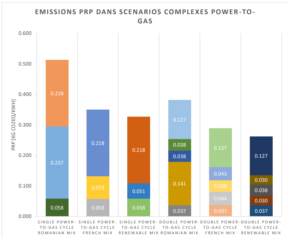
Figure 10.2 Emissions PRP de la production d'électricité dans scénarios complexes Power-to-Gas en employant le carbone fossile des centrales électriques
