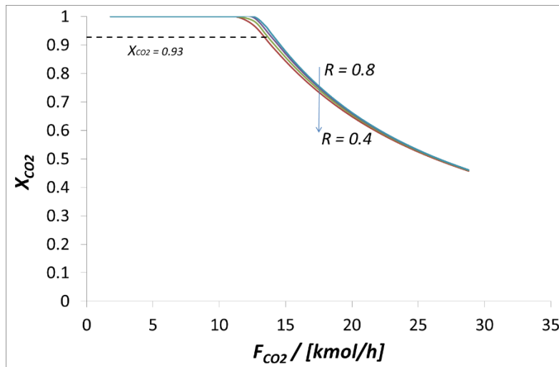
Figure 7.4 Conversion CO_2 versus le débit de dioxyde de carbone à l'entrée du premier réacteur à un rapport différent du recycle. F_{1,H_2} = 54 kmol/h (108 kg/h)
