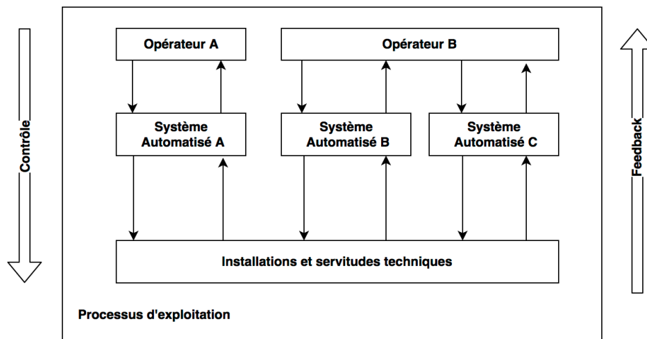
Figure 4-2 Structure de contrôle du processus d'exploitation et d'opération
