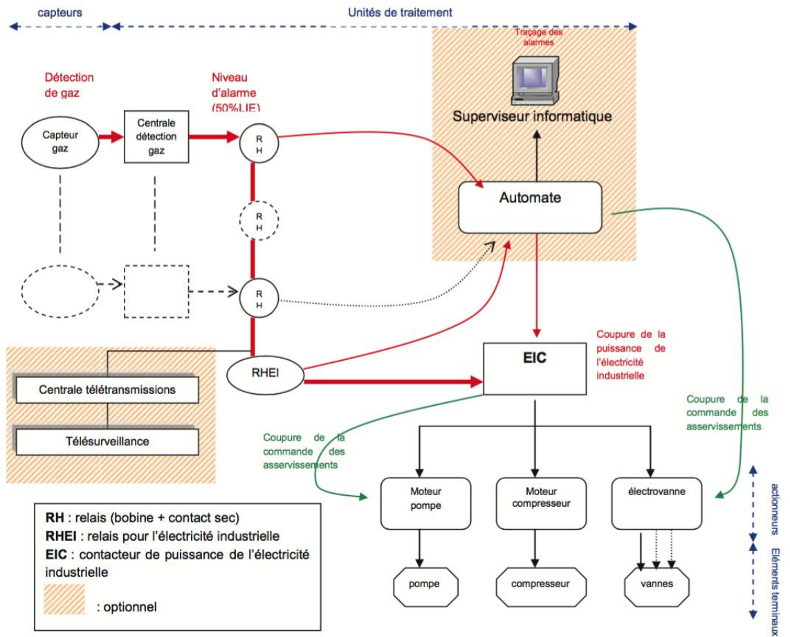
Figure 3-6 La chaîne de détection de gaz
