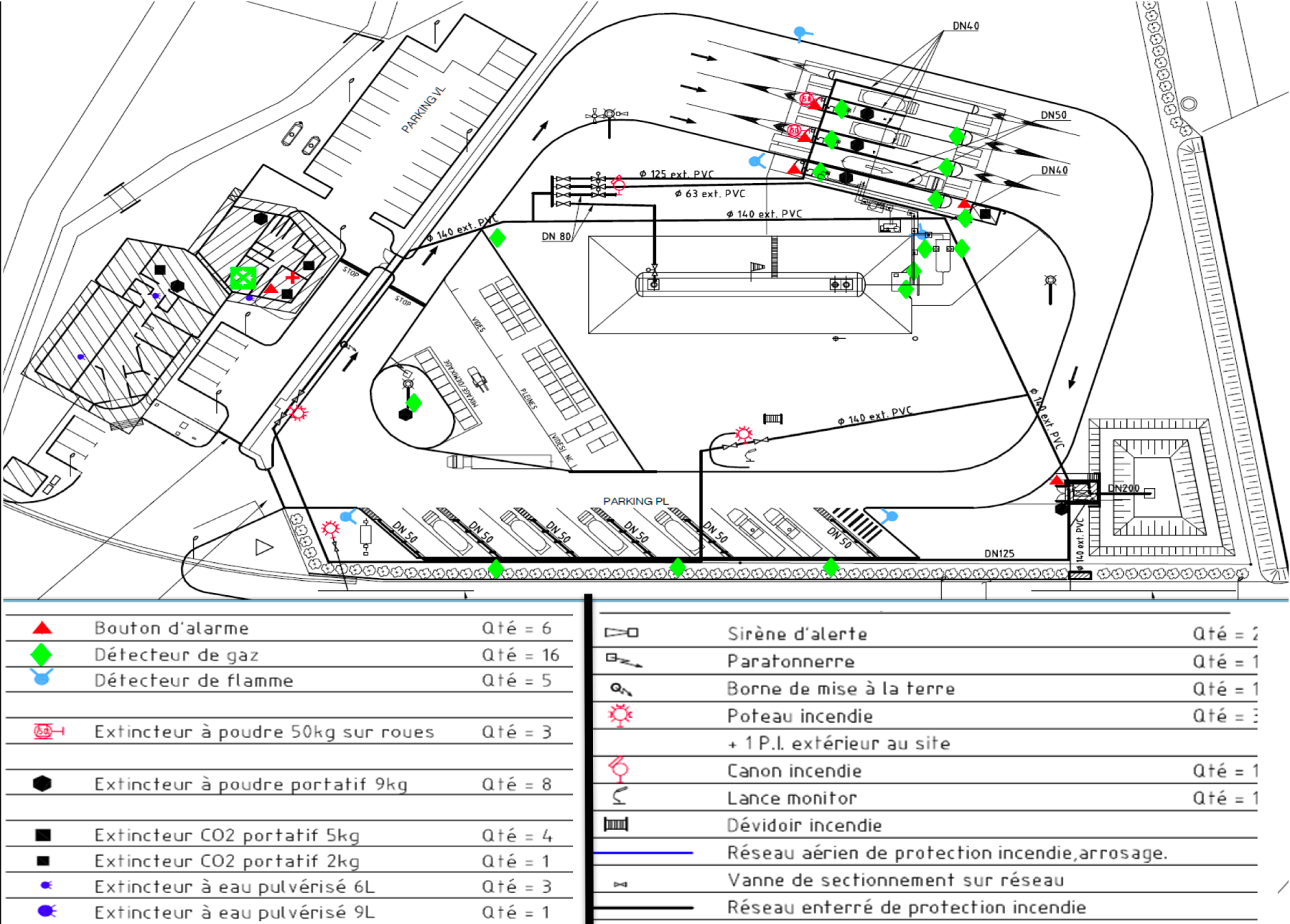
Figure 3-7 Implantation détecteurs
