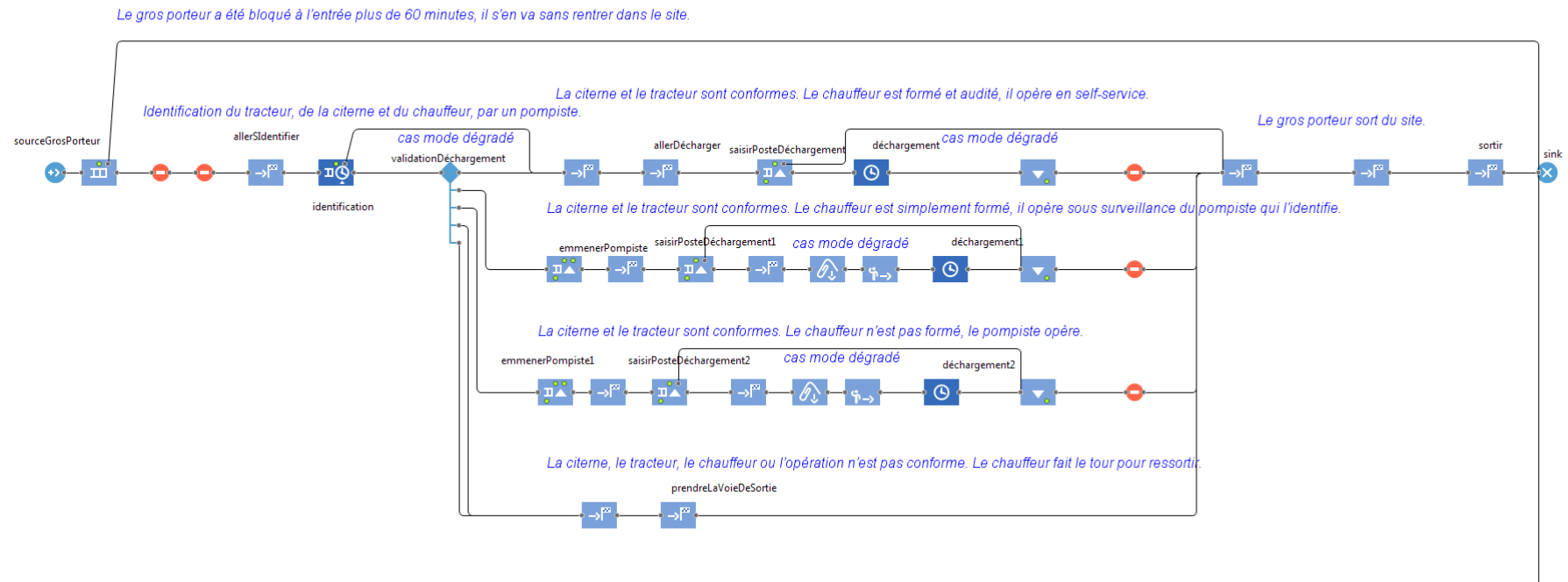
Figure 5-7 Partie SED du Main distinguant les différentes branches possibles selon le niveau de formation du chauffeur du camion gros porteur
