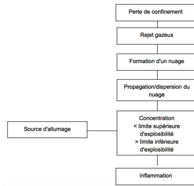
Figure 4-8 Les causes d'un UVCE
