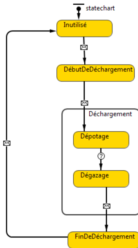
Figure 5-25 Diagramme états-transitions procédural du poste de déchargement
