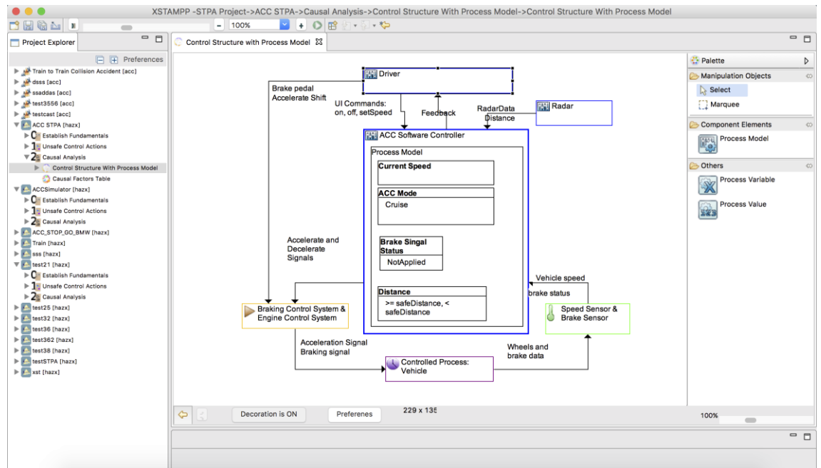
Figure 2-8 Interface du logiciel XSTAMPP pour une étude STPA
