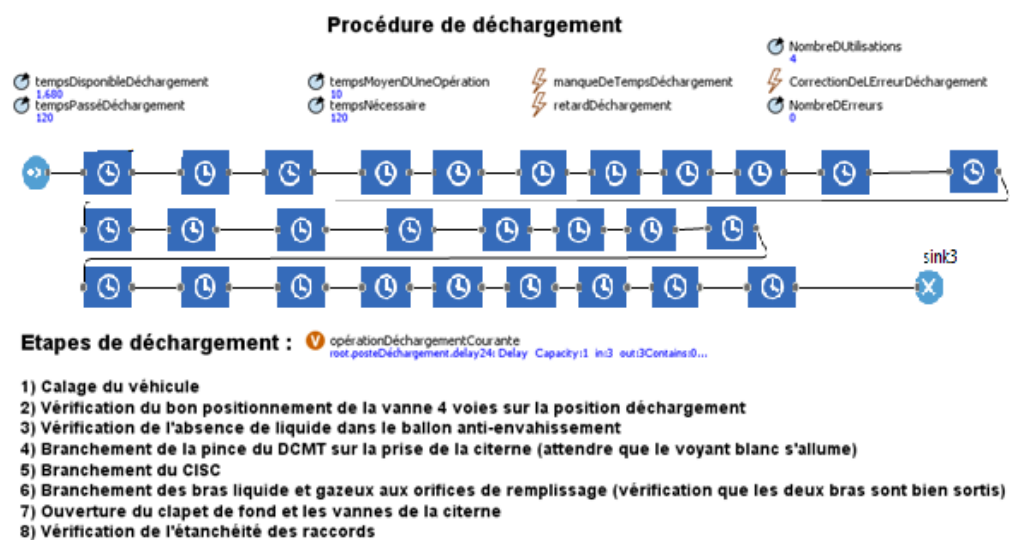
Figure 5-28 Début de déchargement. Vue en système d'événements discrets.
