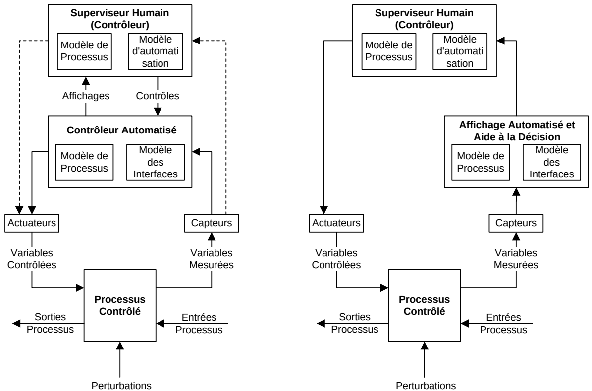
(a) Automatisation émettant directement des commandes sous la supervision d'un contrôleur humain
