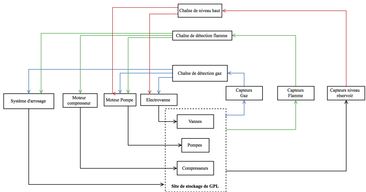
Figure 4-11 Exemple de la structure de contrôle de la sécurité au niveau du système d'exploitation
