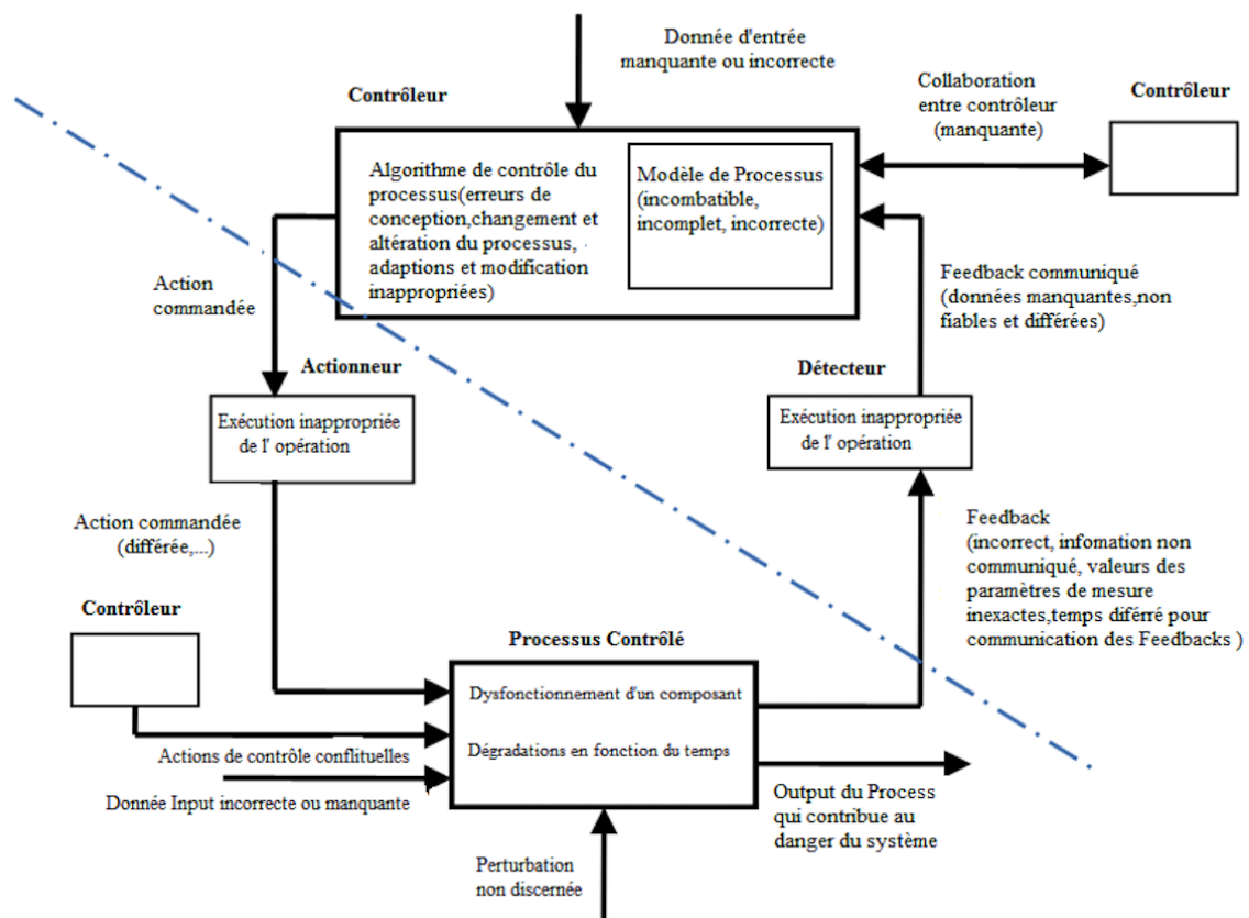
Figure 4-5 Classification des facteurs de causalité contribuant aux dangers
