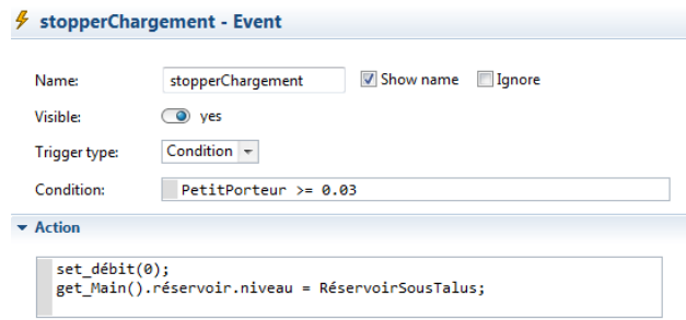
Figure 5-31 Propriété de l'événement « StopperChargement » déclenché par condition (le petit porteur est rempli quand il atteint 3% du volume du réservoir.
