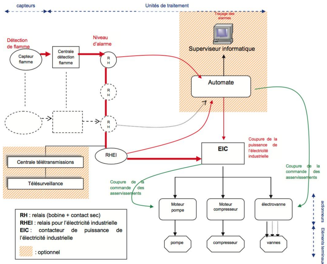
Figure 3-8 La chaîne de détection de flamme
