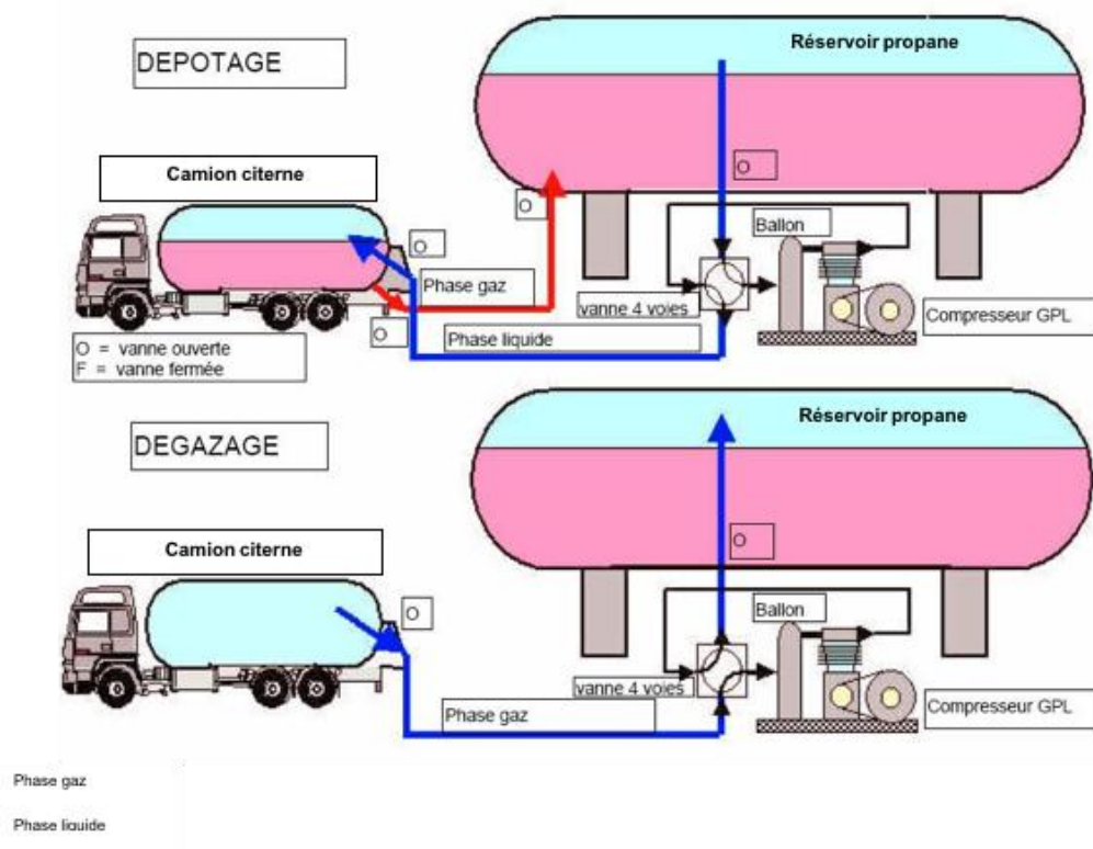
Figure 3-5 Présentation des deux phases de déchargement des camions gros Porteurs
