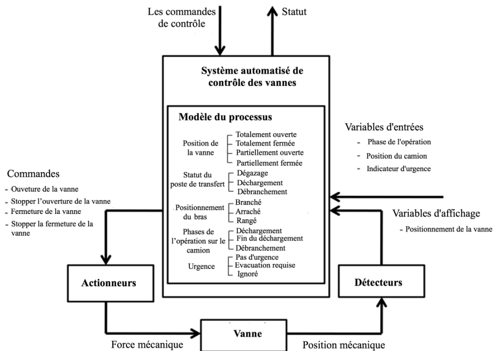
Figure 4-3 Boucle de contrôle de la sécurité
