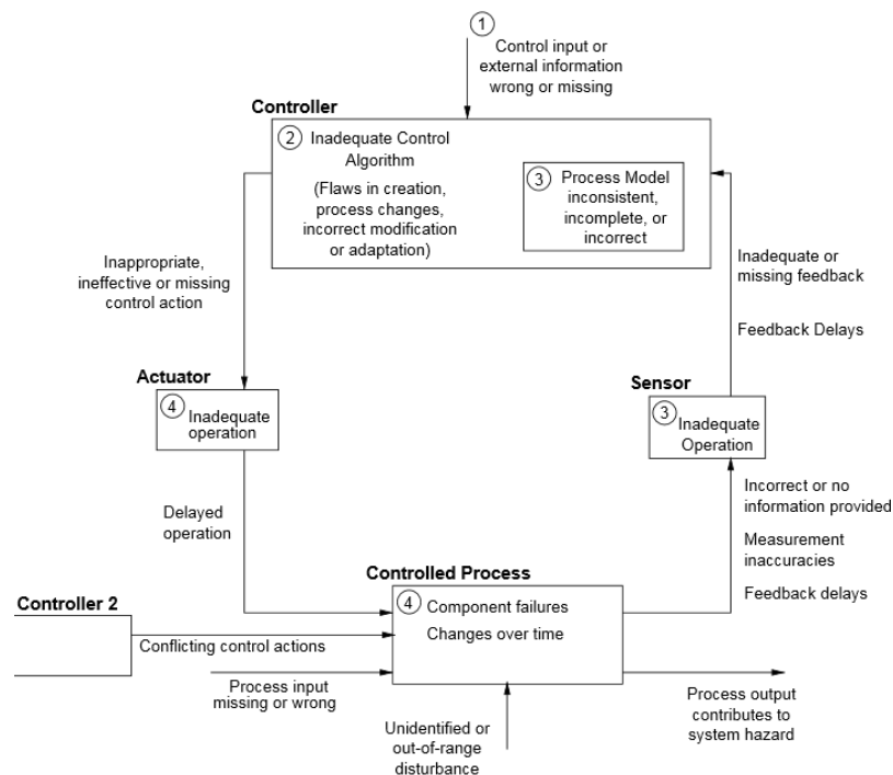
Figure 2-5 Les causes des problèmes de manque de contrôle
