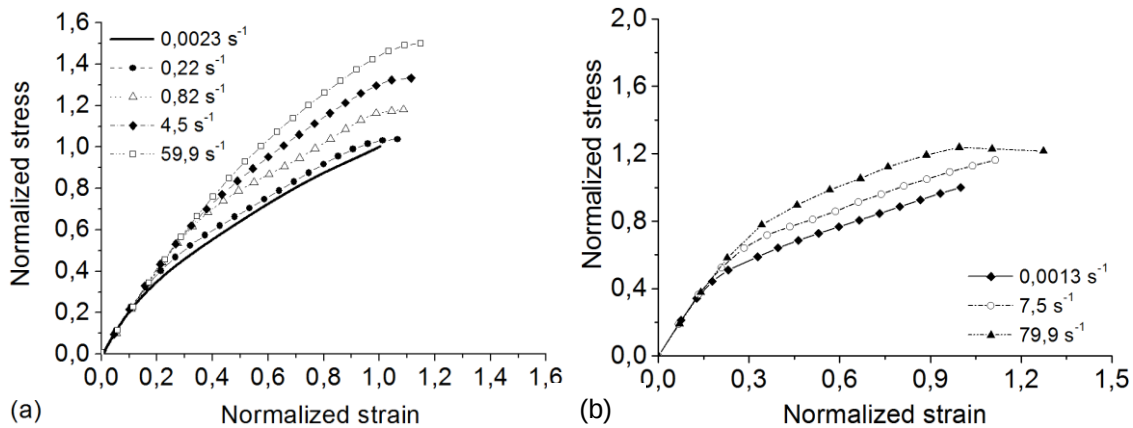
Figure 23 Courbe de traction aux vitesses de déformation différentes : RO-A-SMC (a) et RO-LD-SMC (b), ( \sigma_{\text{normalisée}} = \sigma / \sigma_{r(\text{RO en QS})} ) et ( \epsilon_{\text{normalisée}} = \epsilon / \epsilon_{r(\text{RO en QS})} )).
