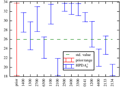
(d) A_0^+ of the Baldwin-Lomax model.
