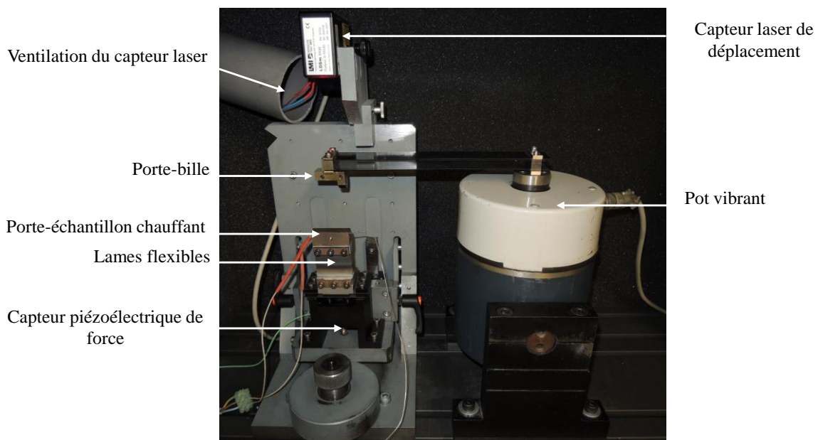
Figure II.14 : Tribomètre d'impact-glissement.
