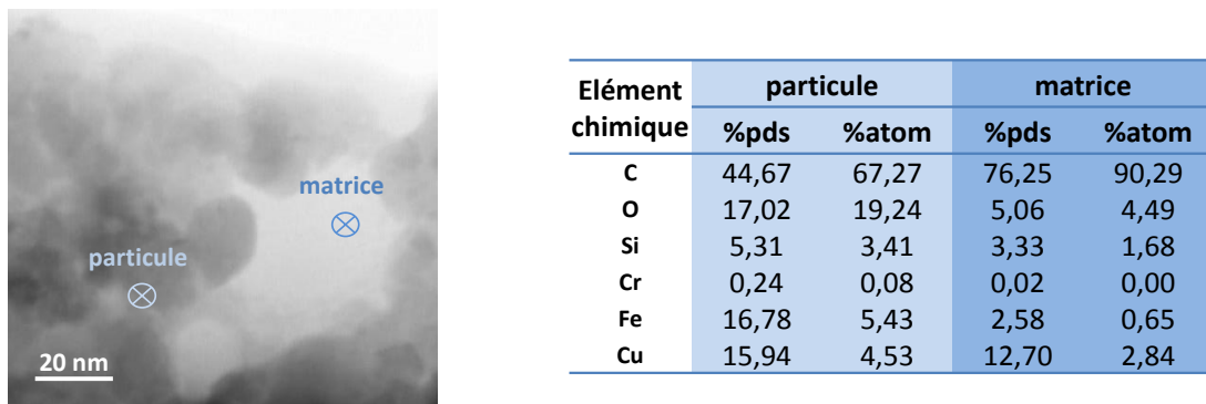
Figure IV.42 : Image MET STEM en fond clair de particules élémentaires. Le tableau répertorie les quantités d'éléments présents mesurées par analyse EDX.
