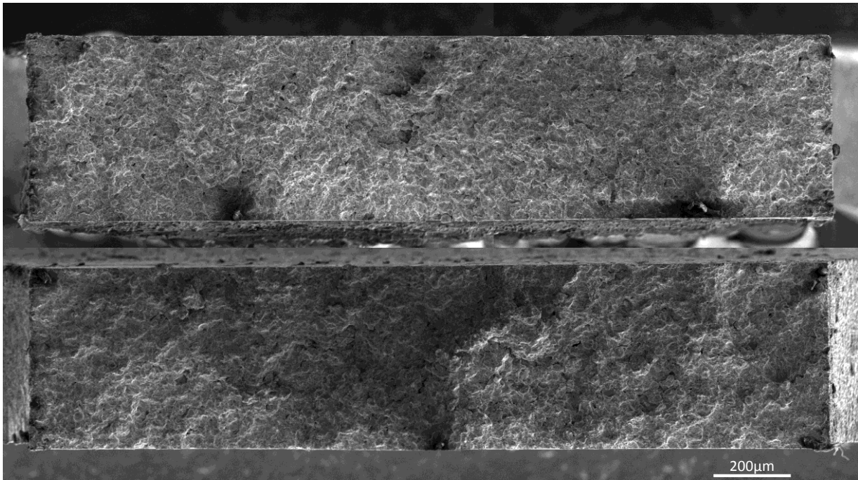
Figure IV.14 : Image MEB en vue de dessus des deux faciès complémentaires de rupture d'une éprouvette de composition 316L+13%Cu+4%Ni700.
