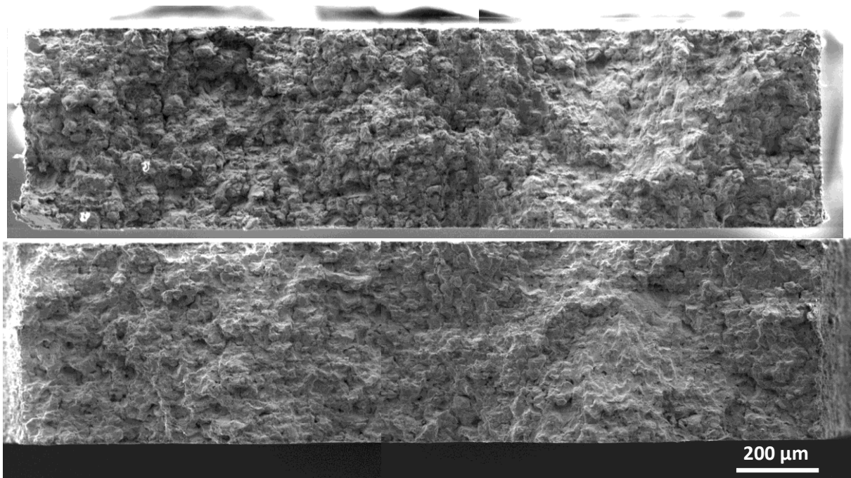
Figure IV.12 : Image MEB en vue de dessus des deux faciès complémentaires de rupture d'une éprouvette de composition 316L+13%Cu.
