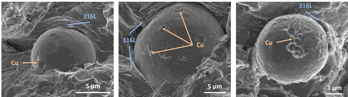
Figure IV.15 : Images MEB en vue de dessus d'un faciès de rupture centrées sur des particules de Ni700 avec du Cu en surface dans une matrice 316L.
