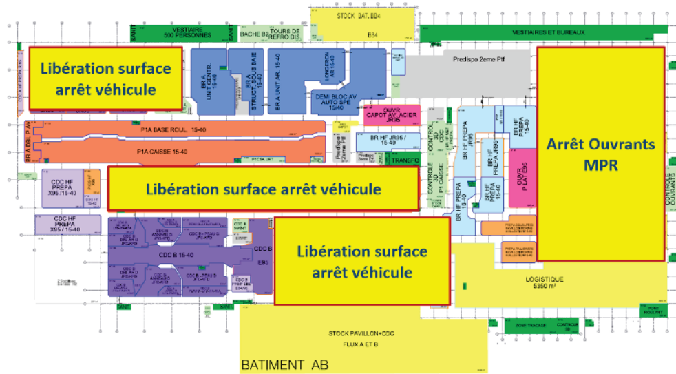
Figure V.7 – Revue globale d'architecture d'implantation d'atelier
