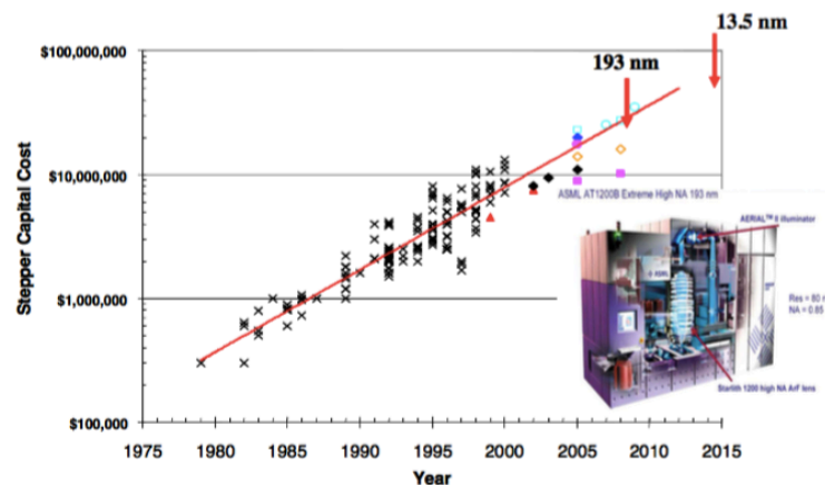
Figure 28 : Evolution des coûts d'équipements de photolithographie en fonction des nœuds technologiques
