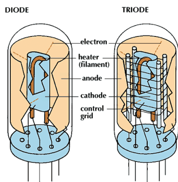
Figure 158: schéma illustrant une diode et triode
