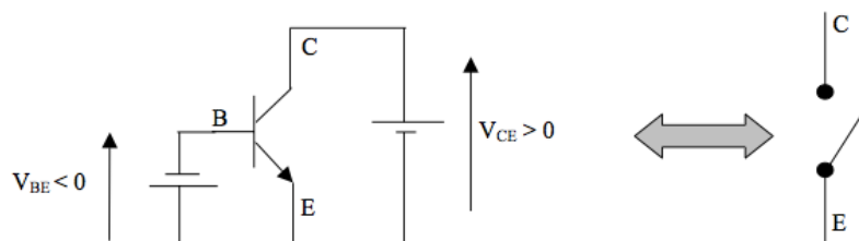
Figure 175: Etat bloqué – transistor bipolaire NPN
