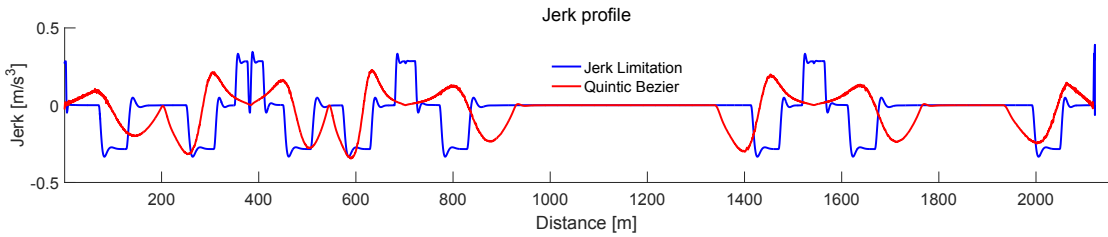
(d) Jerk profile comparison of both methods
