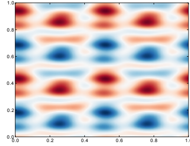
(d) TDLDA susceptibility, \omega = 25.6eV
