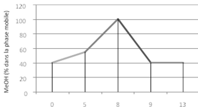
Figure 3 : Gradient d'éluant présentant le pourcentage de méthanol dans la phase mobile en fonction du temps (Geara-Matta, 2012)
