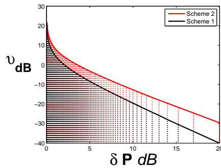
Figure 5: Région d'interférence pour un gain en débit de 100% en fonction de \delta P_{dB}
