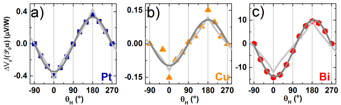
Figure 33 Comparatif de la tension mesurée sur l'électrode de (a) platine 50nm, (b) cuivre 20nm et c) Bismuth 200nm en fonction de l'angle du champ magnétique pour un champ de 1T. Afin de rendre les amplitudes comparables, nous avons normalisé la tension mesurée par la puissance injectée et l'effet de court-circuit de l'électrode (Pham, 2014). La courbe gris clair est un ajustement obtenu correspondant à \cos \theta , avec \theta l'angle hors du plan de l'aimantation obtenu grâce au programme Scilab présenté dans la partie théorique. La courbe gris foncé correspond à \cos \theta_H .
