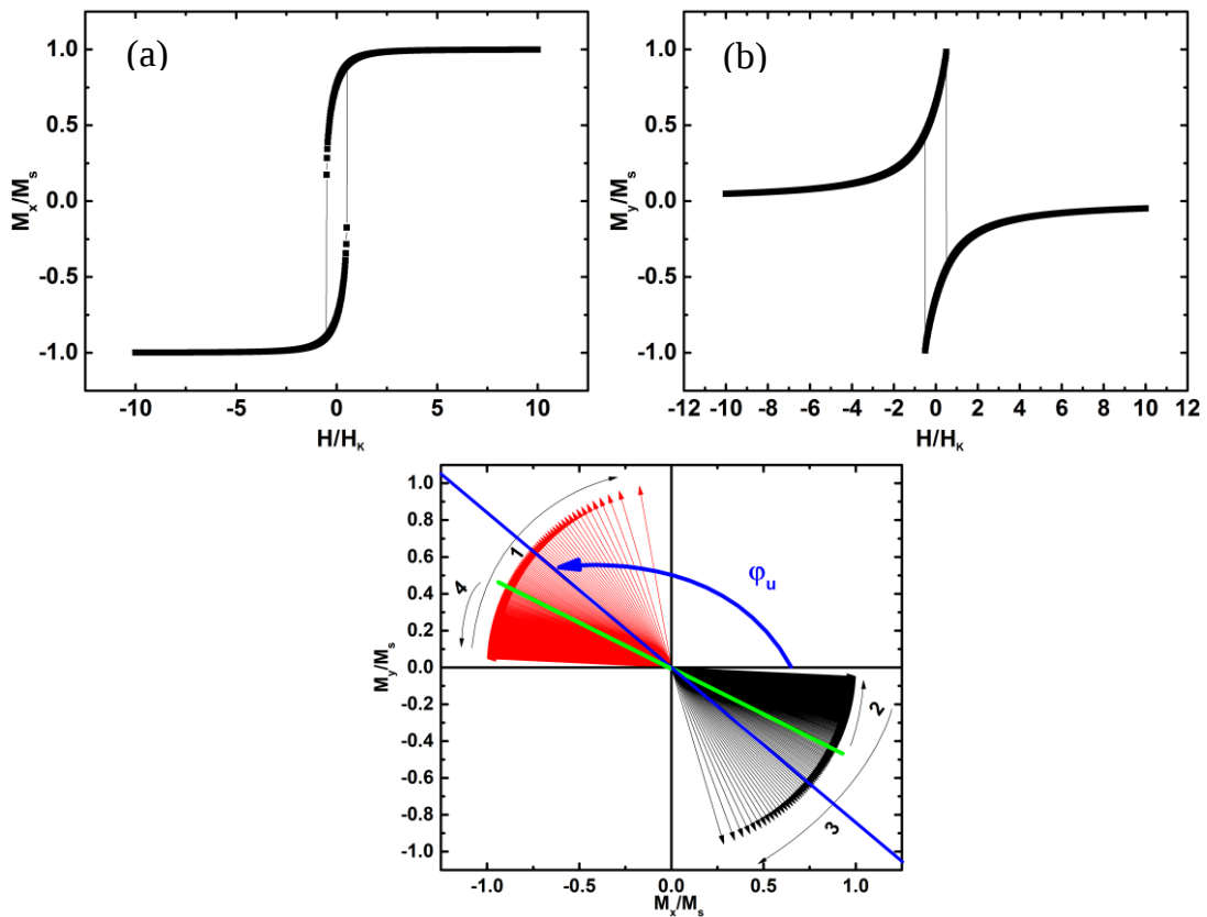
Figure 13 (a) composante selon x de l'aimantation, (b) composante selon y de l'aimantation en fonction du champ magnétique appliqué le long de x et normalisé par l'amplitude de l'anisotropie uniaxiale H_k (c) orientation de l'aimantation représentée par des flèches dans le plan (xy) . Le balayage en champ utilisé pour manipuler l'aimantation correspond à celui des cadrans (a) et (b). Le balayage est le suivant : 1 : champs de -10K à 0,5K ; 2 : champs de 0,5K à 10K ; 3 : champs de 10K à -0,5K et 4 : champs de -0,6K à -10K . L'axe bleu correspond à l'axe de l'anisotropie uniaxiale, tandis que l'axe vert correspond à la position de l'aimantation lors du saut de l'aimantation.
