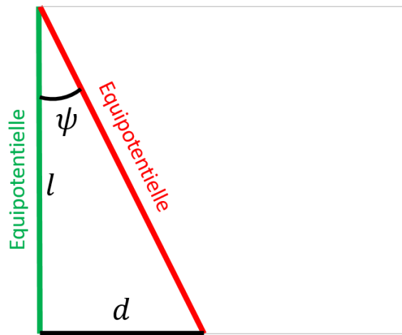
Figure 15 Problème de raccordement entre les équipotentielles sur le bord du barreau et les équipotentielles prédites par le calcul analytique. Il apparaît une distance caractéristique qui dépend de l'angle de Hall \psi et de la largeur du barreau.
