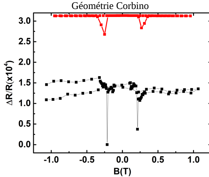
Figure 65 Magnétoconductance \frac{\Delta R}{R} comme définie au paragraphe précédent en fonction du champ magnétique appliqué
