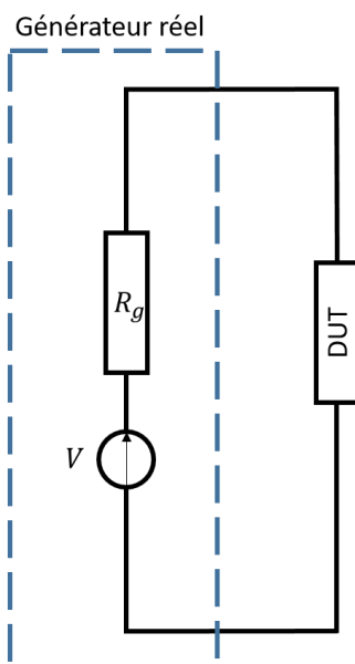
Figure 68 Schéma d'un générateur réel. V est la tension du générateur idéal, R_g la résistance interne et DUT est le dispositif (« Device Under Test »)
