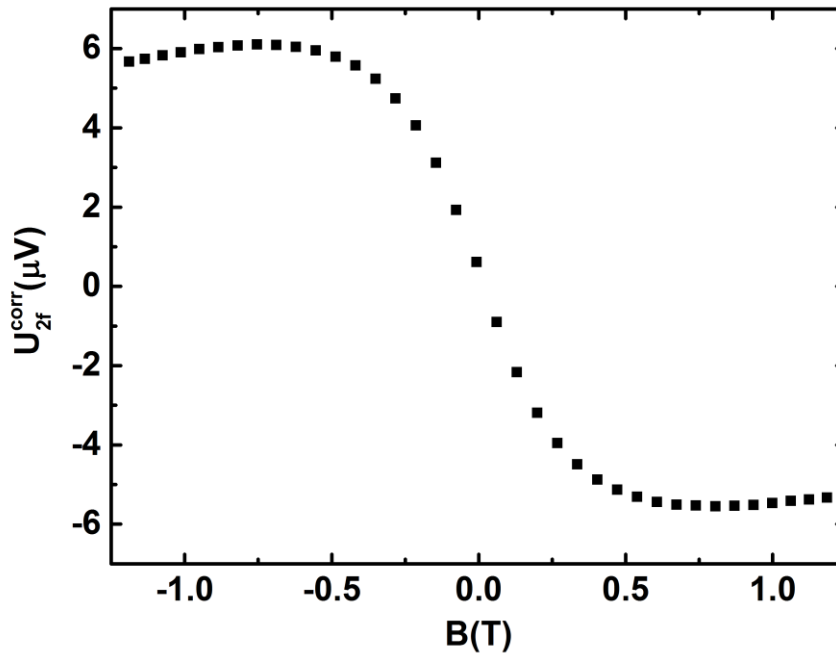
Figure 49 Mêmes données pour la tension à la fréquence 2f que dans la Figure 48 après correction et moyennage. Les données ont été translatées de telle sorte que la tension soit nulle à champ nul puis le signe de la tension a été changé pour les champs positifs.
