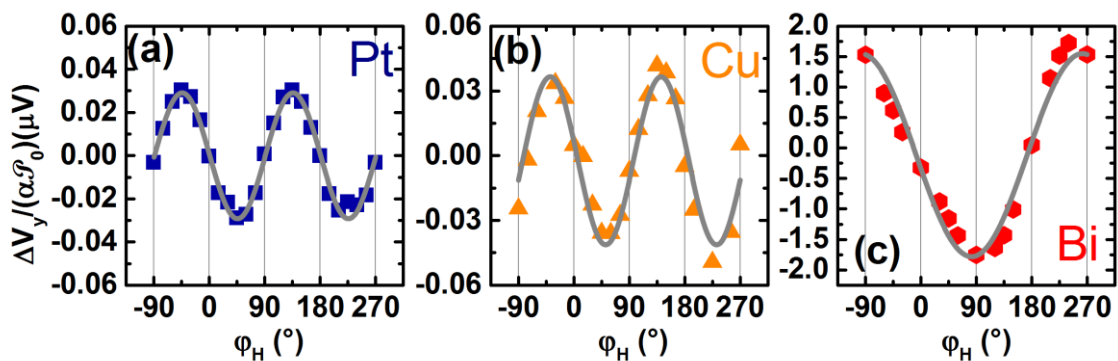
Figure 35 Comparatif de la tension mesurée sur l'électrode de (a) platine 50nm, (b) cuivre 20nm et (c) Bismuth 200nm en fonction de l'angle du champ magnétique pour un champ de 1T. Afin de rendre les amplitudes comparables, nous avons normalisé la tension mesurée par la puissance injectée et l'effet de court-circuit de l'électrode (Pham, 2014). La courbe gris foncé est un ajustement à \sin 2\varphi pour platine et cuivre et à \sin(\varphi_H) pour le bismuth
