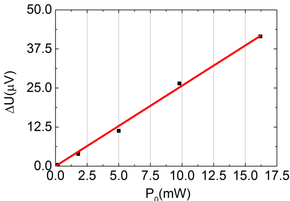
Figure 50 Amplitude du signal \Delta U = U_{2f}^{\text{corr}}(-1\text{T}) - U_{2f}^{\text{corr}}(1\text{T}) en fonction de la puissance injectée. Les carrés noirs sont les données expérimentales tandis que la ligne rouge est un ajustement linéaire passant par 0.
