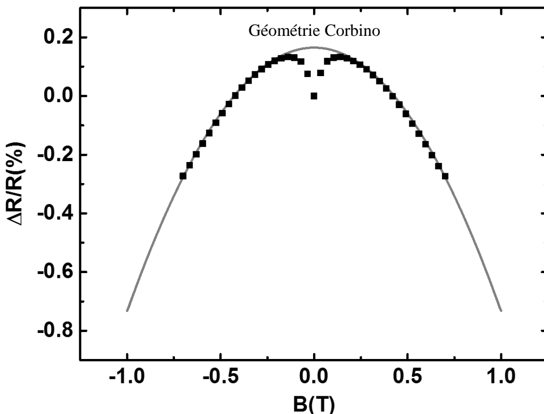
Figure 59 Magnétorésistance de Corbino \frac{\Delta R}{R} = \frac{R(B)-R(B=0)}{R(B=0)} , en fonction du champ magnétique appliqué en dehors du plan. Les carrés noirs sont les mesures expérimentales et la ligne grise a été obtenue à l'aide de la formule 171 ou m_z(B) a été obtenu par le programme Scilab de minimisation de l'énergie ferromagnétique en fonction du champ magnétique et le coefficient \Delta\rho/\rho_0 est la magnétorésistance anisotrope mesurée en géométrie barreau. La courbe obtenue a été translatée.
