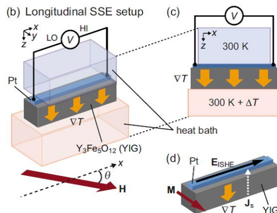
Figure 9 Reproduction de la Figure 1 (b) de (Uchida K., et al., 2010). Dans cette géométrie le courant de chaleur est attendu perpendiculaire à l'échantillon. Il n'y a plus la notion de tension qui change de signe entre les deux côtés de l'échantillon.
