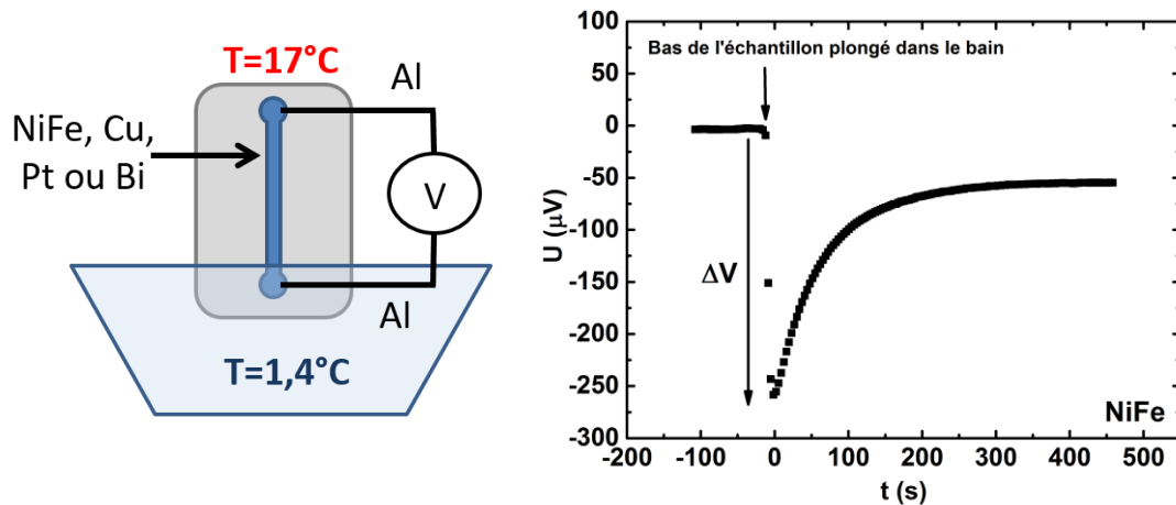
Figure 19 (gauche) Schéma de la mesure utilisée pour mesurer les coefficients Seebeck de nos couches minces. (droite) Mesure de la tension au cours du temps pour une lingette de permalloy. En t=0 le bas de l'échantillon est plongé dans le bain d'eau glacé. A cet instant la différence de température est égale à la différence entre la température du bain et la température extérieure donc \Delta T = 17 - 1,4 = 15,6\text{K} . Cette différence de température correspond à une différence de tension \Delta V représentée sur le graphique. Le coefficient Seebeck est alors : S = \Delta V / \Delta T . Dans le cas présent, le coefficient est négatif.
