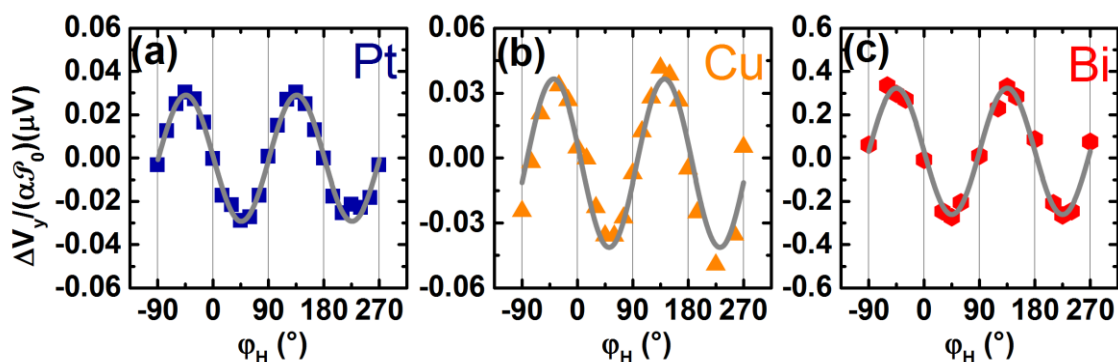
Figure 37 Comparatif de la tension mesurée sur l'électrode de (a) platine 50nm, (b) cuivre 20nm et (c) Bismuth 200nm en fonction de l'angle du champ magnétique pour un champ de 1T, corrigé de l'effet Nernst normal de l'électrode de bismuth causée par un défaut d'alignement. Afin de rendre les amplitudes comparables, nous avons normalisé la tension mesurée par la puissance injectée et l'effet de court-circuit de l'électrode (Pham, 2014) La courbe gris foncé est un ajustement à \sin 2\phi pour platine, le cuivre et le bismuth.
