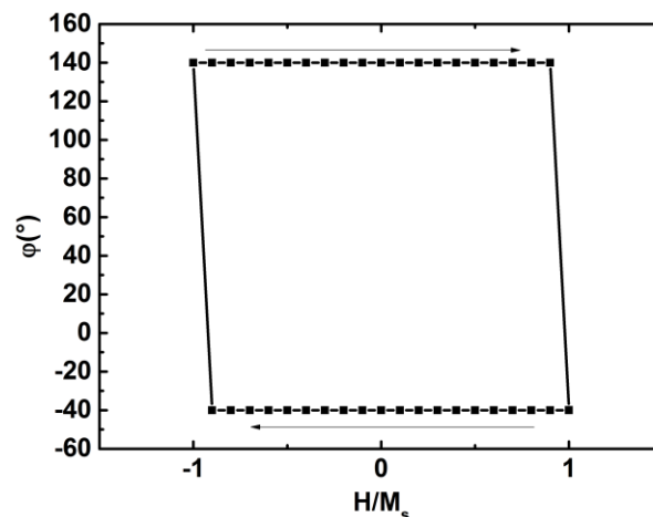
Figure 12 Angle de l'aimantation \varphi en fonction du champ magnétique appliqué normalisé par M_s . On observe que la composante dans le plan (xy) de l'aimantation lorsque l'aimantation n'est pas encore hors du plan est le long de l'axe d'anisotropie uniaxiale. Lorsque H est supérieur à M_s alors l'angle \varphi n'est plus défini puisque la projection de l'aimantation sur le plan (xy) est nulle.
