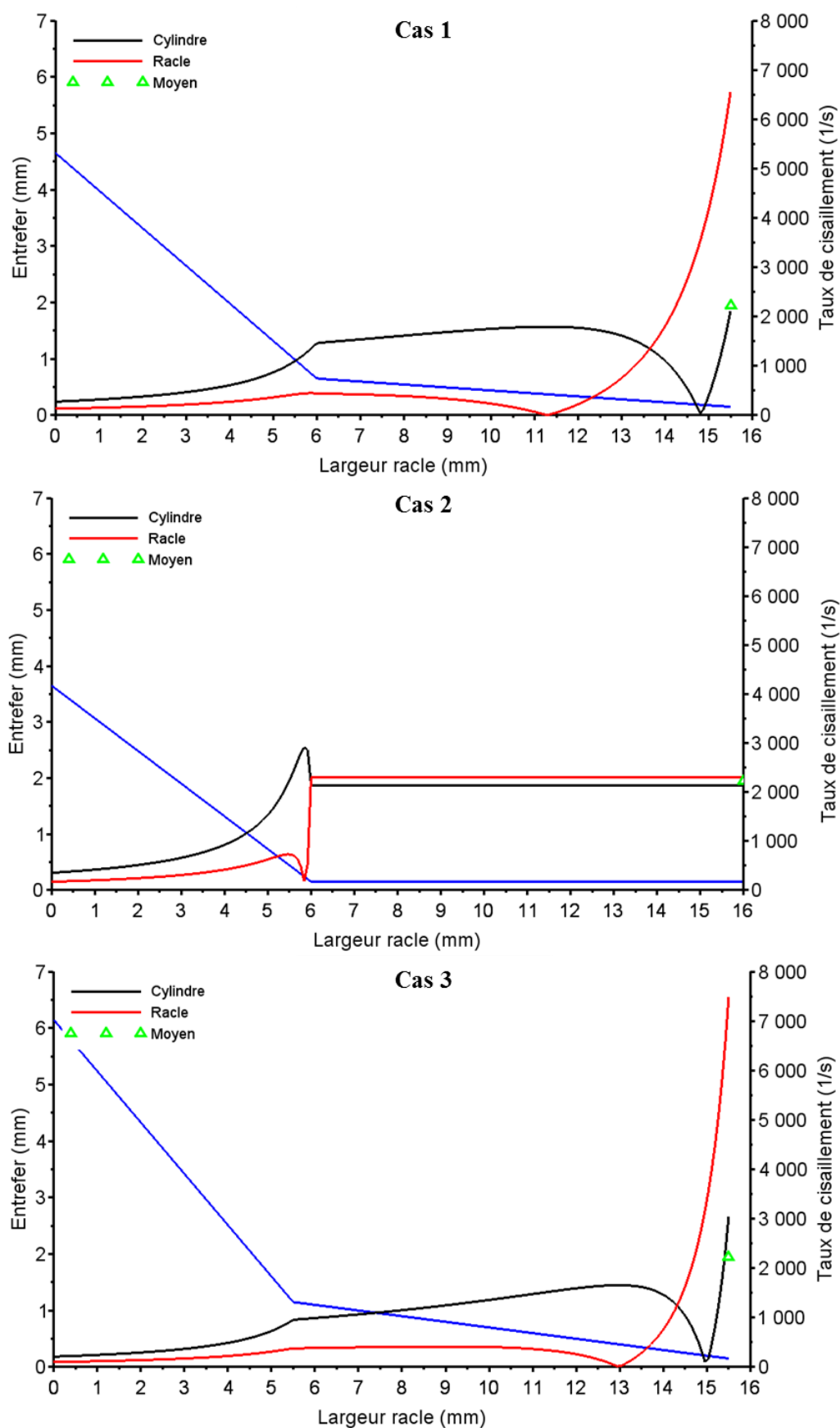
Figure 87 : Variation du taux de cisaillement au contact du cylindre (noir) et de la racle (rouge), et taux de cisaillement moyen pour les 3 cas (angle 15, 11 et 19°) à 20 m/min
