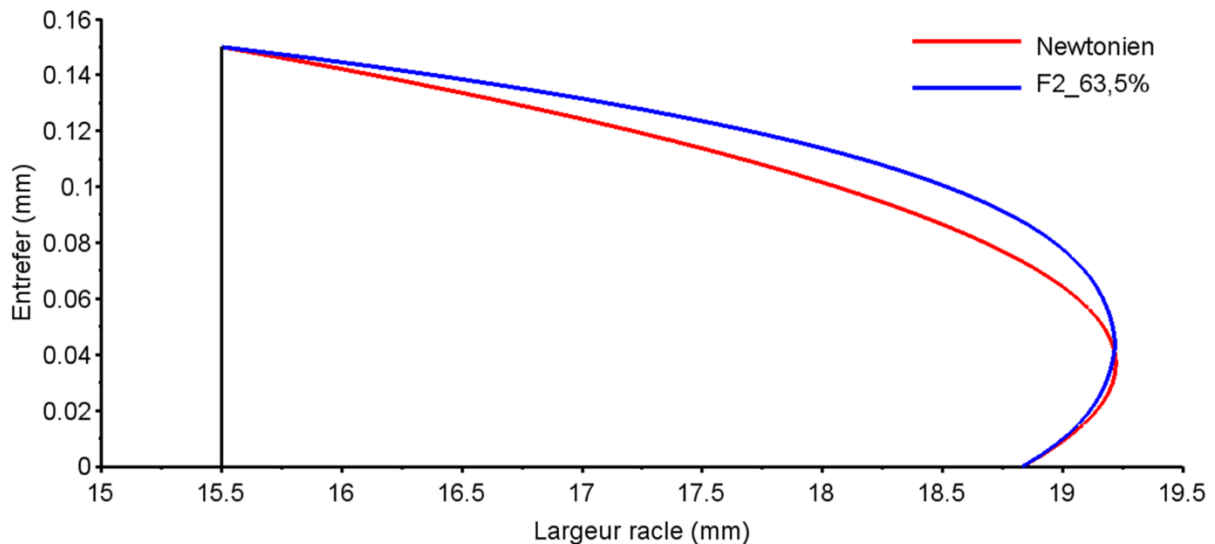
Figure 90 : Champ de vitesse en sortie de racle, comparaison entre le cas Newtonien et le cas réel (F2 à \phi=63,5\% ) : vitesse 20 m/min, entrefer final 0,15 mm, angle de la racle 15°
