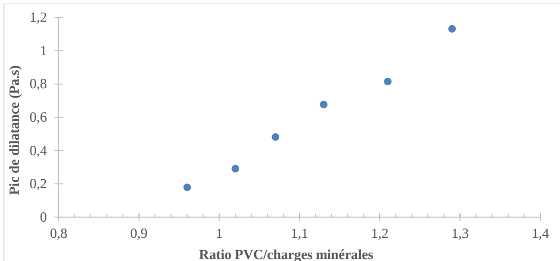
Figure 61 : Évolution du pic de dilatanse en fonction du ratio entre les particules PVC et les charges minérales pour la formulation F2D40 à \phi=64\%
