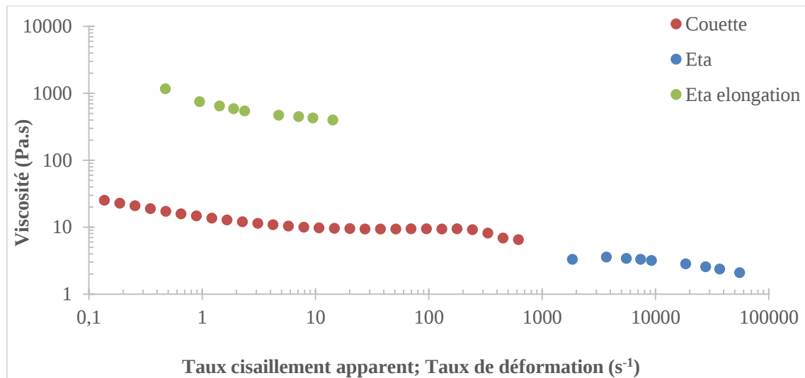
Figure 65 : Mesures rhéologiques au rhéomètre de Couette et au rhéomètre capillaire D=0,50 mm et la viscosité élongationnelle déduite des mesures capillaires pour F2D40 à \phi=64\%
