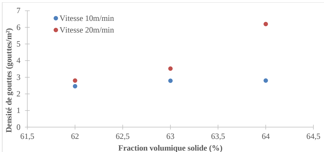
Figure 114 : Influence de la fraction volumique solide de F2D10 pour 2 vitesses d'enduction et une épaisseur déposée de 0,10 mm
