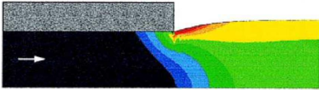
Figure 144 : Carte des contraintes tangentielles en sortie de capillaire :valeurs allant de -0,2 à 0,15 MPa en passant du bleu au rouge, la valeur 0 est entre le vert et le jaune (Venet et Vergnes 2000)
