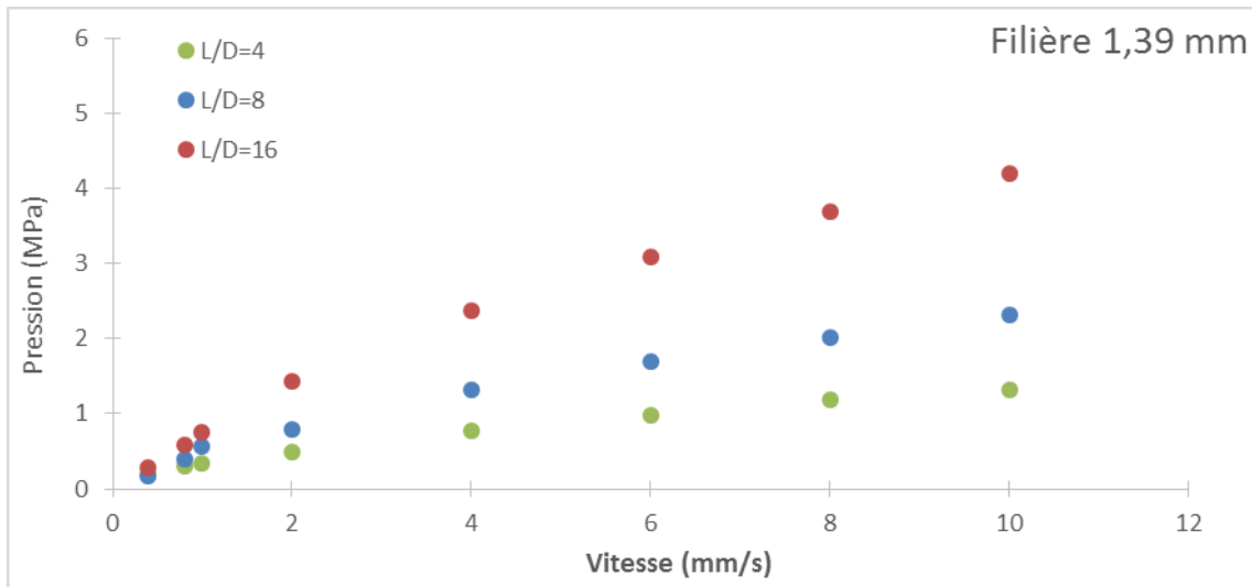
Figure A. 6 : Mesures de pressions à différentes vitesses pour le capillaire de diamètre 1,39 mm à différents ratio L/D pour F2
