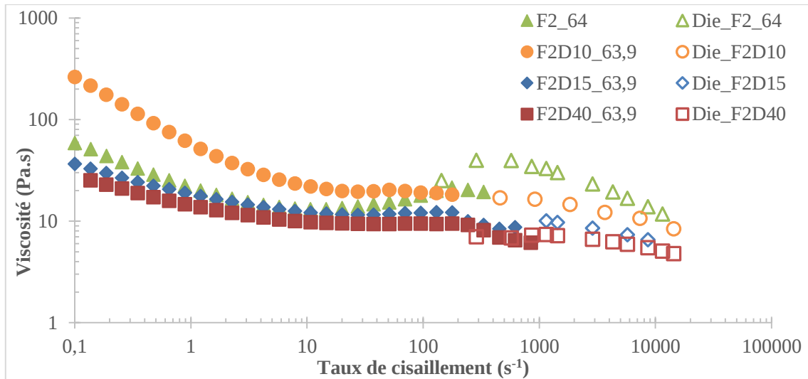
Figure 56 : Mesures rhéologiques au rhéomètre de Couette (symboles pleins) et au rhéomètre capillaire D=0,93 mm (symboles vides) pour la formulation de plastisol F2 et les formulations avec substitution de particules de PVC par des particules de \text{CaCO}_3 de taille variable
