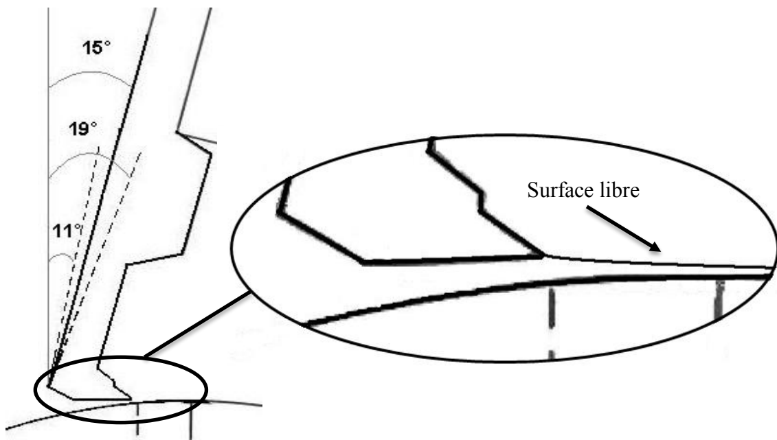
Figure 84 : Description de la position de la racle par rapport au cylindre
