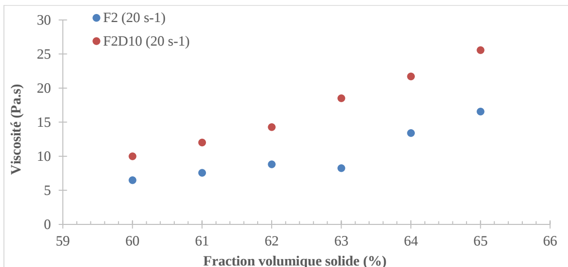
Figure 58 : Évolution comparée de la viscosité des formulations F2 et F2D10 à 20 \text{ s}^{-1}
