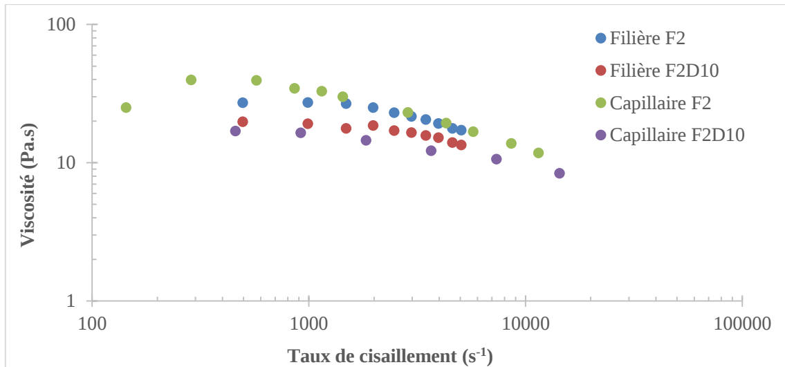
Figure 134 : Viscosité déduite des tests à la filière plate et en rhéométrie capillaire pour les formulations F2 et F2D10 à \phi=64\%
