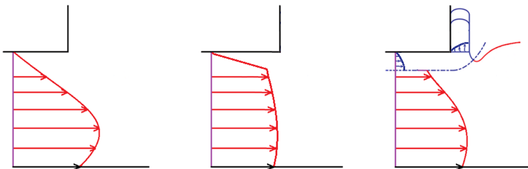
Figure 141 : Passage d'un écoulement d'un écoulement de coextrusion à la création d'un dépôt
