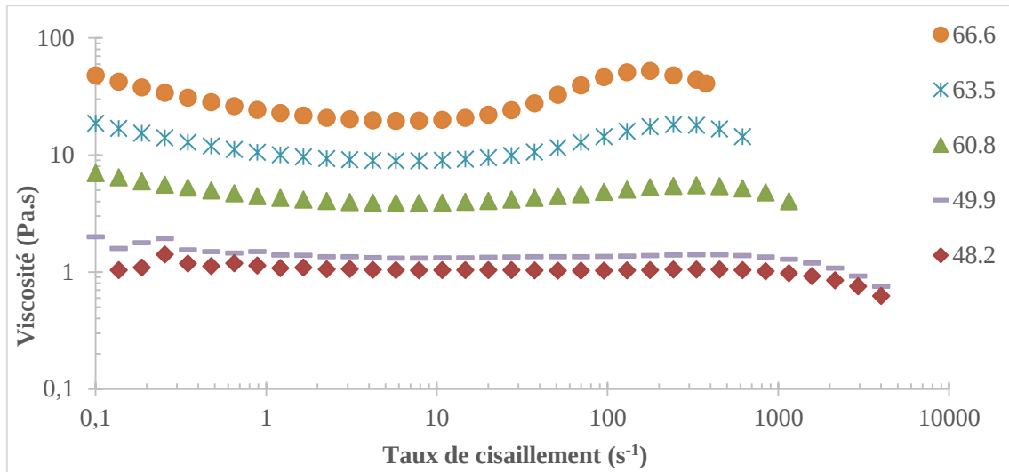
Figure 50 : Évolution de la rhéologie des formulations bimodales F2 en fonction du taux de particules
