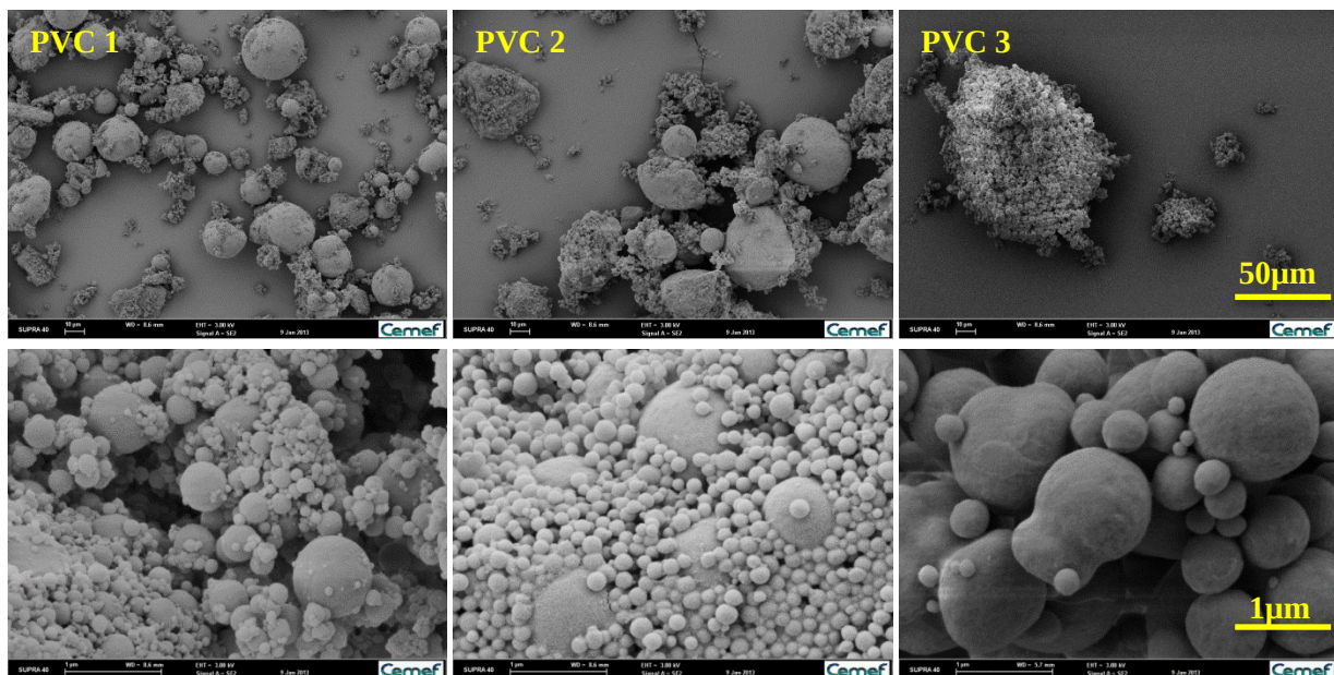
Figure 27 : Micrographies MEB à deux échelles différentes des 3 résines de PVC utilisées
