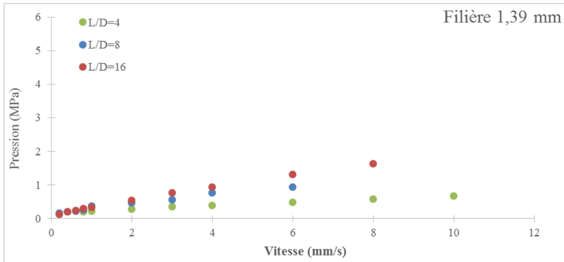
Figure A. 11 : Mesures de pressions à différentes vitesses pour le capillaire de diamètre 1,39 mm à différents ratio L/D pour F2D40
