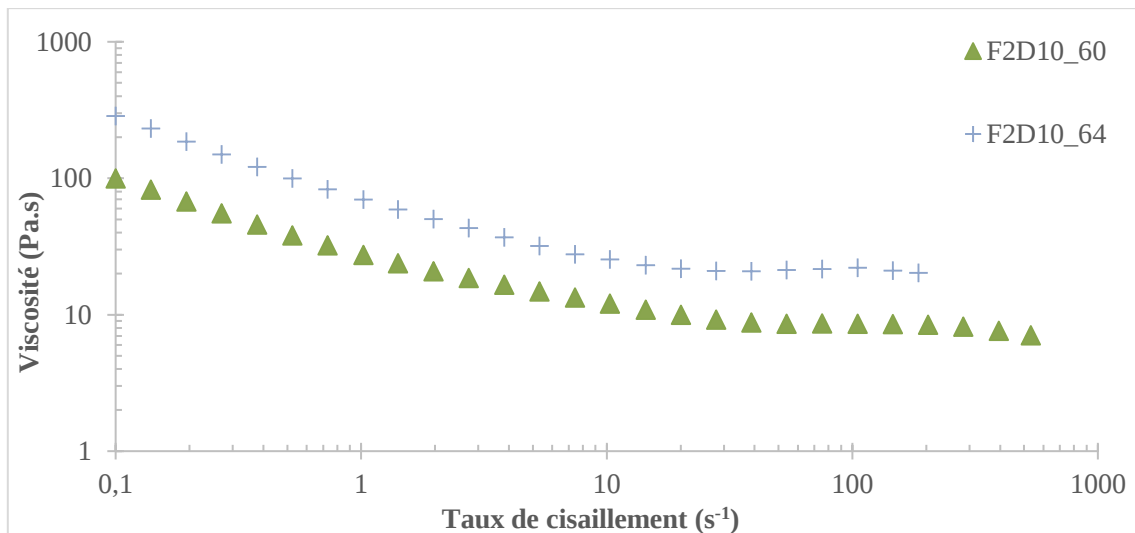
Figure 107 : Viscosité de F2D10 à \phi=60 et 64%
