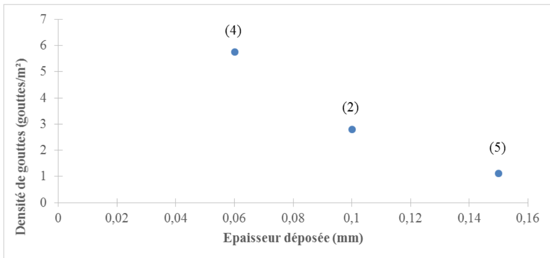
Figure 109 : Influence de l'épaisseur déposée sur F2D10 à \phi=63\% pour une vitesse de ligne de 10 m/min
