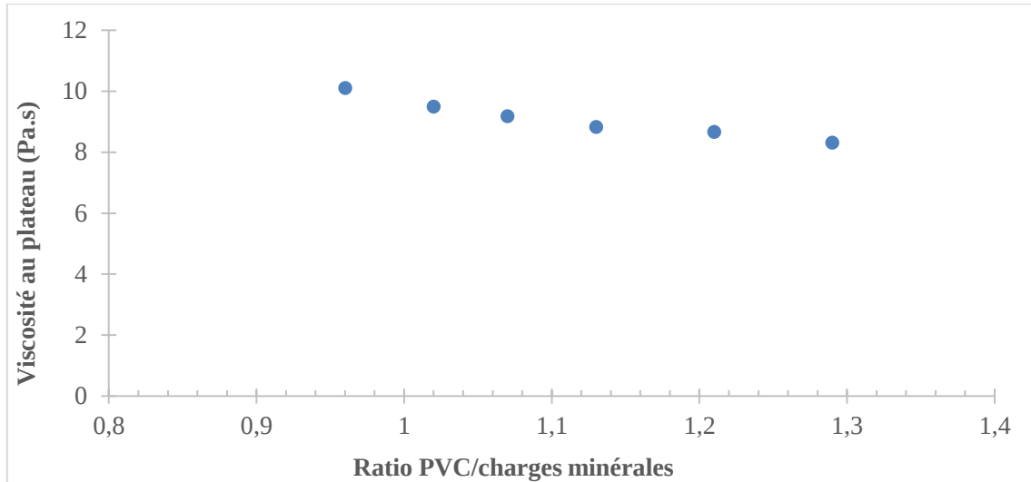
Figure 62 : Évolution de la viscosité au plateau Newtonien en fonction de la distribution de particules de PVC et de charges minérales pour la formulation F2D40 à \phi=64\%
