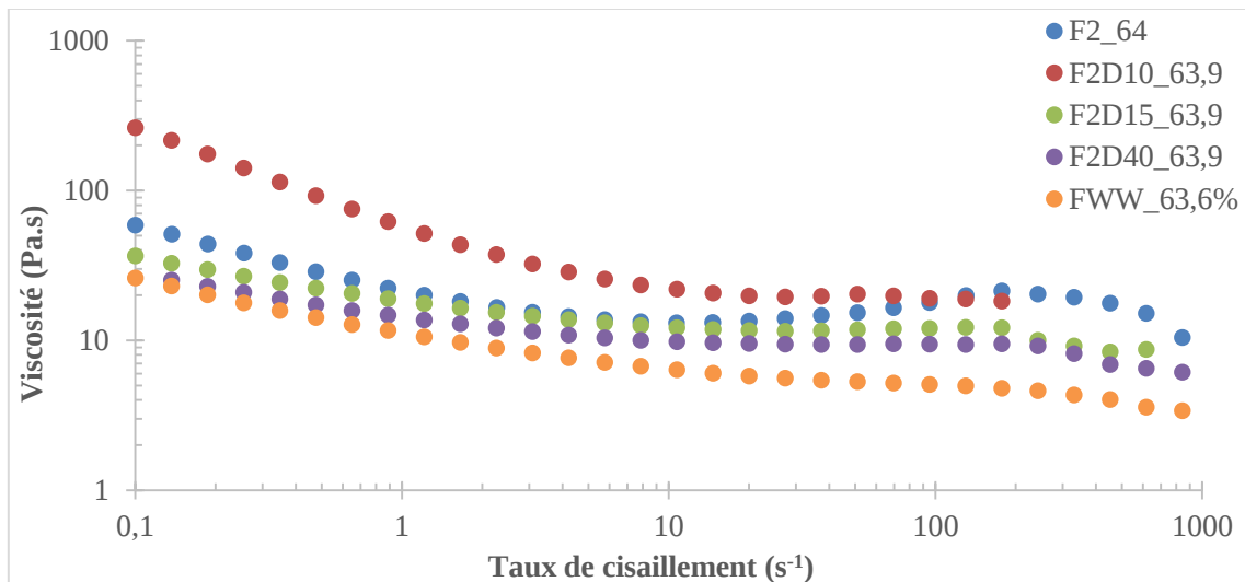
Figure 67 : Comparaison des mesures rhéologiques de la formulation industrielle FWW à \phi=63,6\% et des formulations modèles sans charge (F2 à \phi=64\% ) et avec charge (F2D10, F2D15 et F2D40 à \phi=63,9\% )
