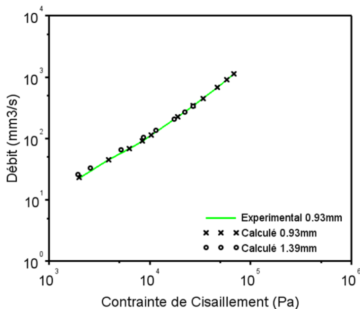
Figure 78 : Courbe d'écoulement expérimentale obtenue en capillaire pour un diamètre 0,93 mm comparée à la courbe des débits calculés à partir de la rhéologie capillaire pour un diamètre 0,93 mm et 1,39 mm, pour F2D40 à \phi=63,9\%
