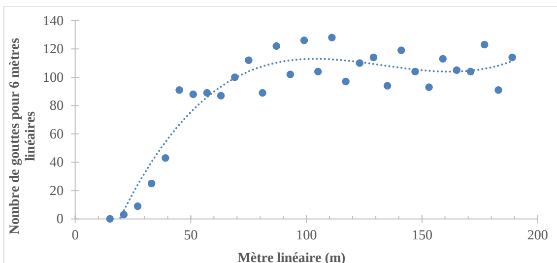
Figure 106 : Nombre de gouttes par mètre linéaire à 10 m/min pour FWW à \phi=63,6\%
