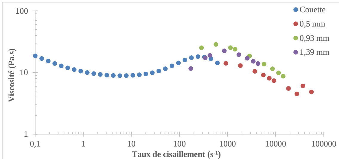
Figure 69 : Courbe de viscosité en rhéométrie Couette et en rhéométrie capillaire pour 3 diamètres (D=0,5 ; 0,93 et 1,39 mm) en fonction du taux de cisaillement pour la formulation F2 à \phi=63,5\%
