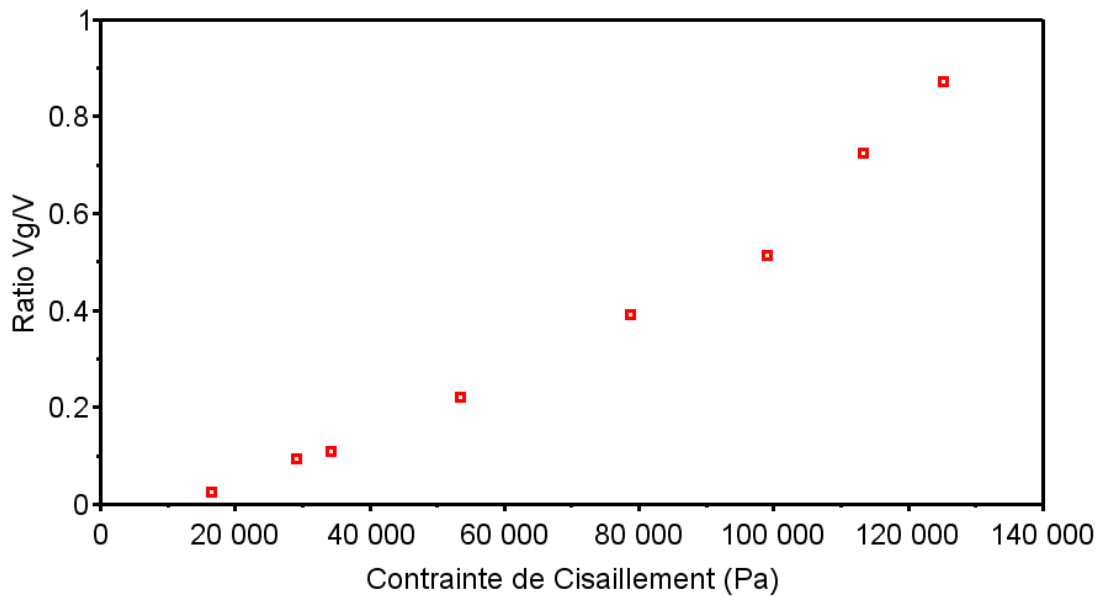
Figure 75 : Ratio de la vitesse de glissement (diamètre 0,50 mm) sur la vitesse moyenne en fonction de la contrainte de cisaillement pour F2 à \phi=63,5\%
