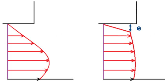
Figure 138 : Passage d'un écoulement pour un plastisol homogène à un écoulement de coextrusion
