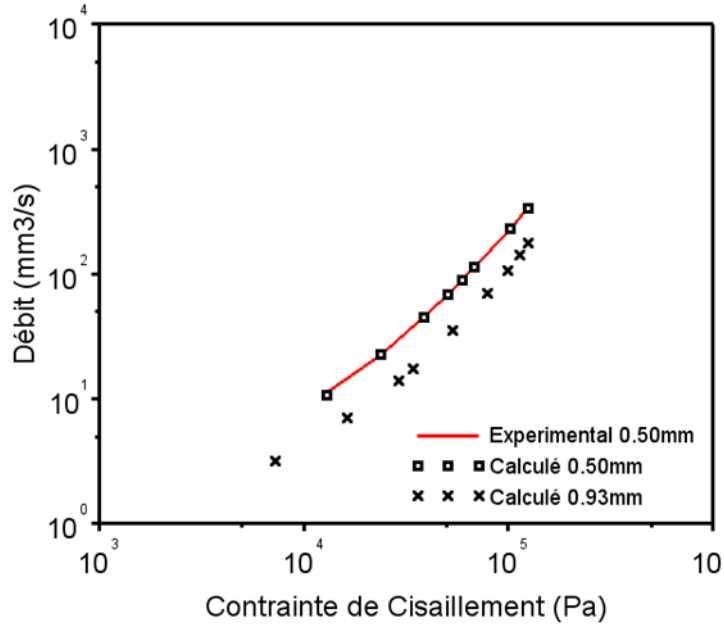
Figure 73 : Courbe d'écoulement expérimentale obtenue en capillaire pour un diamètre 0,50 mm comparée à la courbe des débits calculés à partir de la rhéologie capillaire pour un diamètre 0,50 mm et 0,93 mm, pour F2 à \phi=63,5\% ,
