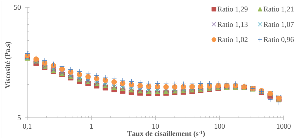
Figure 60 : Influence du ratio PVC/charge pour la formulation F2D40 à \phi=64\%
