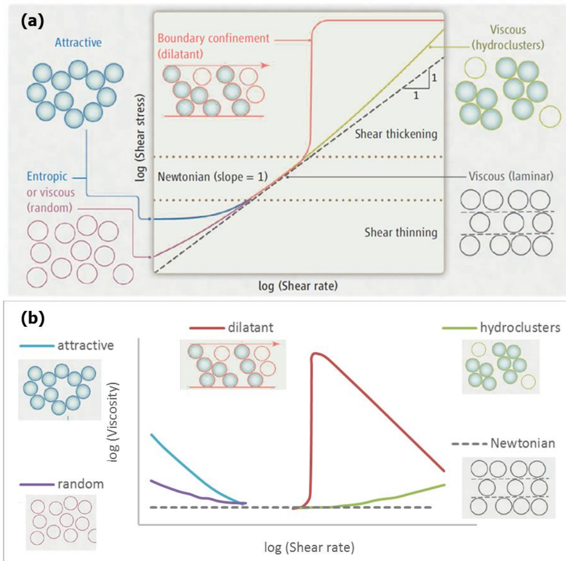
Figure 23 : Approche synthétique du comportement des suspensions, (a) : d'après Brown et Jaeger (2011) et (b) : retranscription exprimant la viscosité en fonction du taux de cisaillement
