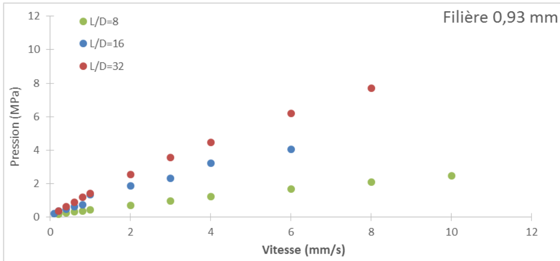
Figure A. 10 : Mesures de pressions à différentes vitesses pour le capillaire de diamètre 0,93 mm à différents ratio L/D pour F2D40
