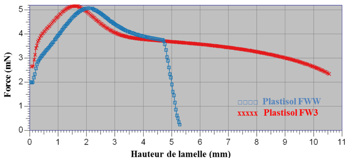
Figure 147 : Test d'extraction de lamelle pour la formulation avec charge FWW ou sans charge FW3
