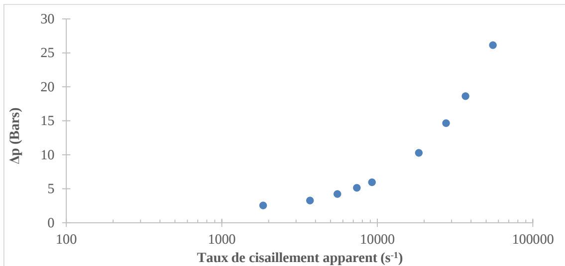
Figure 64 : Corrections de pression d'entrée en fonction du taux de cisaillement aval, avec le capillaire D=0,50 \text{ mm} pour F2D40 à \phi=64\%
