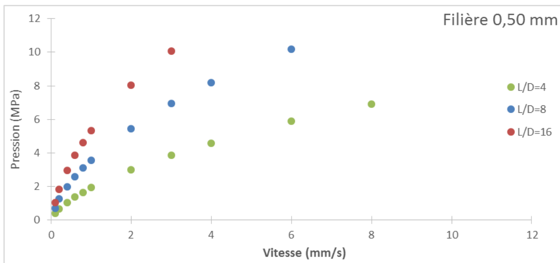
Figure A. 4 : Mesures de pressions à différentes vitesses pour le capillaire de diamètre 0,50 mm à différents ratio L/D pour F2
