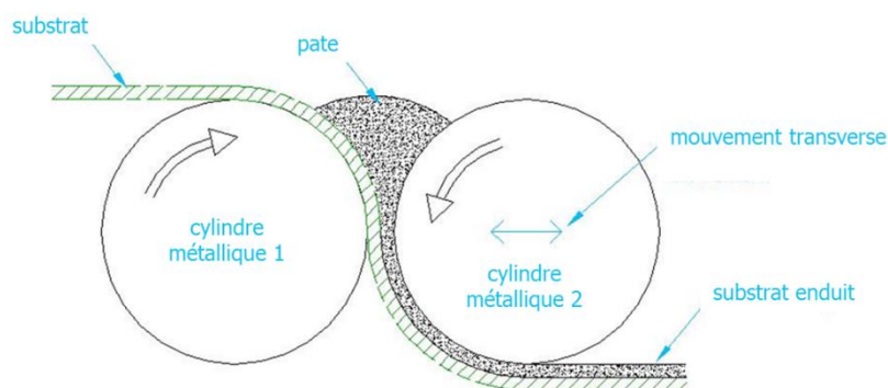
Figure 8 : Procédé d'enduction calandrage
