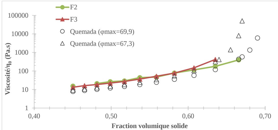
Figure 52 : Évolution de la viscosité au palier Newtonien en fonction de la fraction volumique solide pour les formulations F2 et F3 mesurées à 4,2 s -1 . Comparaison au modèle de Quemada pour deux valeurs de \phi_{max}
