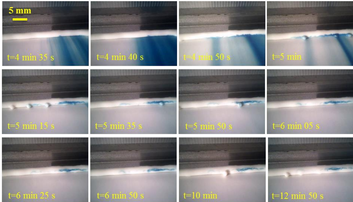
Figure 105 : Observation de la vitesse de montée du dépôt en aval de la racle pour la formulation FWW à \phi=63,6\% pour une vitesse de 10 m/min et une épaisseur déposée de 0,10 mm
