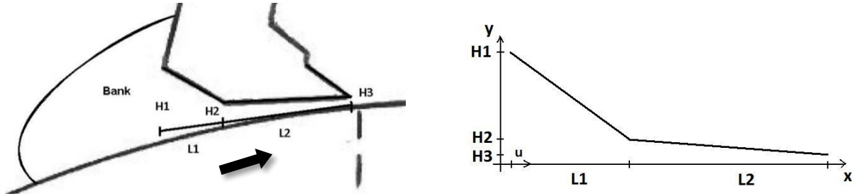
Figure 82 : (a) : Géométrie de la racle ; (b) : Géométrie équivalente dans un repère (x,y)
