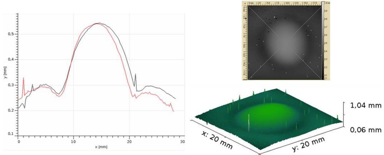
Figure 103 : Mesure au rugosimètre optique d'une goutte prégélifiée
