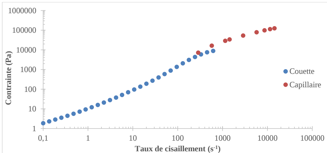
Figure 68 : Courbe de contrainte en rhéométrie Couette et en rhéométrie capillaire ( D=0,93\text{mm} ) en fonction du taux de cisaillement pour la formulation F2 à \phi=63,5\%
