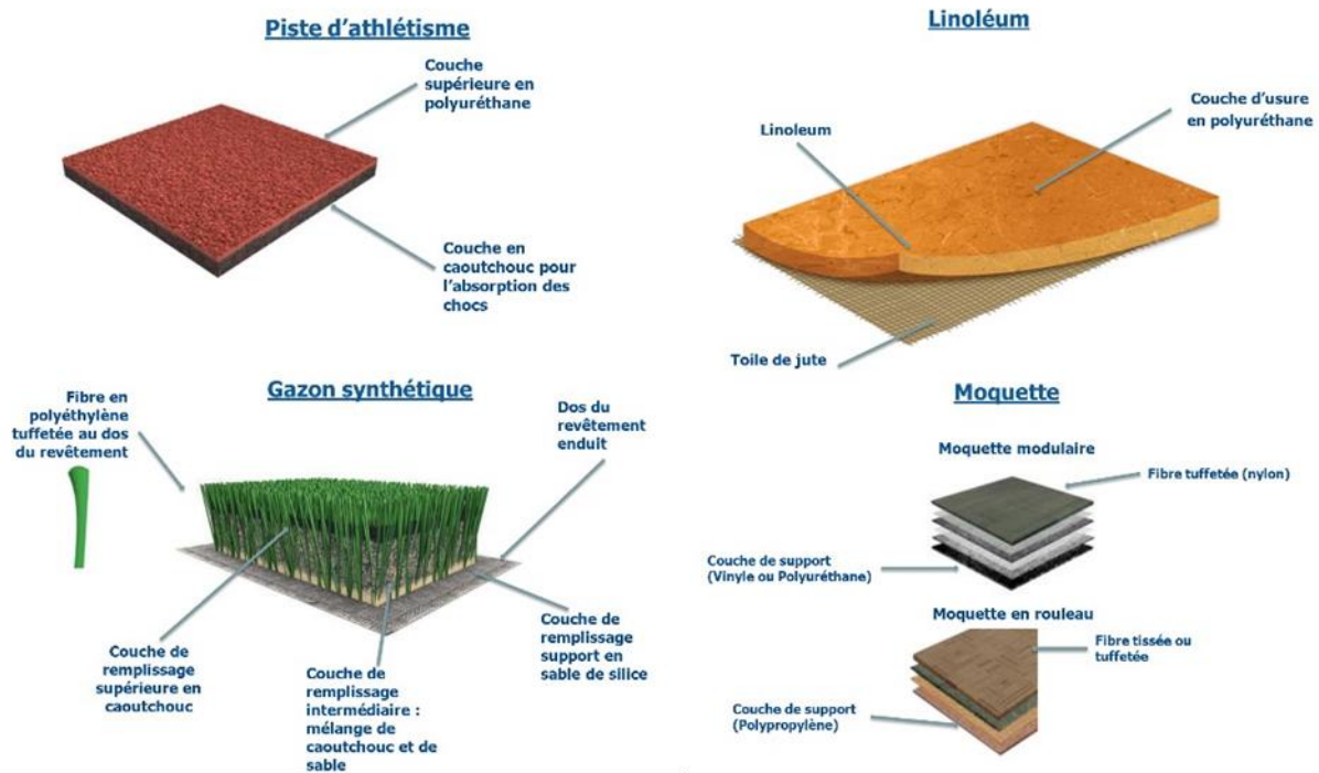
Figure 3 : Composition des revêtements piste d'athlétisme, linoléum, gazon synthétique et moquette
