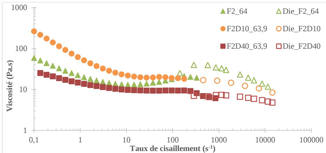
Figure 98 : Courbe de viscosité en rhéométrie Couette et en rhéométrie capillaire pour le diamètre D=0,93 mm en fonction du taux de cisaillement pour les formulations F2 à \phi=64\% , F2D10 et F2D40 à \phi=63,9\%
