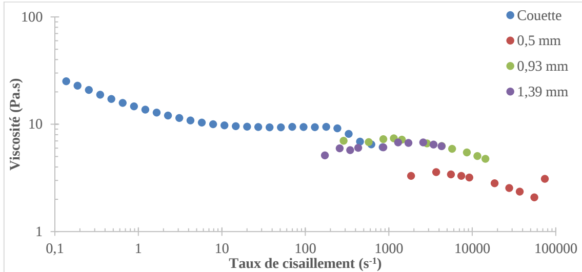
Figure 76 : Courbe de viscosité en rhéométrie Couette et en rhéométrie capillaire pour 3 diamètres ( D=0,5 ; 0,93 et 1,39 mm) en fonction du taux de cisaillement pour la formulation F2D40 à \phi=63,9\%
