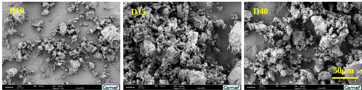
Figure 29: Micrographies MEB des trois charges CaCO 3 utilisées
