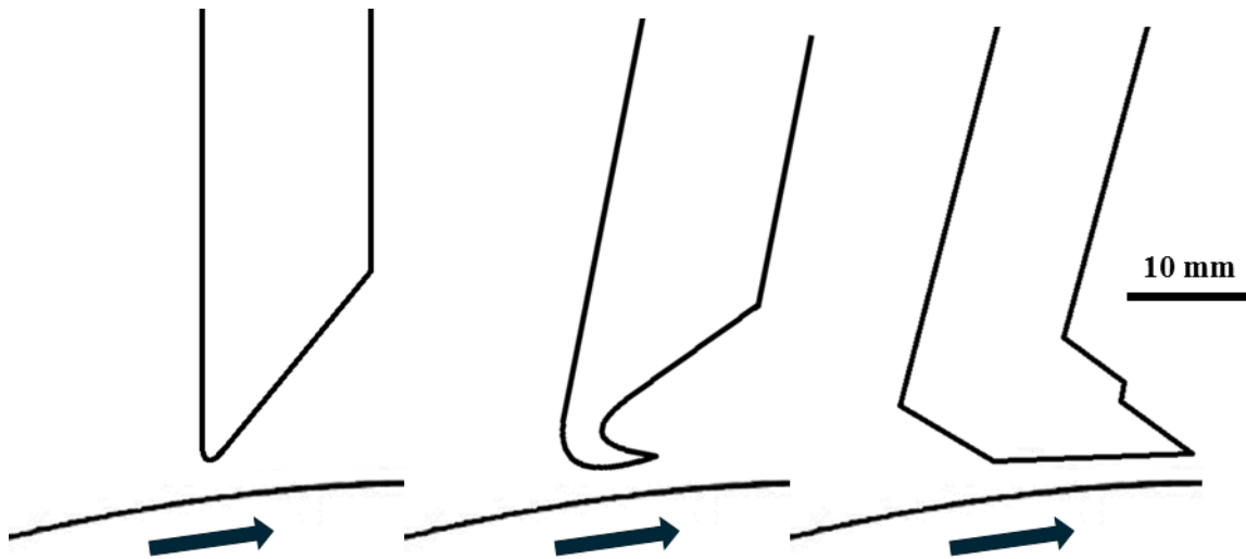
Figure 7 : Schéma de différentes géométries de racle : simple, à bec et à talon
