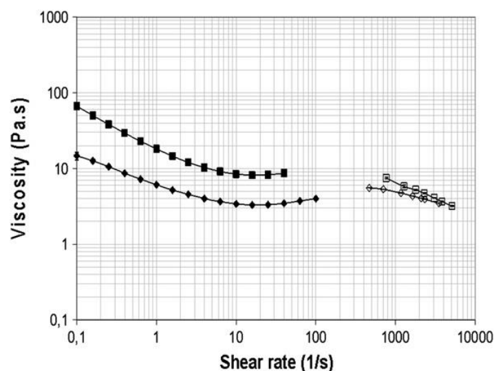
Figure 26 : Comparaison d'un plastisol contenant 30% (◆) et 10%(■) de grosses particules, (Barroso et al. 2010)
