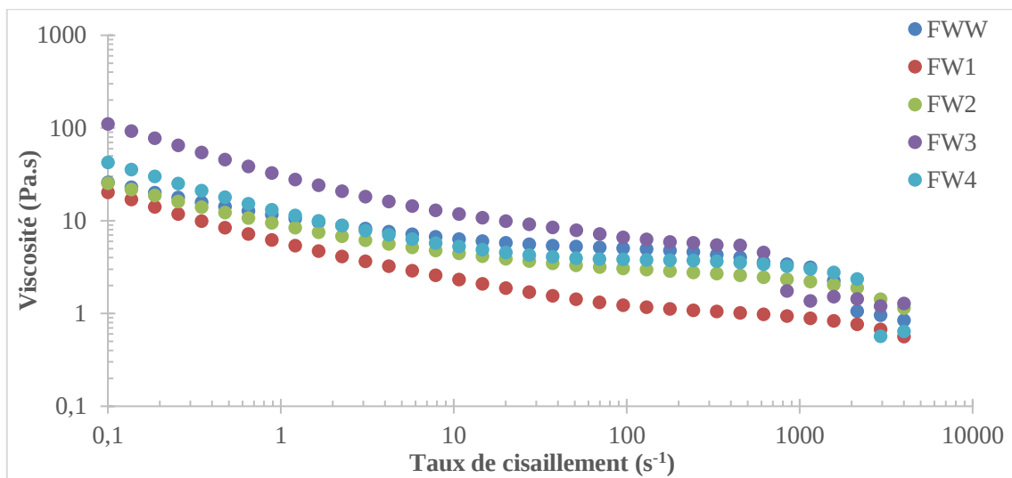
Figure 124 : Viscosité mesurée en rhéométrie Couette de FWW et ses dérivées
