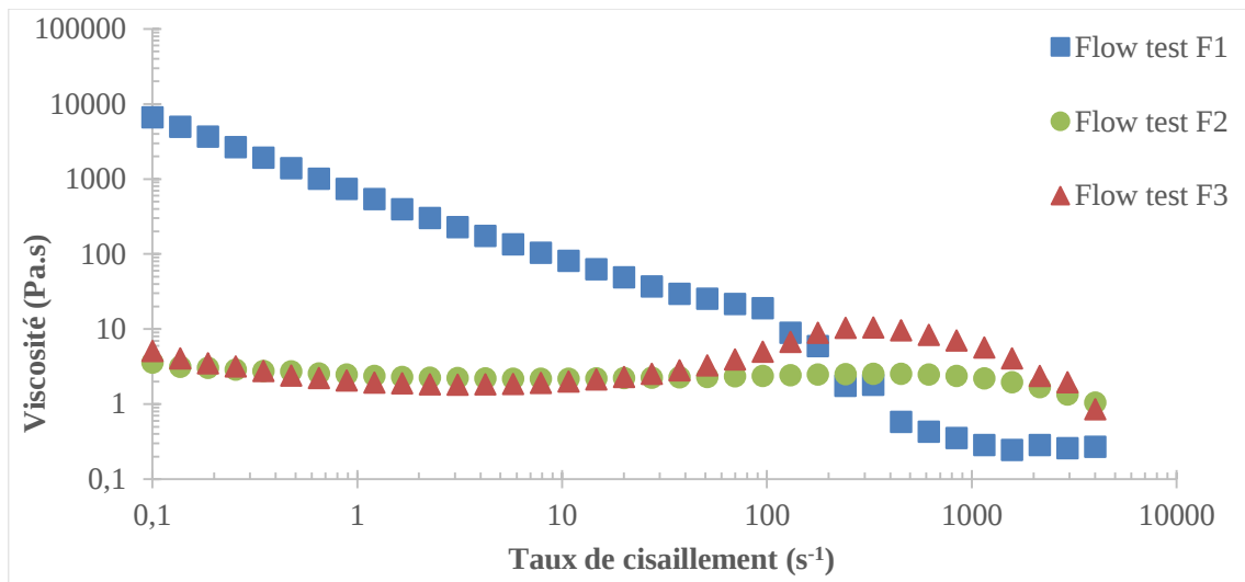
Figure 46 : Mesures de viscosité des trois formulations de plastisol avec des distributions de taille de particules différentes ( \phi=57,3\% ; rhéomètre de Couette)
