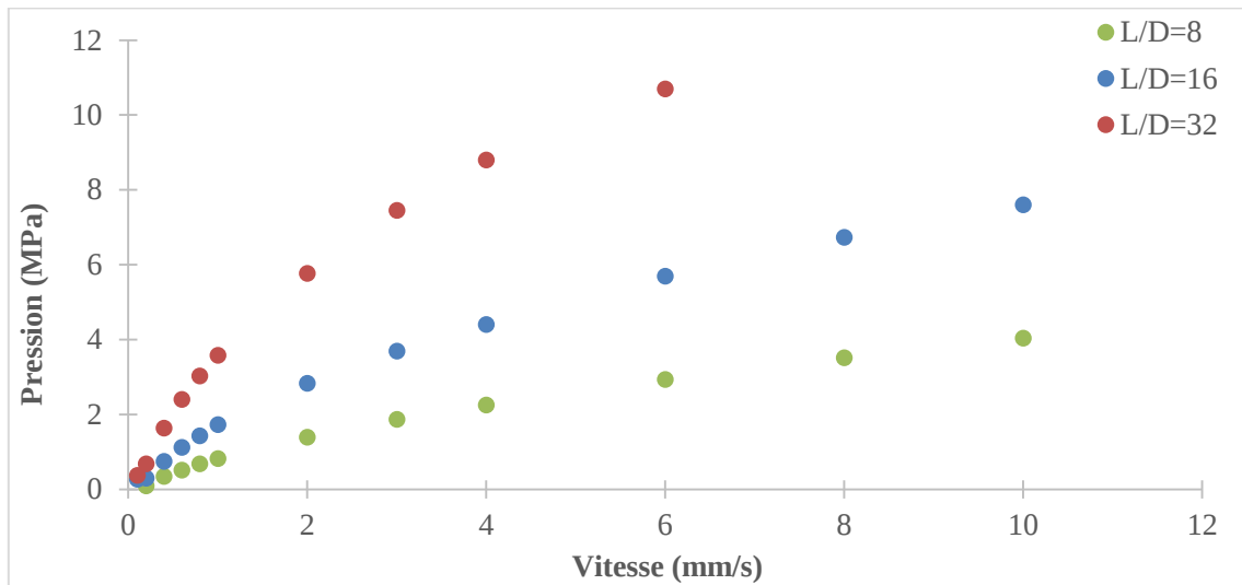
Figure 37 : Mesures de pressions à différentes vitesses pour le capillaire de diamètre 0,93 mm à différents ratio L/D pour F2 à \phi=63\% .
