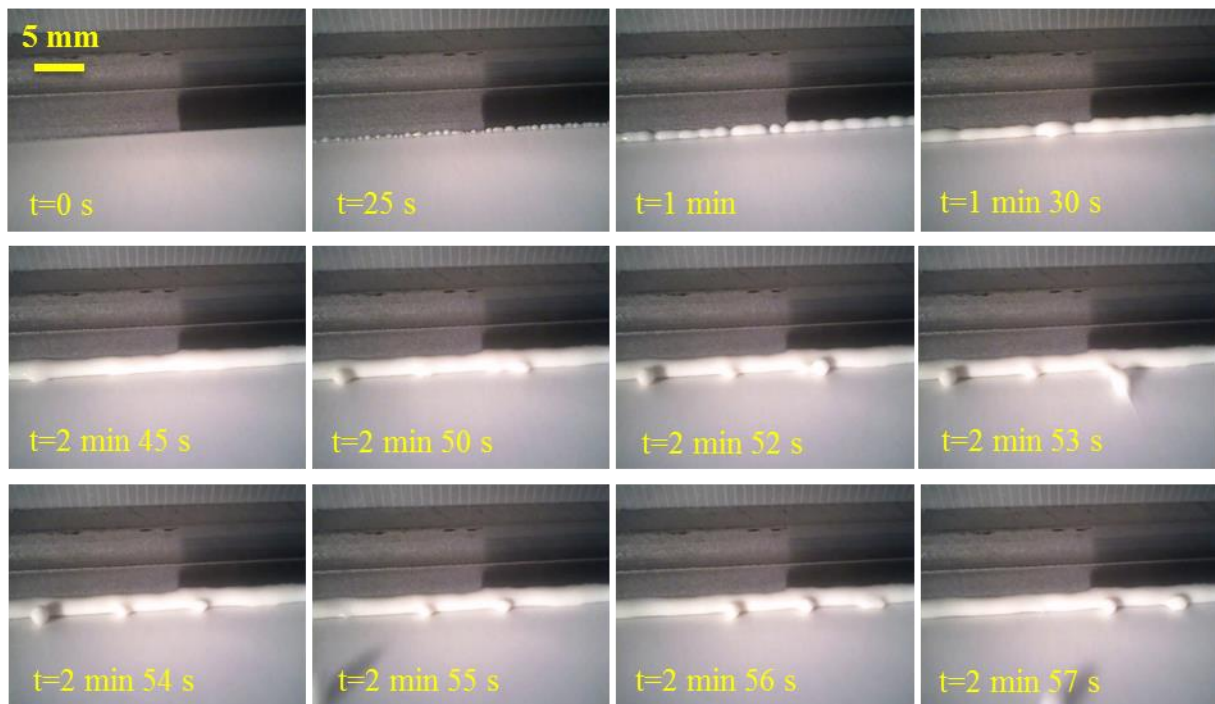
Figure 101 : Création du dépôt et de gouttes en aval de la racle pour la formulation FWW à \phi=63,6\% pour une vitesse de 10 m/min et une épaisseur déposée de 0,10 mm
