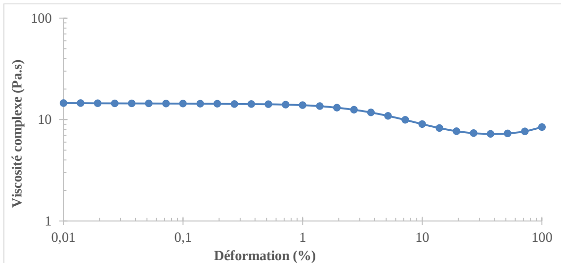
Figure 31 : Balayage en déformation à 10 \text{ rad/s} de F2 à \phi=63\%
