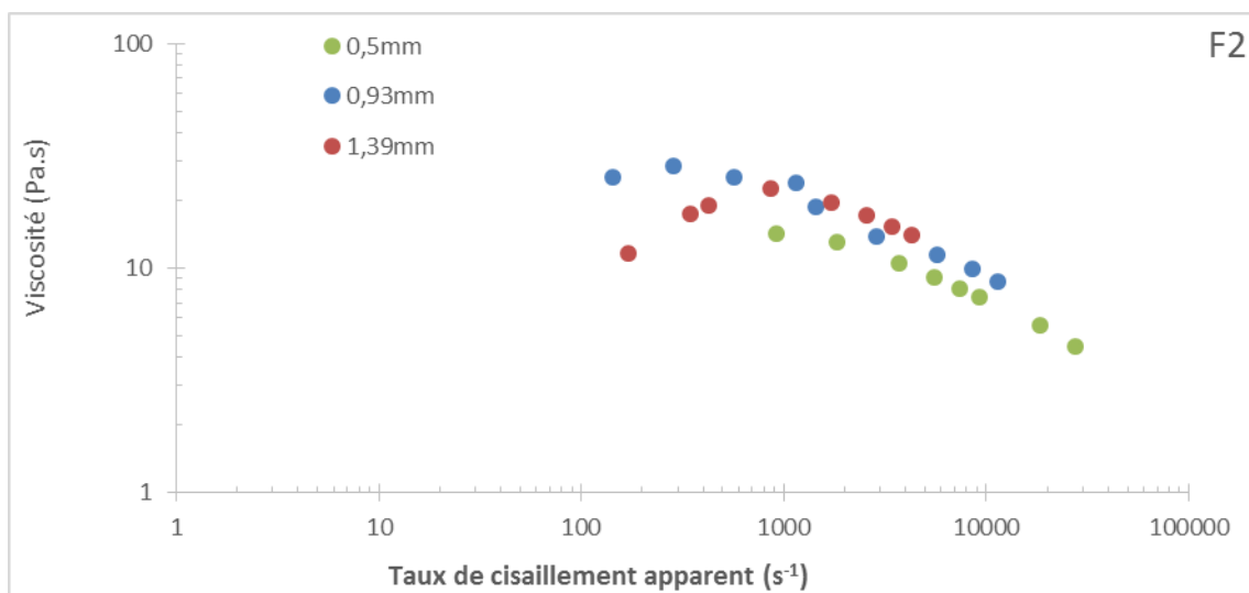
Figure A. 8 : Viscosité en fonction du taux de cisaillement pour F2
