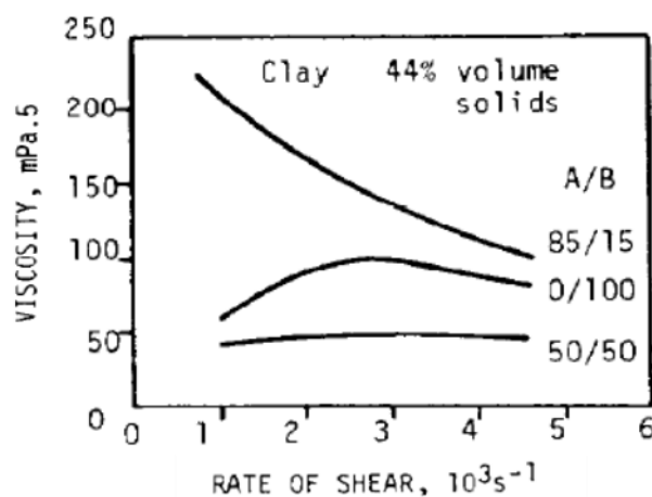
Figure 20 : Viscosité de mélanges de 2 charges monomodales de tailles différentes : A ( 9\mu\text{m} ) et B ( 0,7\mu\text{m} ), (Barnes 1989; Alince and Lepoutre 1983)
