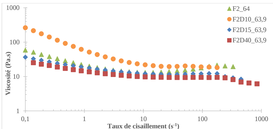
Figure 54 : Mesures rhéologiques pour les formulations F2, F2D10, F2D15 et F2D40 pour un taux de charge global \phi \approx 64\% (rhéologie Couette)
