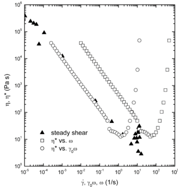
Figure 21 : Viscosité d'une solution de silice (60%) en fonction du taux de cisaillement
