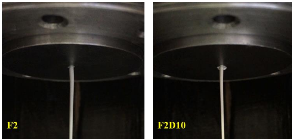
Figure 136 : Dépôt en sortie de filière plate pour les formulations F2 et F2D10 à \phi=63\% à 3000 \text{ s}^{-1}
