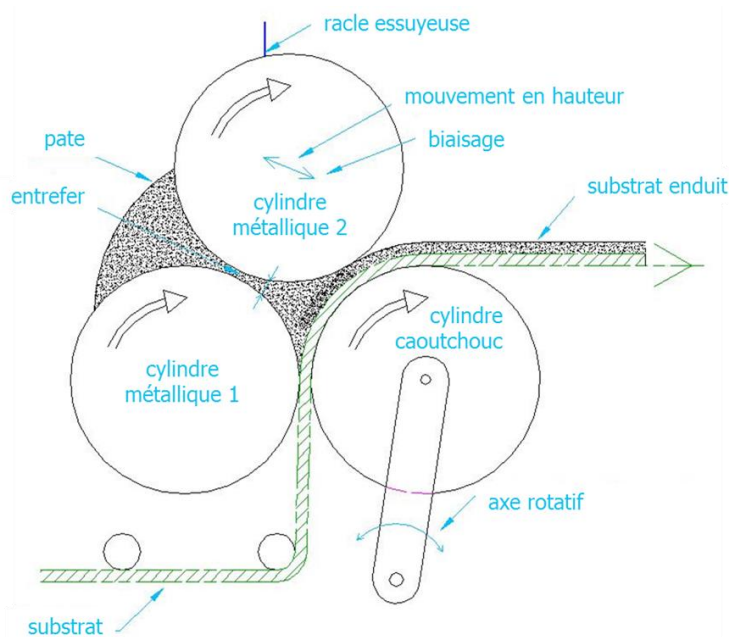
Figure 10 : Procédé d'enduction en « reverse roll »
