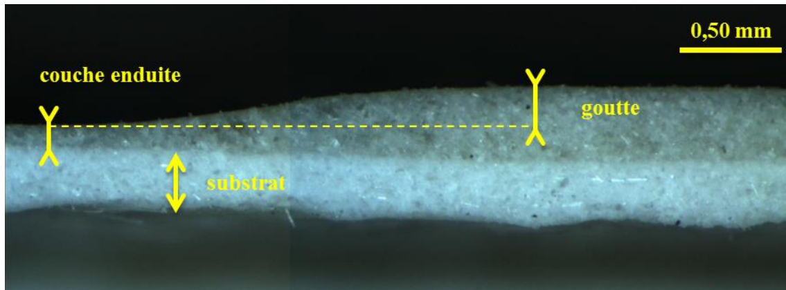
Figure 104 : Coupe du substrat, du plastisol déposé et d'une goutte pour la formulation FWW
