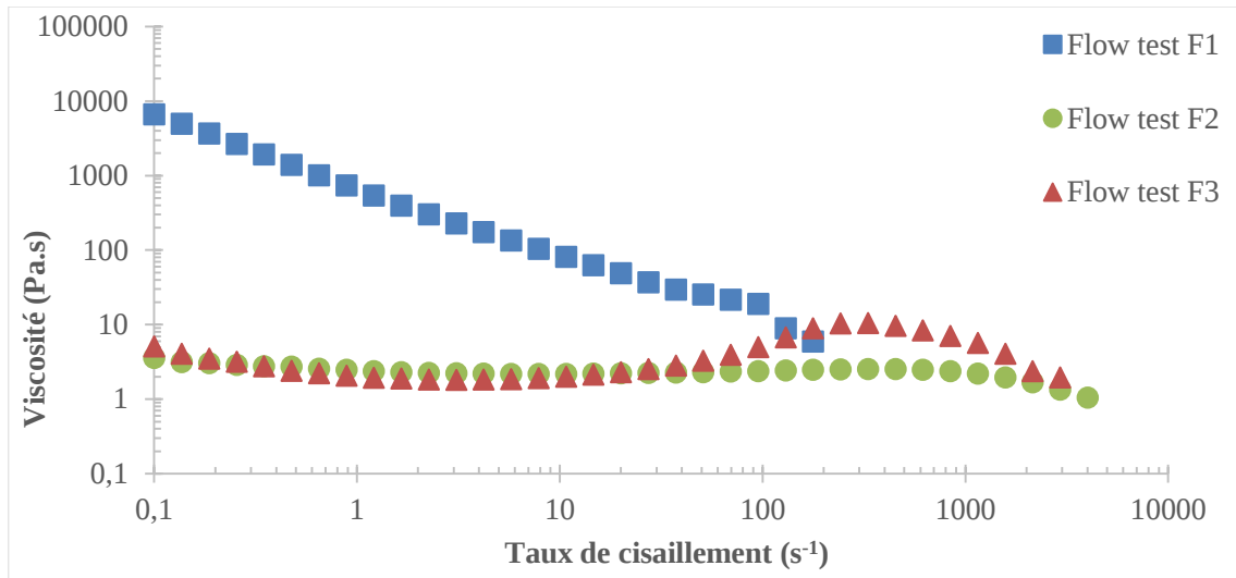
Figure 47 : Mesures de viscosité de F1, F2 et F3 à \phi=57,3\%
