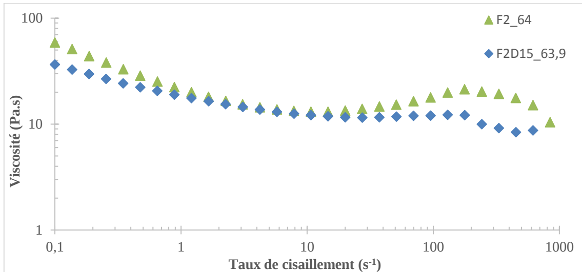
Figure 142 : Courbes de viscosité de différents plastisols donnant du dépôt (◆), ne donnant pas de dépôt (▲)
