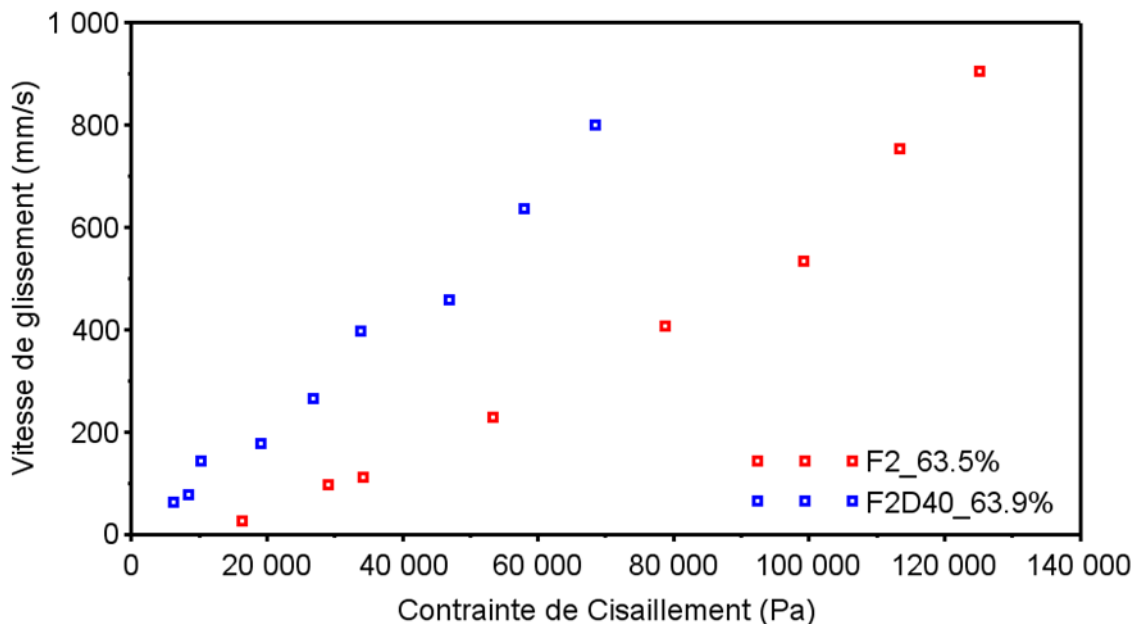
Figure 80 : Vitesse de glissement en fonction de la contrainte à la paroi pour F2 à \phi=63,5\% et F2D40 à \phi=63,9\%
