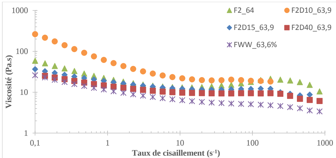
Figure 128 : Comparaison des rhéologies Couette des formulations modèles et de la formulation industrielle FWW
