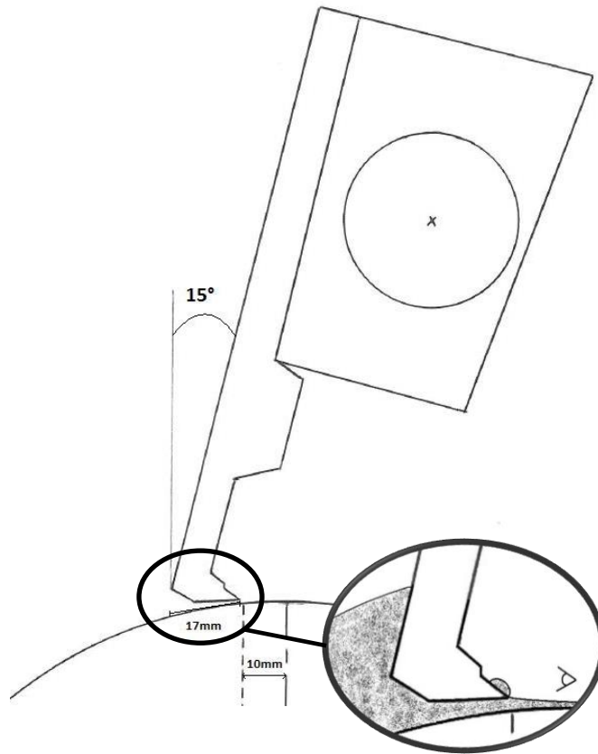
Figure 100 : Racle du pilote à Wiltz
