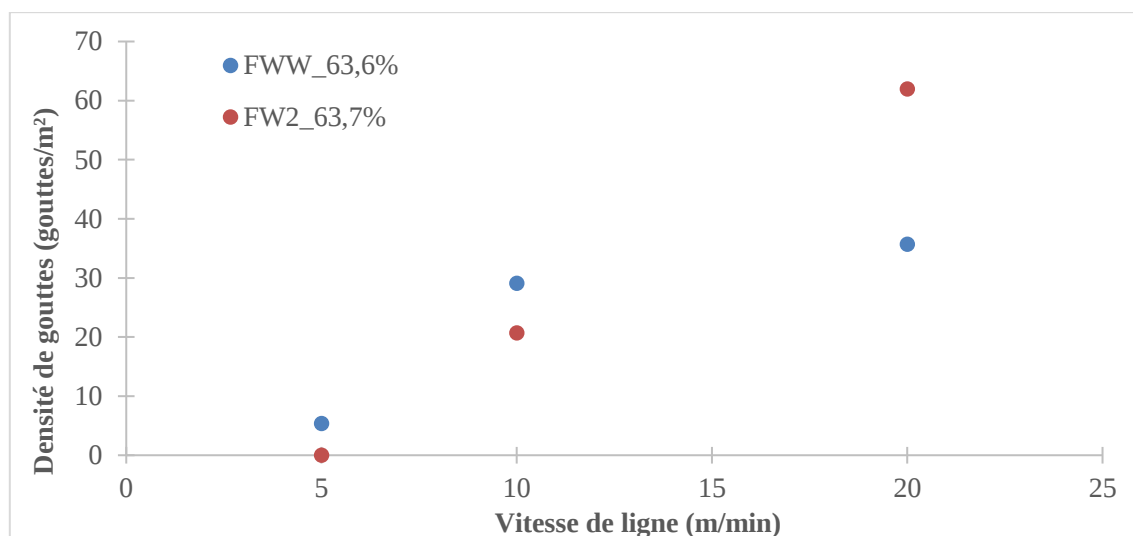
Figure 125 : Comparaison de la densité de gouttes d'une formulation avec (FWW) et sans (FW2) adjuvant en fonction de la vitesse de ligne pour une épaisseur déposée de 0,10 mm
