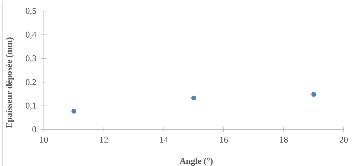
Figure 96 : Épaisseur déposée en fonction de l'angle de la racle pour F2 à \phi=63,5\%
