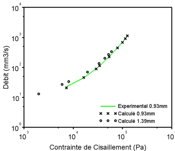
Figure 72 : Courbe d'écoulement expérimentale obtenue en capillaire pour un diamètre 0,93 mm comparée à la courbe des débits calculés à partir de la rhéologie capillaire pour un diamètre 0,93 mm et 1,39 mm, pour F2 à \phi=63,5\% ,
