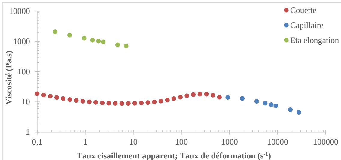
Figure 45 : Comparaison entre la viscosité élongationnelle de la Figure 44 et la viscosité en cisaillement (Couette et capillaire D=0,50 mm) pour F2 à \phi=63,5\%
