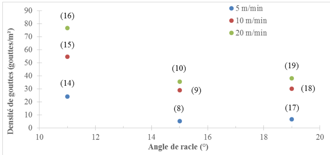
Figure 122 : Influence de l'angle de la racle sur FWW à \phi=63,6\% à 5, 10 et 20/min pour une épaisseur déposée de 0,10 mm
