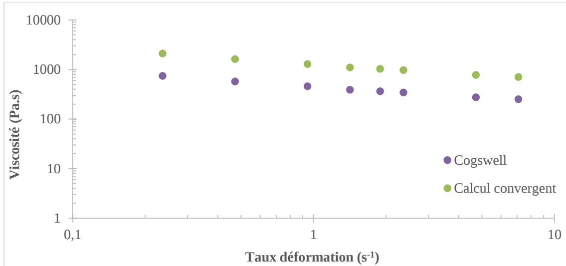
Figure 44 : Viscosité élongationnelle du plastisol F2 à \phi=63,5\% . Comparaison de la méthode de Cogswell et de la méthode convergente pour le capillaire D=0,50 mm
