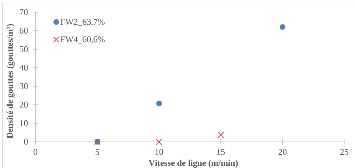
Figure 126 : Densité de gouttes en fonction de la vitesse de ligne pour FW2 à \phi=63,7\% et FW4 à \phi=60,6\% pour une épaisseur déposée de 0,10 mm
