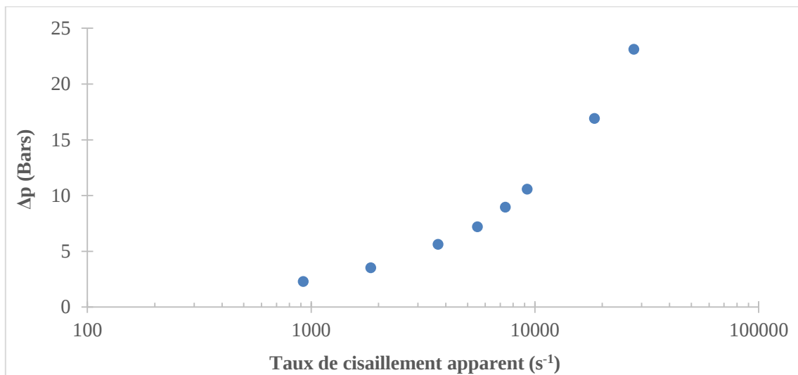
Figure 43 : Corrections de pression d'entrée en fonction du taux de cisaillement aval, avec le capillaire D=0,50 mm pour F2 à \phi=63,5\%
