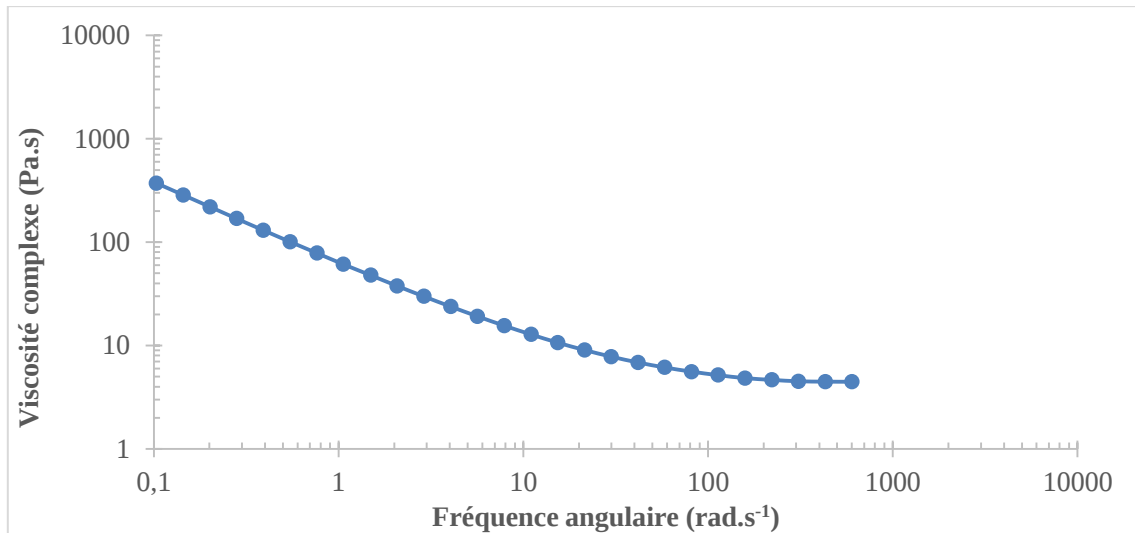
Figure 32 : Balayage en fréquence à une déformation de 1% de F2 à \phi=63\%
