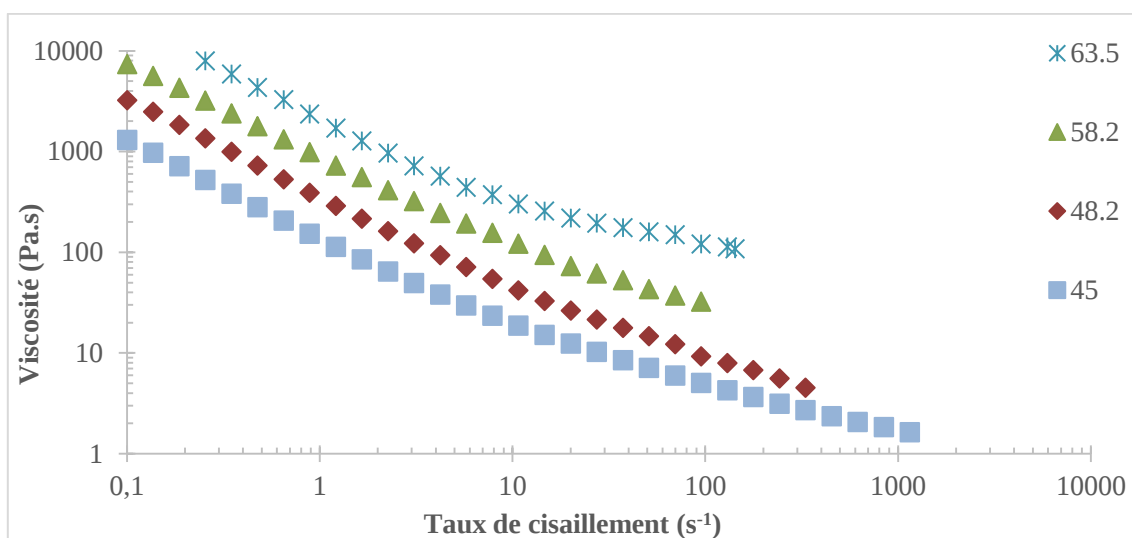
Figure 48 : Mesures de viscosité pour les formulations multimodales (F1) à taux de particules de PVC variable
