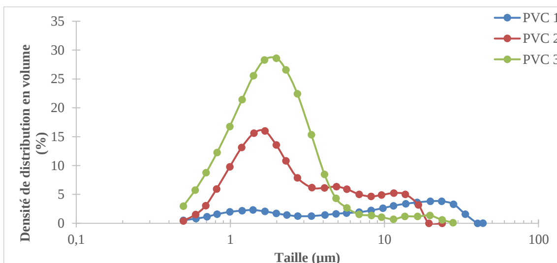
Figure 28 : Distribution volumique de taille des particules et des agglomérats de PVC
