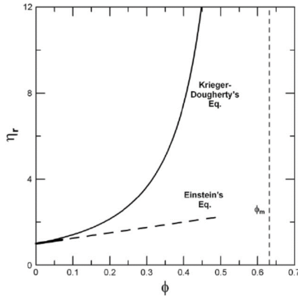
Figure 15 : Viscosité relative en fonction de la fraction volumique de charge ; comparaison de la loi d'Einstein et de la loi de Krieger Dougherty. La fraction volumique maximale est \phi_m=0,63
