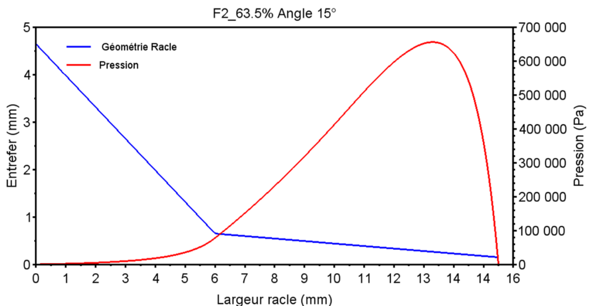
Figure 91 : Pic de pression pour F2 à \phi=63,5\% , vitesse 20 m/min, angle 15°, entrefer final 0,15 mm
