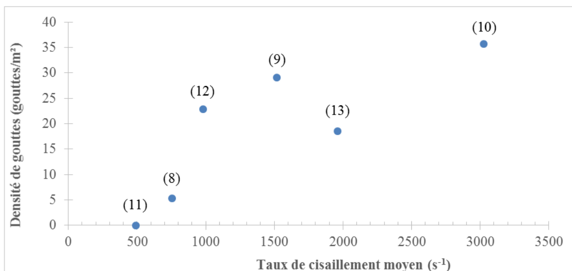
Figure 123 : Densité de gouttes en fonction du taux de cisaillement moyen pour FWW à \phi=63,6\%
