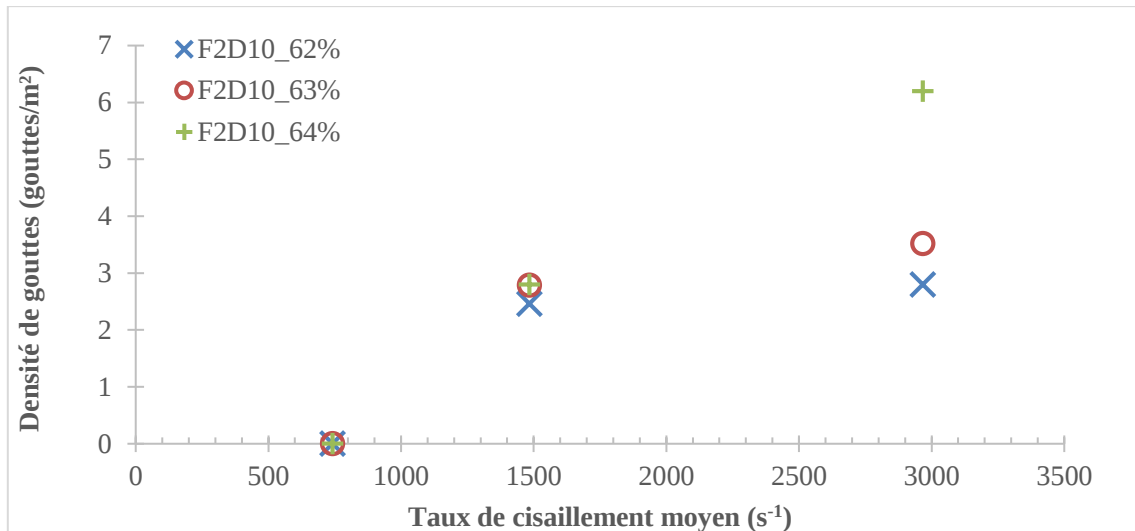
Figure 116 : Influence du taux de cisaillement sur la densité de gouttes pour F2D10 à \phi=62, 63 et 64\% pour une épaisseur déposée à 0,10 mm
