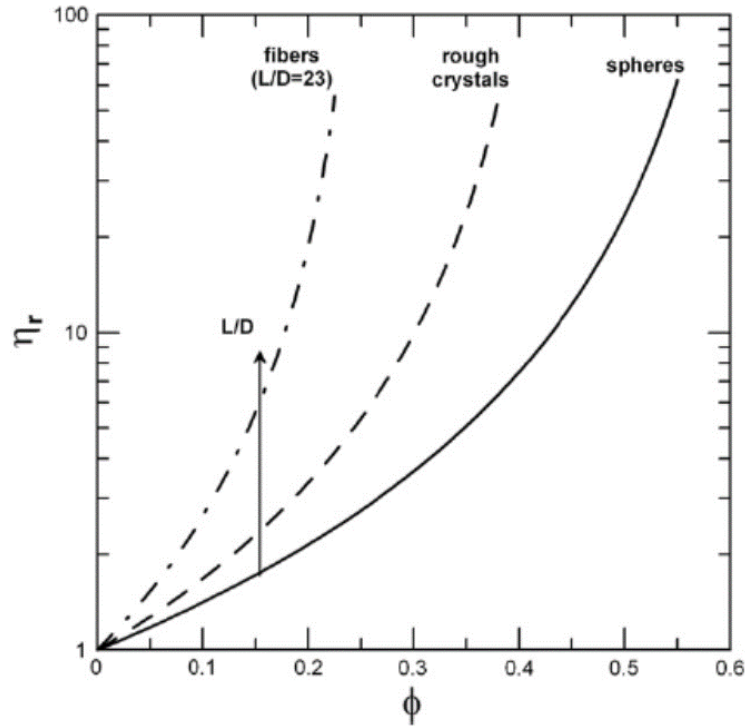
Figure 18 : Évolution de la viscosité relative en fonction de la fraction volumique solide pour des charges sphériques, des charges rugueuses et des fibres (Genovese 2012)
