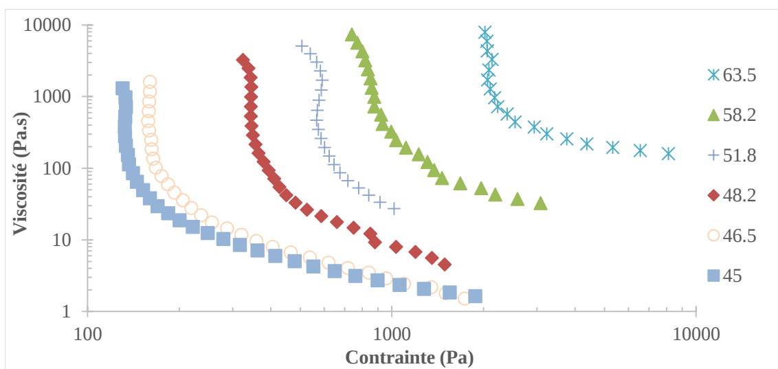
Figure 49 : Viscosité de la formulation F1 en fonction de la contrainte de cisaillement pour différents taux de particules PVC
