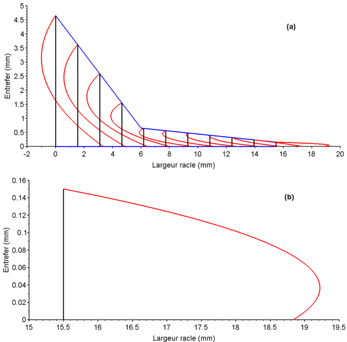
Figure 85 : (a) Champ de vitesse entre la racle et le cylindre et (b) Profil de vitesse en sortie dans le cas Newtonien, pour un angle de 15°, un entrefer de 0,15 mm à une vitesse de ligne de 20 m/min
