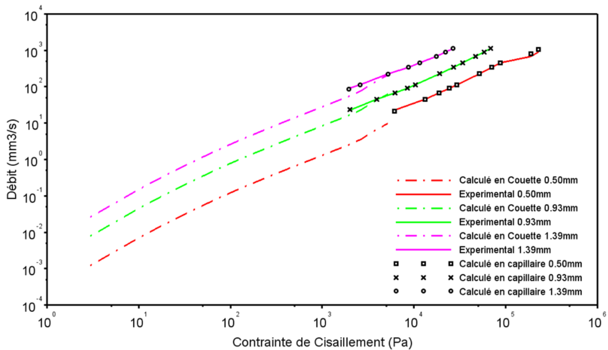
Figure 77 : Débit en fonction de la contrainte de cisaillement à la paroi pour F2D40 à \phi=63,9\% , (—) : courbes expérimentales capillaires pour les 3 diamètres ; (— · —) : débits capillaires recalculés pour chaque diamètre à partir des données Couette ; débits recalculés pour un diamètre de (□) : 0,50 mm, (×) : 0,93 mm et (○) : 1,39 mm à partir des données rhéologiques capillaires de la Figure 76
