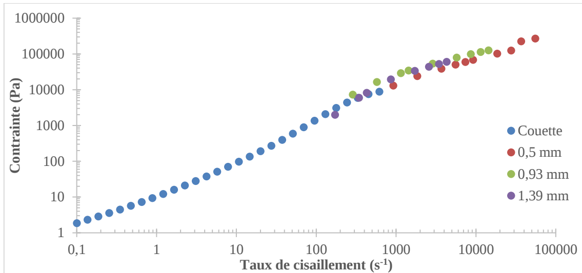
Figure 70 : Courbe de contrainte en fonction du taux de cisaillement pour la formulation F2 à \phi=63,5\% en rhéométrie Couette et en rhéométrie capillaire pour 3 diamètres ( D=0,5 ; 0,93 et 1,39\text{mm} )
