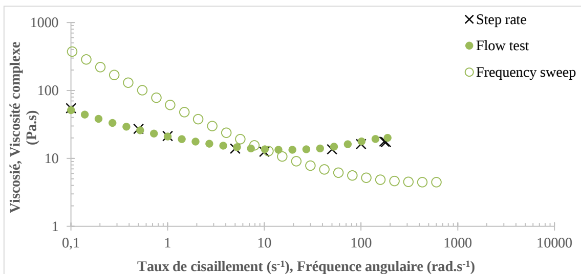
Figure 35 : Viscosité et viscosité dynamique (à 1% de déformation) en fonction du taux de cisaillement et de la fréquence angulaire pour F2 à \phi=63\%
