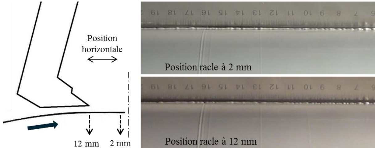
Figure 110 : Montée du dépôt de F2D10 à \phi=63\% à deux positions horizontales de la racle par rapport à la verticale de l'axe de rotation du cylindre après 10 min d'enduction
