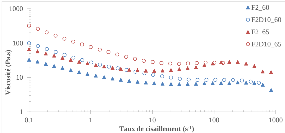
Figure 53 : Formulation avec charge (F2D10) et sans charge (F2) : Influence de la substitution de particules de PVC par des particules de \text{CaCO}_3 sur la viscosité pour deux taux de charge global différents \phi=60 et 65\% (rhéologie Couette)
