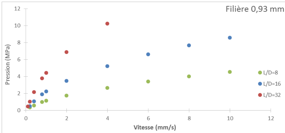
Figure A. 5 : Mesures de pressions à différentes vitesses pour le capillaire de diamètre 0,93 mm à différents ratio L/D pour F2
