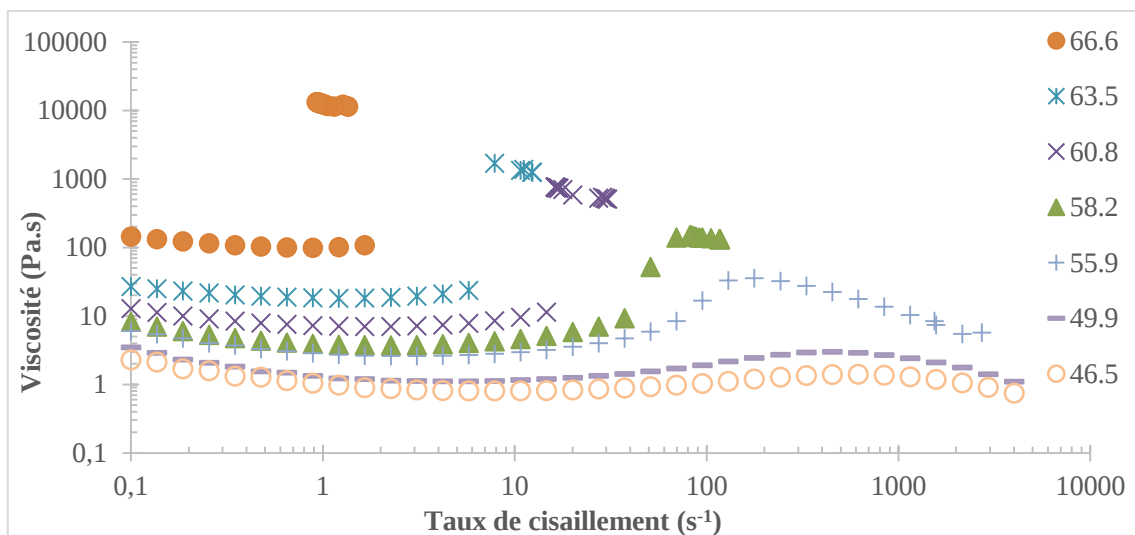
Figure 51 : Comportement rhéologique de formulations monomodales (F3) à différents taux de charge
