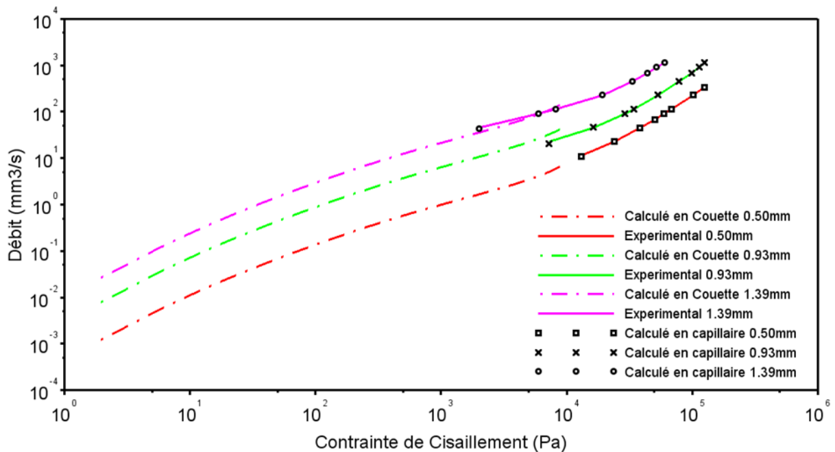
Figure 71 : Débit en fonction de la contrainte de cisaillement à la paroi pour F2 à \phi=63,5\% , (—) : courbes expérimentales capillaires pour les 3 diamètres ; (— · —) : débits capillaires recalculés pour chaque diamètre à partir des données Couette ; débits recalculés pour un diamètre de ( \square ) : 0,50\text{ mm} , ( \times ) : 0,93\text{ mm} et ( \circ ) : 1,39\text{ mm} à partir des données rhéologiques capillaires de la Figure 69
