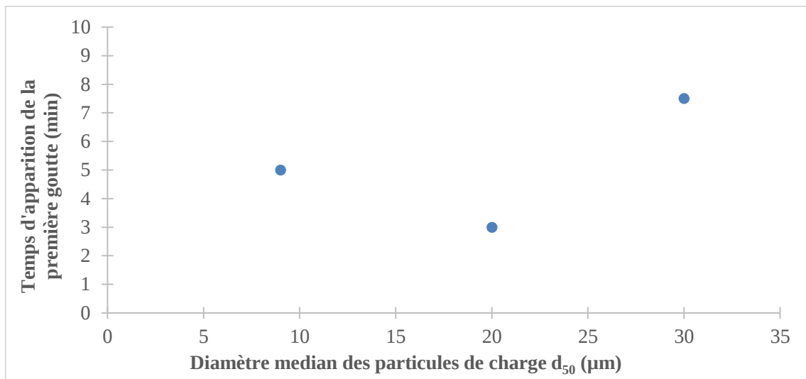
Figure 118 : Influence du diamètre médian ( d_{50} ) de la charge sur le temps d'apparition de la première goutte pour F2 avec charges minérales à \phi=64\% pour une vitesse de 20 m/min et une épaisseur déposée de 0,10 mm
