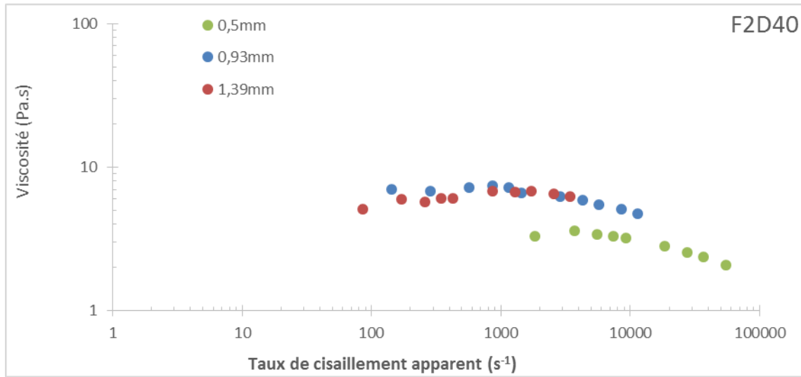
Figure A. 13 : Viscosité en fonction du taux de cisaillement pour F2D40
