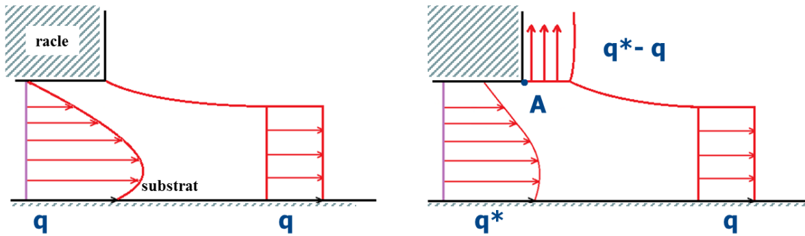
Figure 148 : Mécanisme de glissement-adhésion
