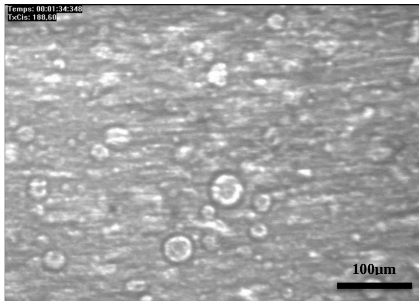
Figure 63 : Image de la rhéologie optique de F2 à \phi=63\% à 188\text{s}^{-1}
