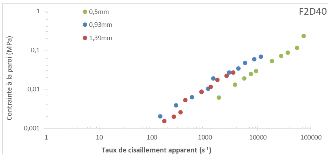
Figure A. 12 : Contrainte à la paroi en fonction du taux de cisaillement apparent pour F2D40
