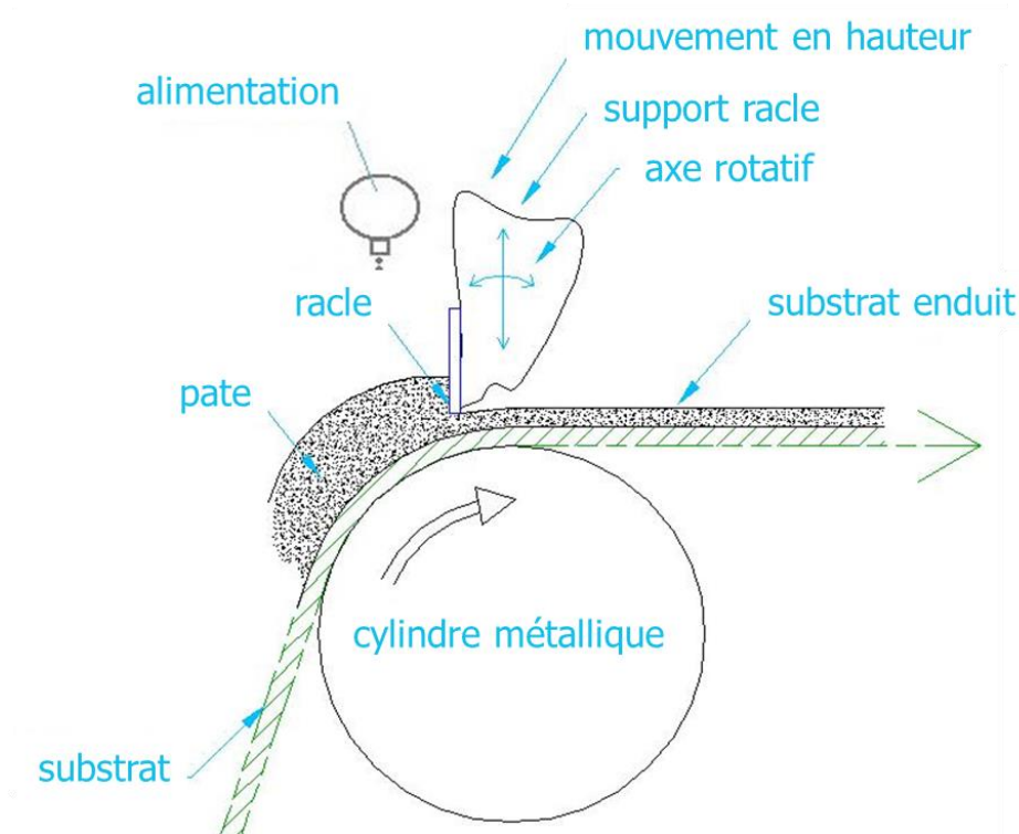
Figure 6 : Procédé d'enduction à la racle
