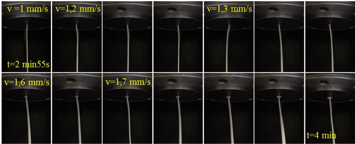
Figure 132 : Images d'extrudât de la formulation F2 à \phi=63\% prises toutes les 5 secondes pour 5 vitesses différentes
