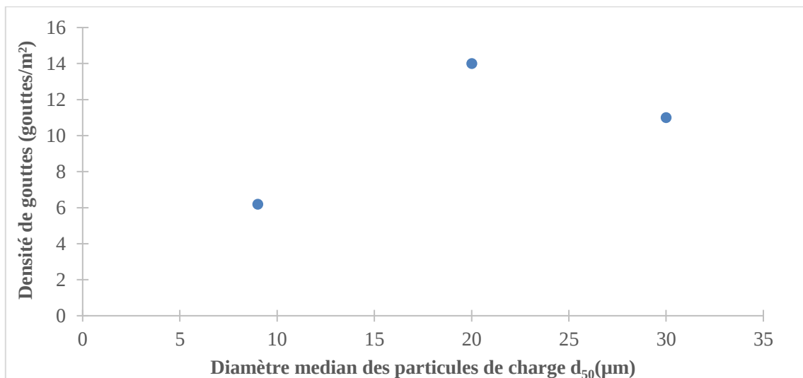
Figure 117 : Effet de la taille moyenne des particules de charge sur le défaut pour F2 avec charges minérales à \phi=64\% à 10 m/min
