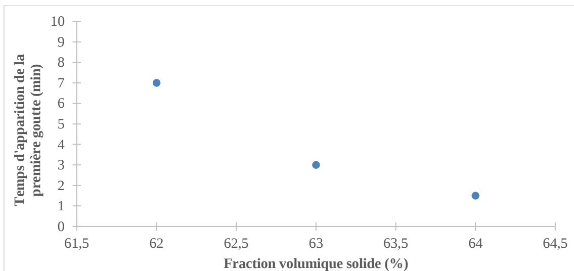
Figure 115 : Influence de la fraction volumique solide de F2D10 sur le temps d'apparition de la première goutte pour une épaisseur déposée de 0,10 mm et une vitesse de 10 m/min
