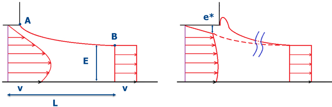
Figure 143 : Rupture de la surface libre du plastisol en sortie de racle
