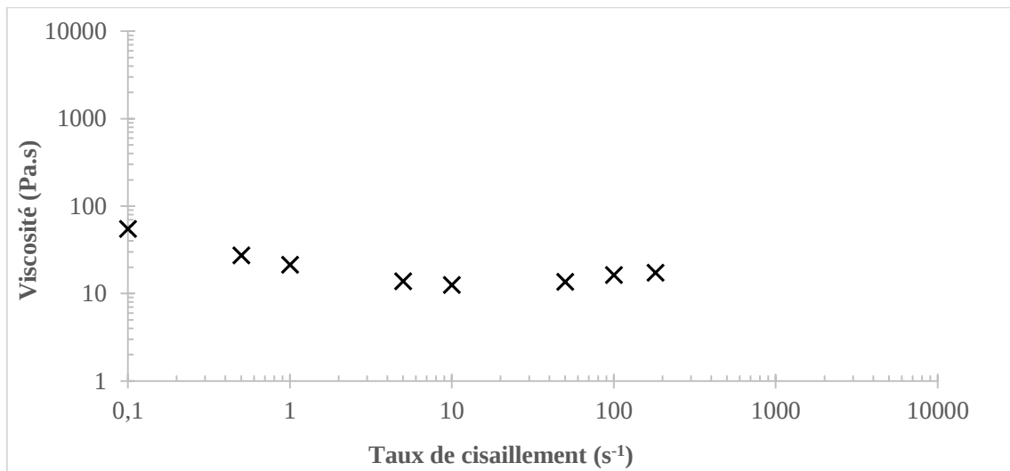
Figure 33 : Viscosité mesurée à taux de cisaillement imposé (palier de 500 s) pour F2 à 63%
