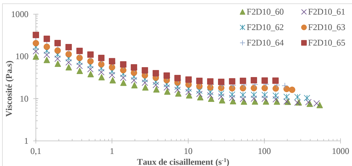
Figure 57 : Influence de la fraction volumique globale sur la viscosité de formulations F2D10
