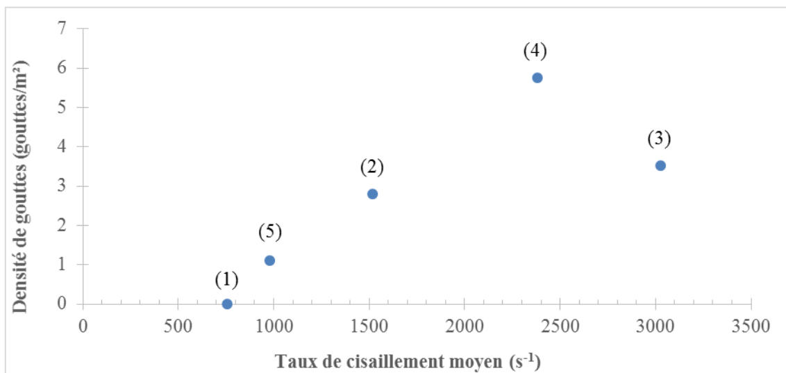
Figure 113 : Densité de gouttes en fonction du taux de cisaillement moyen pour F2D10 à \phi=63\%
