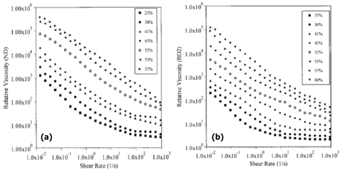
Figure 19 : Évolution de la viscosité relative de latex de polystyrène pour des distributions de tailles étroites (a) ou larges (b) à différentes fractions volumiques solides (Luckham et Ukeje 1999)
