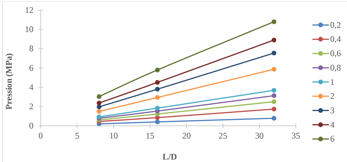
Figure 38 : Mesures de pressions en fonction de L/D à différentes vitesses pour le capillaire de diamètre 0,93 mm pour F2 à \phi=63\% .
