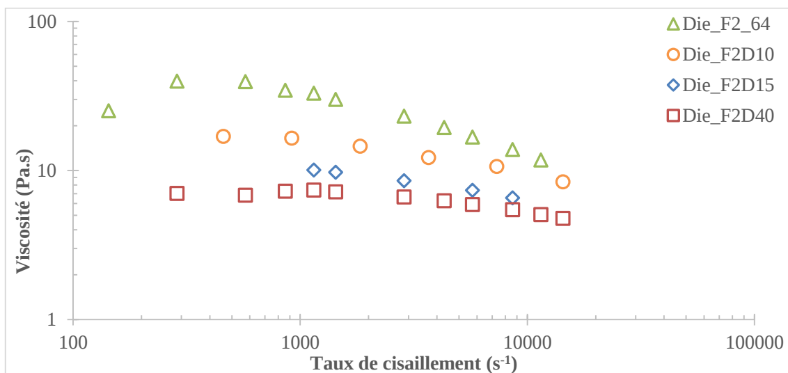
Figure 55 : Mesures rhéologiques au rhéomètre capillaire D=0,93 \text{ mm} pour les formulations F2, F2D10, F2D15 et F2D40 pour un taux de charge global \phi \approx 64\%
