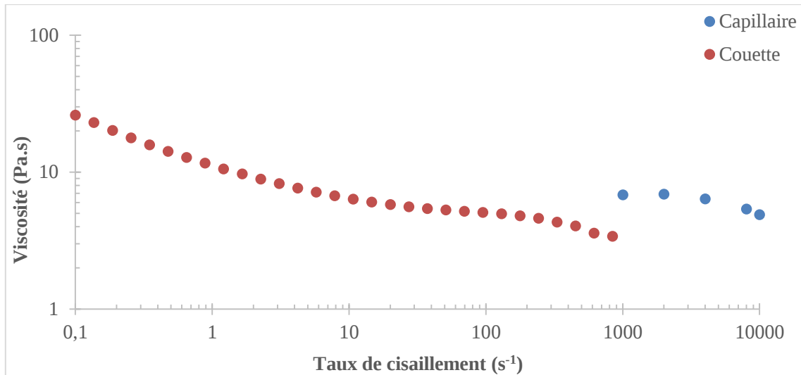
Figure 66 : Mesures rhéologiques au rhéomètre de Couette et capillaire D=0,93 mm pour la formulation industrielle de plastisol FWW à \phi=63,6\%
