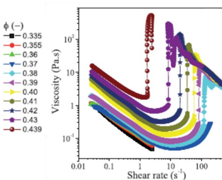
Figure 22 : Évolution de la viscosité en fonction du taux de cisaillement pour des suspensions de fécule de maïs dans l'eau à fraction volumique croissante (Fall et al. 2015)
