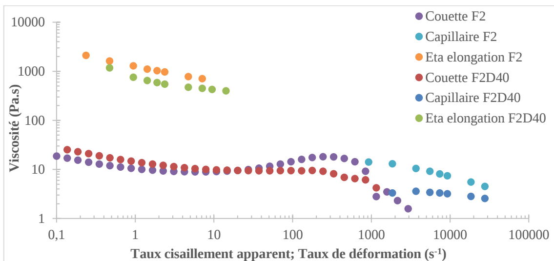
Figure 145 : Comparaison rhéologie élongationnelle et rhéologie en cisaillement, produit non chargé (F2 à \phi=63,5\% ) et produit chargé (F2D40 à \phi=63,9\% )
