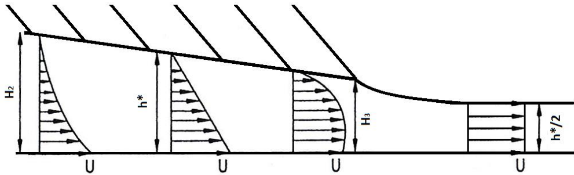
Figure 83 : Profil de vitesse sous la seconde partie de la racle.
