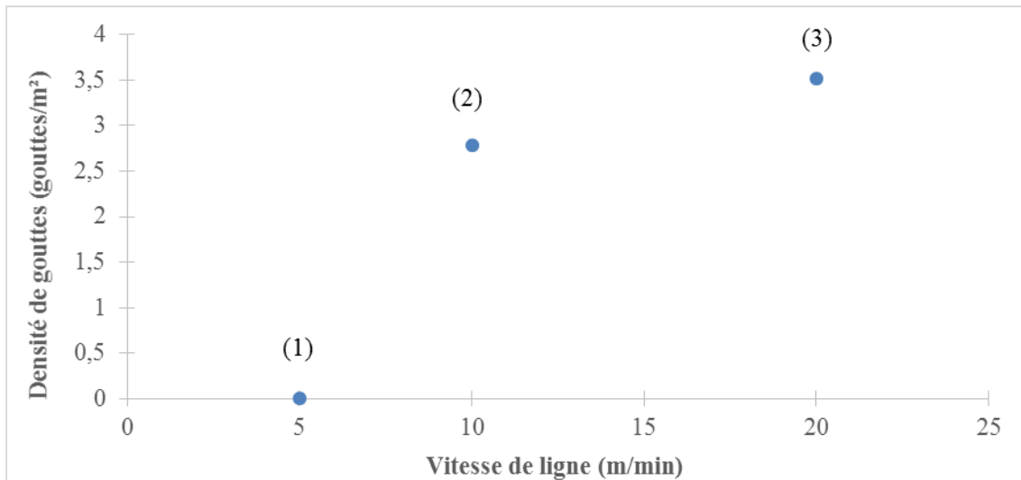
Figure 108 : Influence de la vitesse de ligne sur F2D10 à \phi=63\% pour une épaisseur déposée de 0,10 mm
