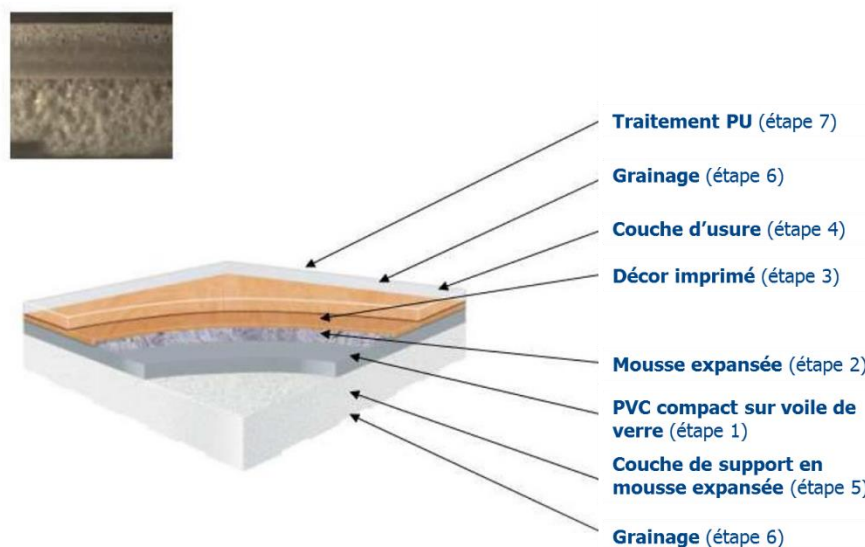
Figure 4 : Description d'un revêtement vinyle hétérogène
