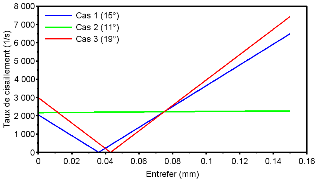
Figure 88 : Variation du taux de cisaillement à l'entrefer final H_3=0,15 mm en sortie de racle
