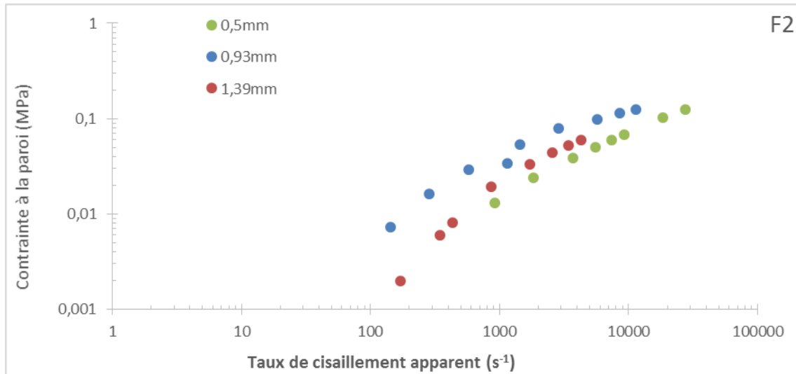
Figure A. 7 : Contrainte à la paroi en fonction du taux de cisaillement apparent pour F2
