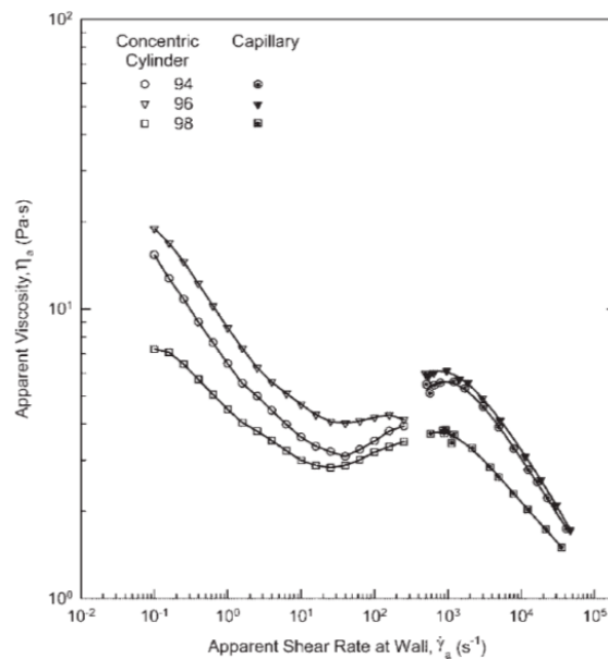
Figure 25 : Viscosité de plastisol en fonction du taux de cisaillement, (Nakajima et Harrell 2010)
