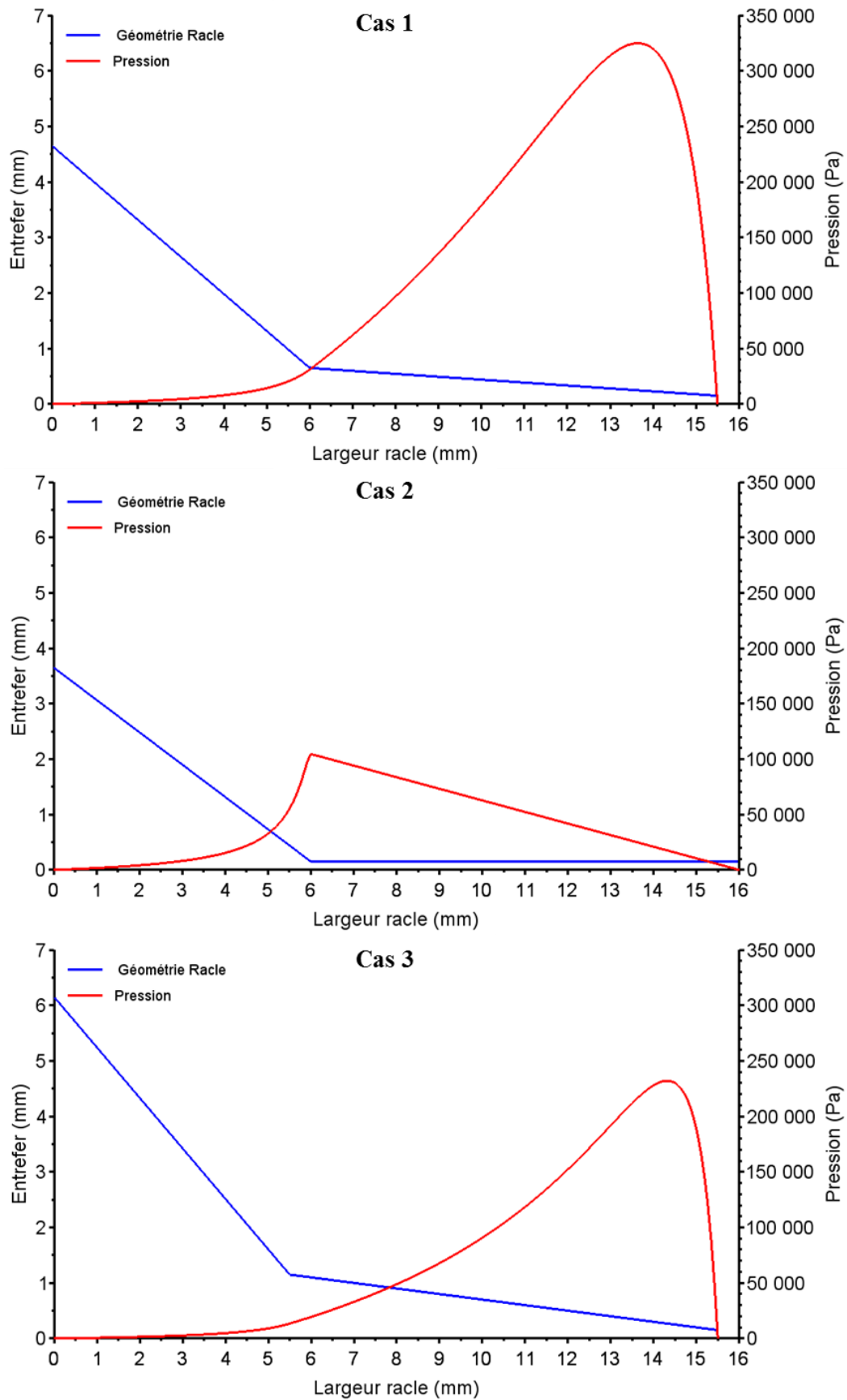
Figure 86 : Variation de la pression sous la racle pour les 3 cas (angle 15, 11 et 19°) à 20 m/min
