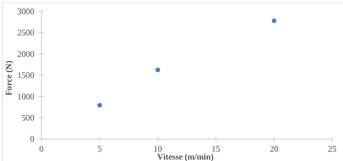
Figure 93 : Force sous la racle en fonction de la vitesse de ligne pour F2 à \phi=63,5\% pour un entrefer final de 0,15 mm et an angle de 15^\circ
