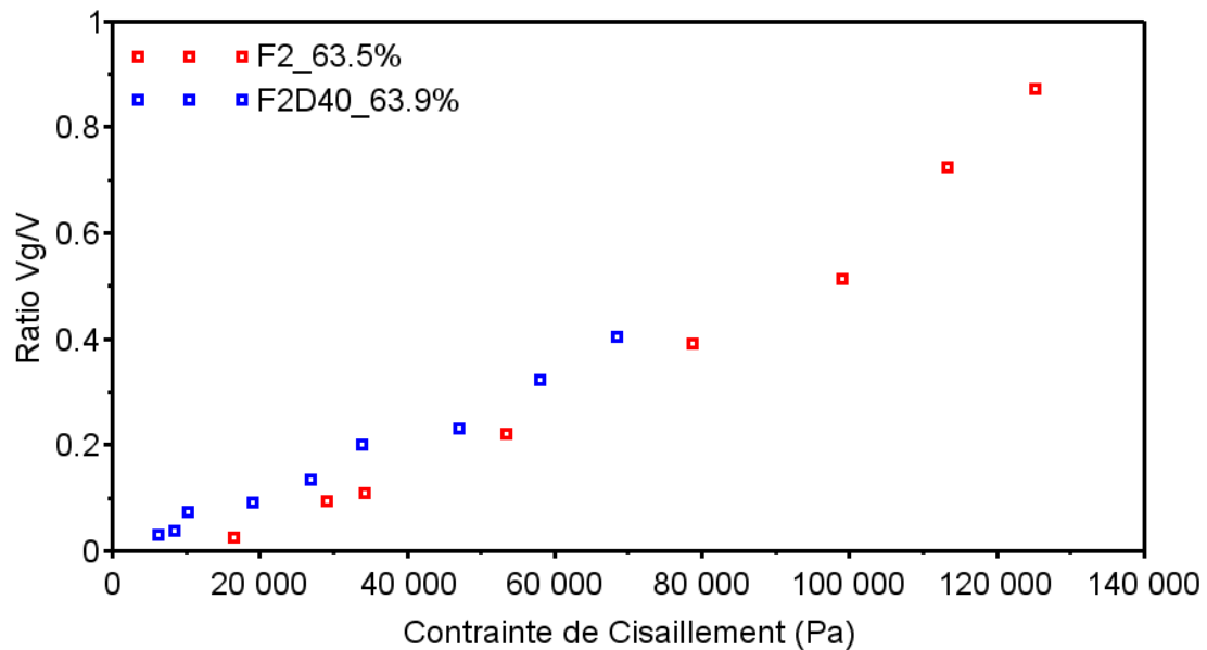
Figure 81 : Ratio de la vitesse de glissement sur la vitesse moyenne en fonction de la contrainte de cisaillement pour F2 à \phi=63,5\% et F2D40 à \phi=63,9\%
