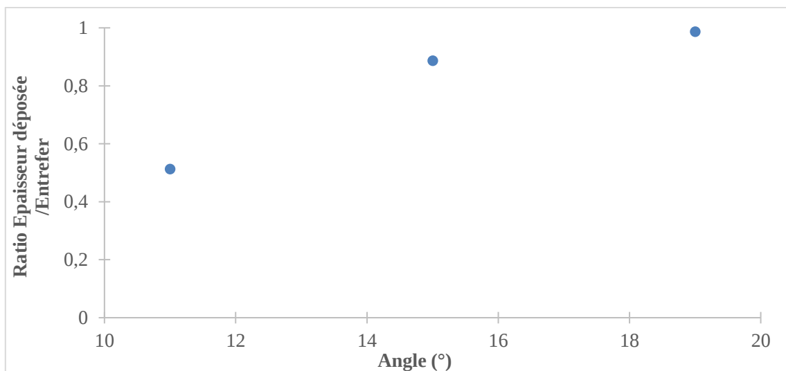
Figure 97 : Ratio épaisseur déposée/entrefer en fonction de l'angle de la racle pour F2 à \phi=63,5\%
