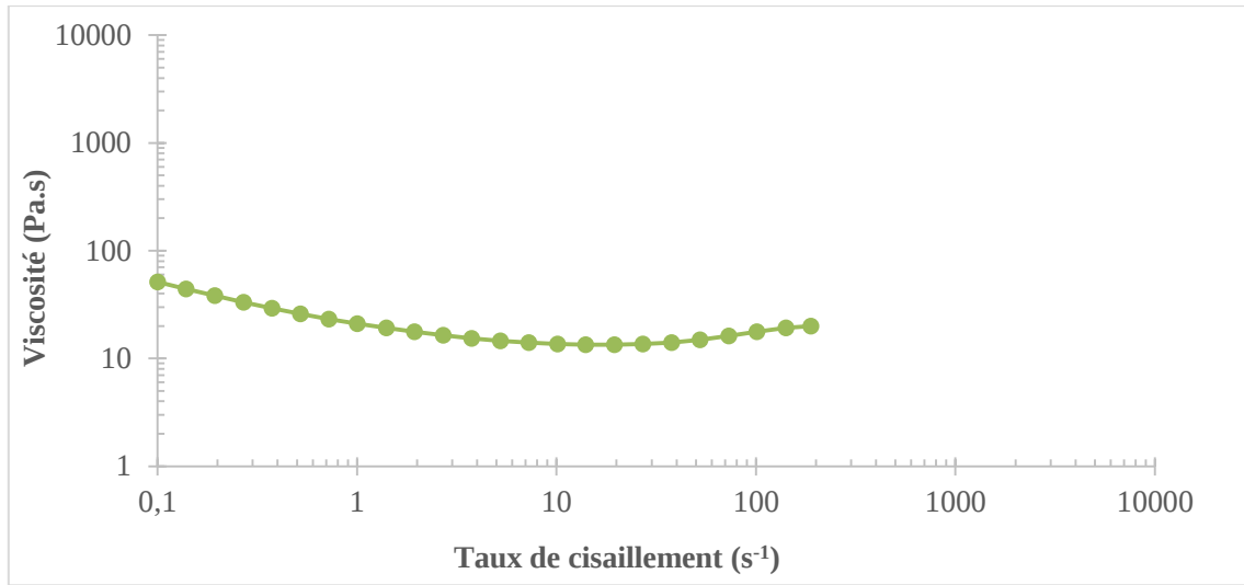
Figure 34 : Viscosité mesurée en accélération pour F2 à \phi=63\%
