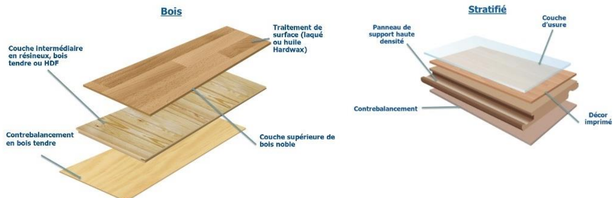
Figure 2 : Composition des revêtements bois et stratifié
