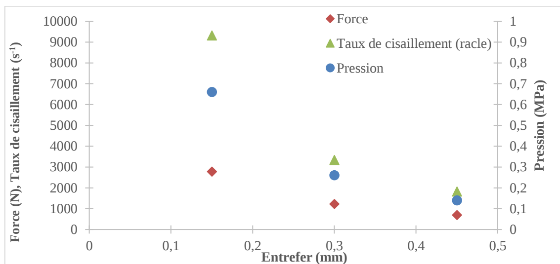
Figure 94 : Force exercée sous la racle, taux de cisaillement maximal le long de la racle et pression maximale induite sous la racle en fonction de l'entrefer final pour F2 à \phi=63,5\%
