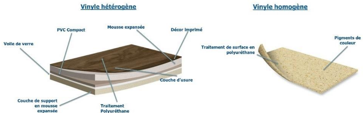
Figure 1 : Composition des revêtements vinyle hétérogène et homogène
