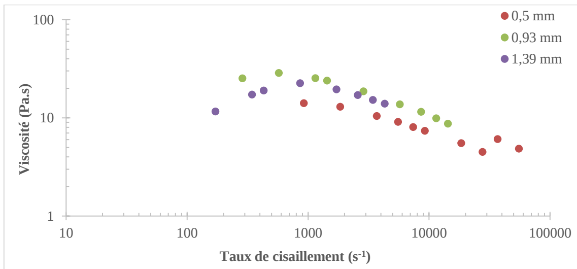
Figure 41 : Viscosité en fonction du taux de cisaillement pour les diamètres de capillaires 0,50 ; 0,93 et 1,39 mm pour F2 à \phi=63,5\%
