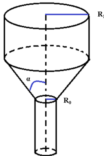
Figure A. 1 : Géométrie du convergent entre le réservoir du rhéomètre capillaire et la filière
