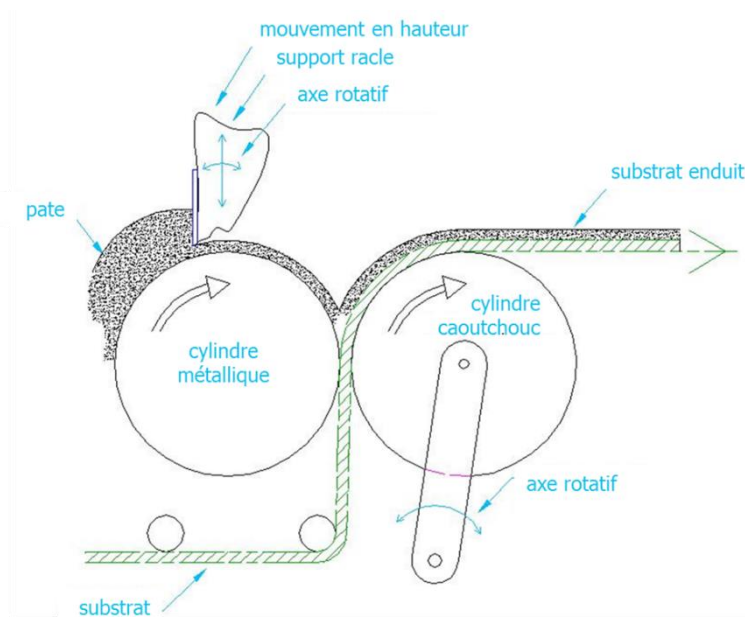
Figure 9 : Procédé d'enduction en « semi reverse roll »
