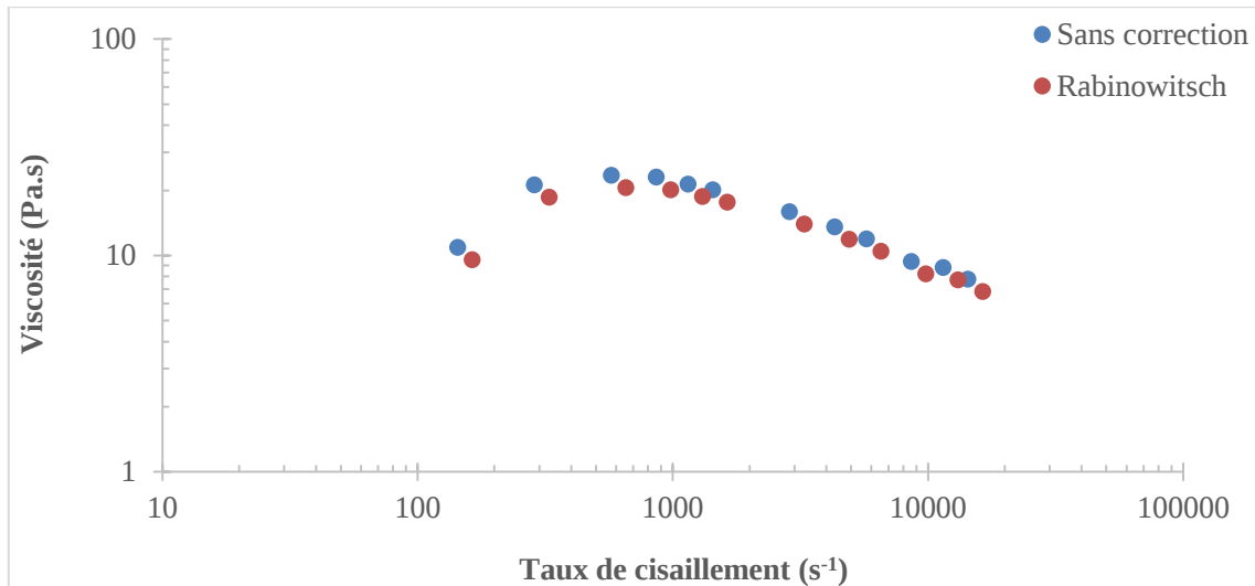
Figure 40 : Viscosité capillaire avec et sans corrections de Rabinowitsch en fonction du taux de cisaillement pour le diamètre 0,93 mm pour F2 à \phi=63\%
