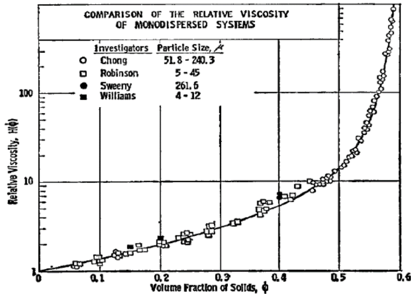
Figure 16 : Viscosité relative en fonction de la fraction volumique solide pour différentes tailles de particules, (Farris 1968)
