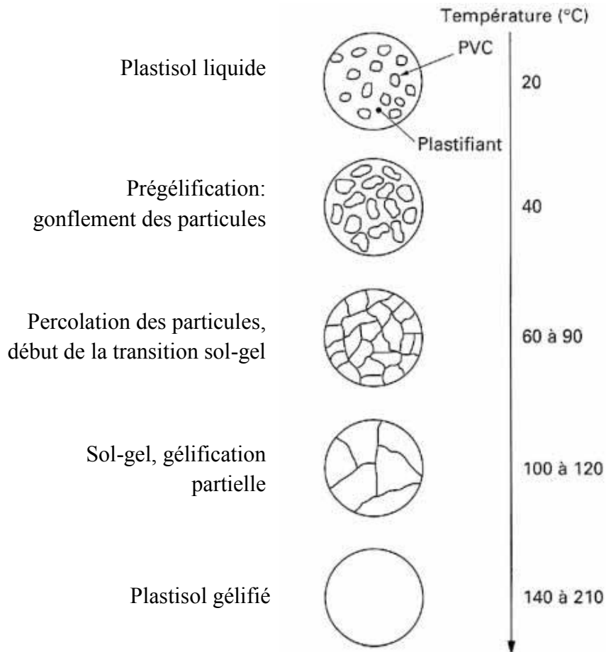
Figure 11 : Prégélification et gélification d'un plastisol (d'après Georget (1996))
