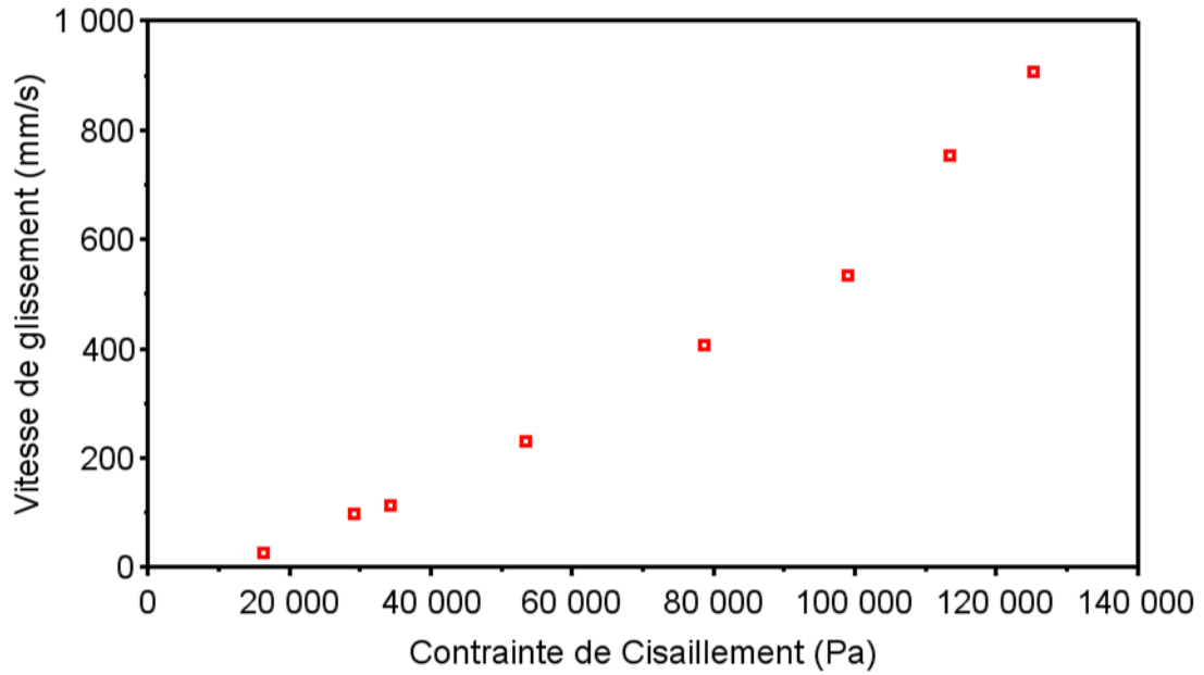
Figure 74 : Vitesse de glissement en fonction de la contrainte de cisaillement au diamètre 0,50 mm pour F2 à \phi=63,5\%
