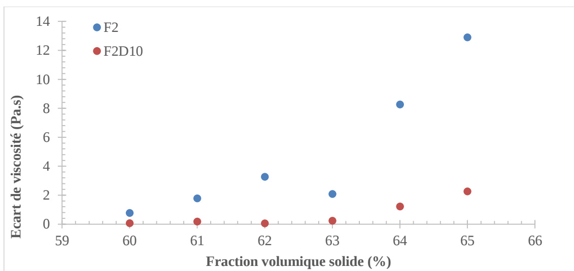
Figure 59 : Écart de viscosité entre le pic de dilatance et le plateau Newtonien pour les formulations F2 et F2D10
