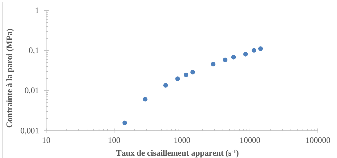
Figure 39: Contrainte à la paroi en fonction du taux de cisaillement apparent pour le diamètre 0,93 mm pour F2 à \phi=63\%
