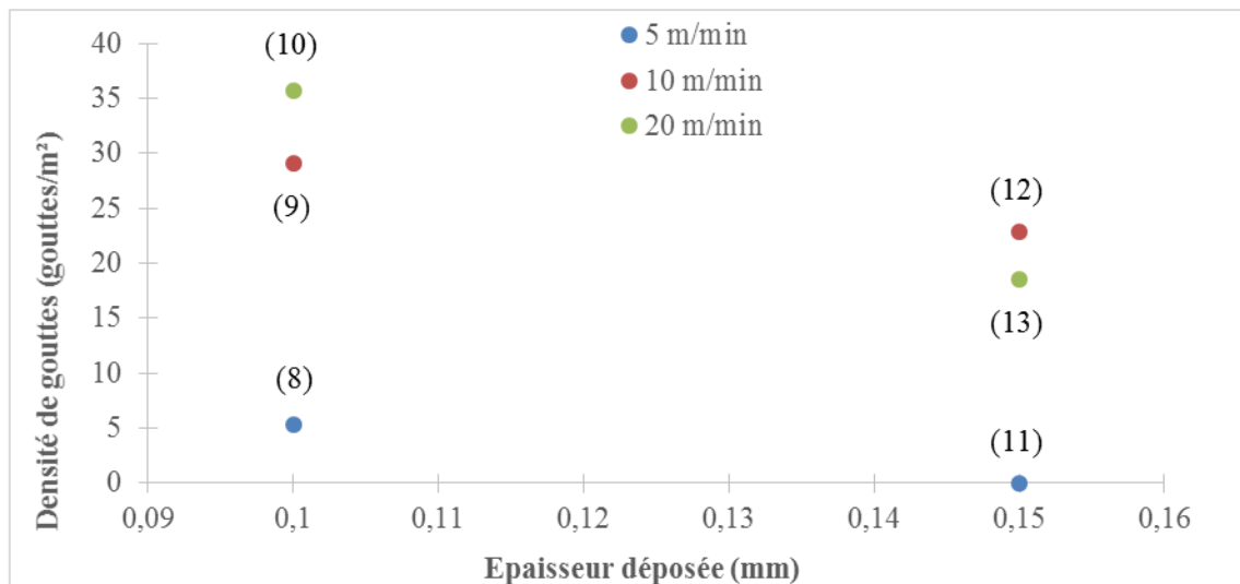
Figure 121 : Influence de l'épaisseur déposée sur le défaut de goutte pour FWW à \phi=63,6\% à 5, 10 et 20 m/min
