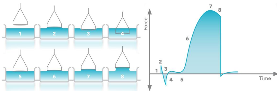
Figure 146 : Dispositif d'extraction d'une lamelle de plastisol à vitesse contrôlée
