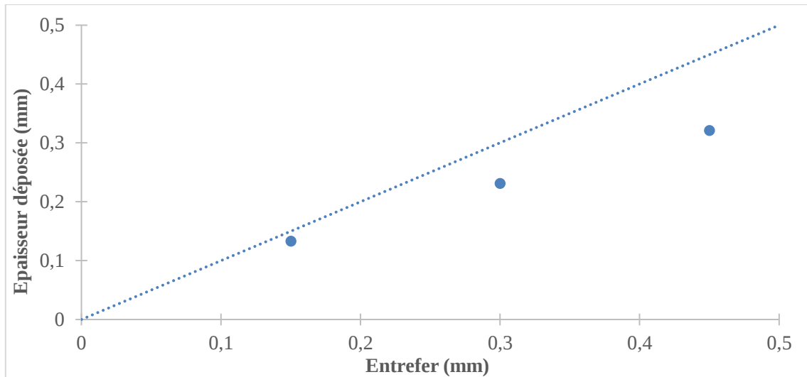
Figure 95 : Épaisseur déposée calculée pour la rhéologie réelle (F2 à \phi=63,5\% ) en fonction de l'entrefer final
