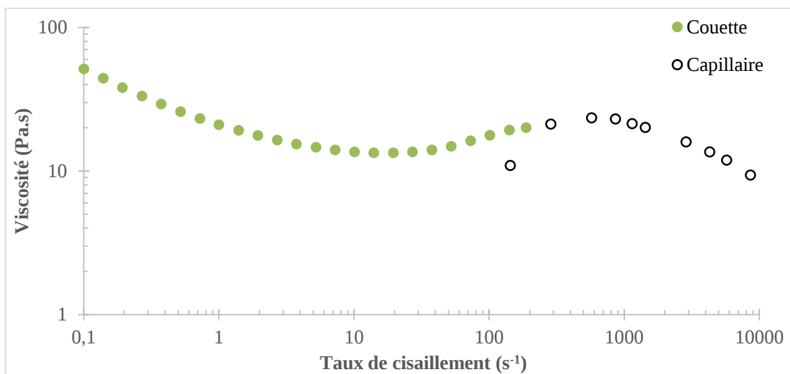
Figure 42 : Comparaison entre les mesures en rhéométrie de Couette et les mesures en rhéométrie capillaire pour un diamètre 0,93 mm pour F2 à \phi=63\%
