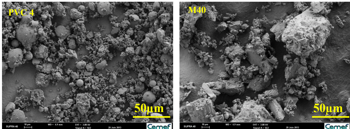
Figure 5 : Image MEB d'une résine PVC et d'une charge craie
