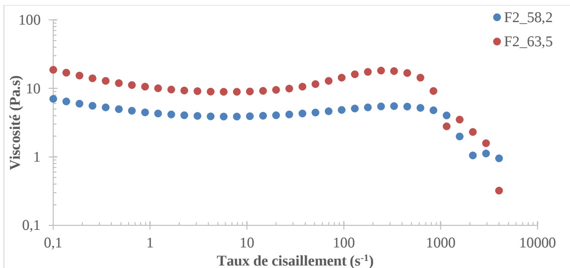
Figure 137 : Évolution de la viscosité en fonction du taux de PVC et du taux de plastifiant pour la formulation F2
