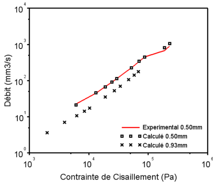
Figure 79 : Courbe d'écoulement expérimentale obtenue en capillaire pour un diamètre 0,50 mm comparée à la courbe des débits calculés à partir de la rhéologie capillaire pour un diamètre 0,50 mm et 0,93 mm, pour F2D40 à \phi=63,9\%
