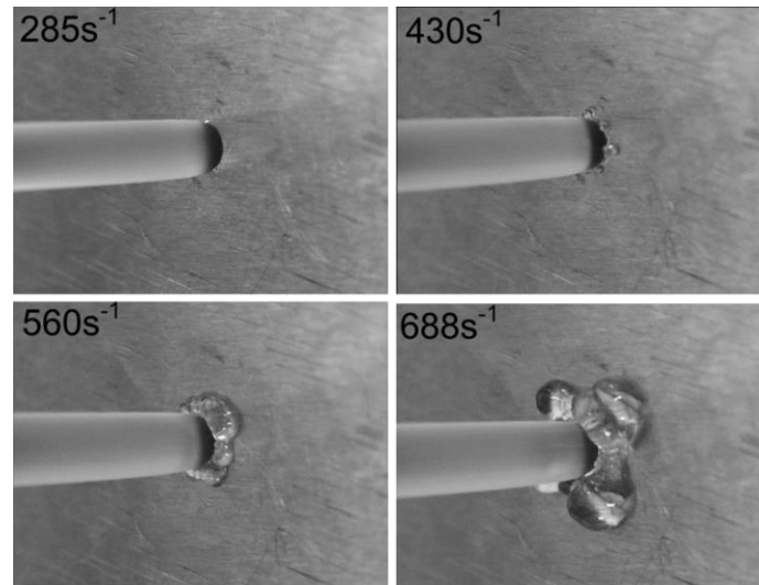
Figure 139 : Exemple de dépôt en sortie de filière d'extrusion (Musil and Zatloukal 2011)
