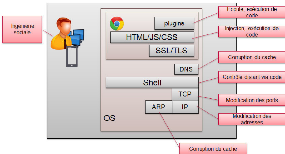
FIGURE 2.7 – Menaces sur les clients Web
