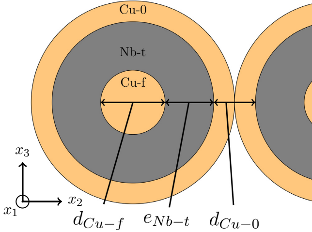
Fig. 4. Largeur théorique des canaux \delta : sur le Zoom 1, e_{\text{Nb-t}} désigne l'épaisseur des tubes de niobium, d_{\text{Cu-f}} le diamètre des filaments de cuivre, d_{\text{Cu-0}} la largeur des canaux de cuivre.
