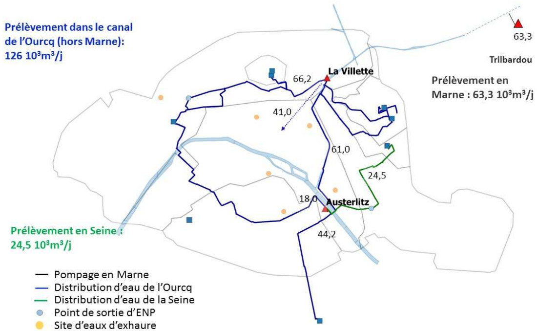
Figure 64 : Modèle hydraulique construit pour le scenario «Ourcq». Volumes journaliers indiqués en 10^3 \text{ m}^3/\text{j}
