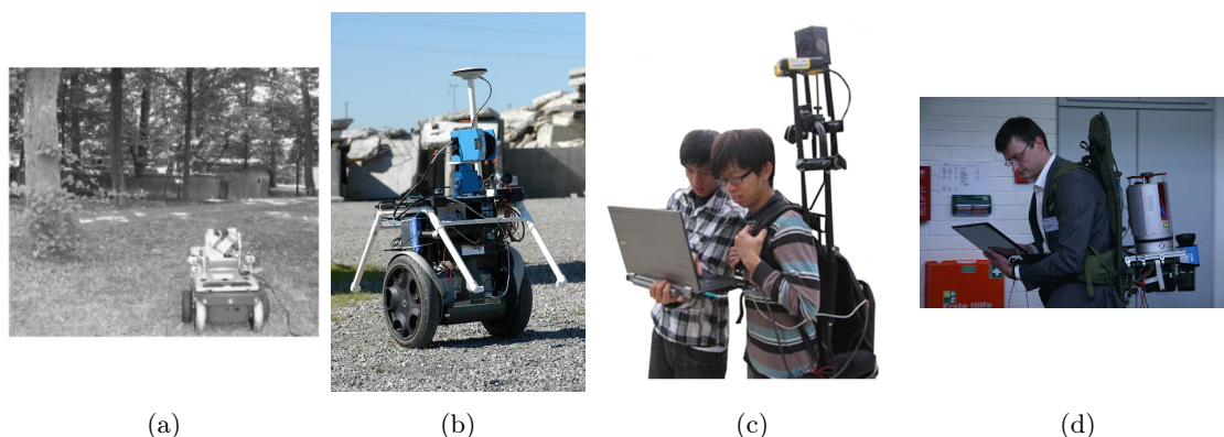
FIGURE 2.3 – Quelques exemples de systèmes mobiles : a) robot pour acquisition en extérieur [Nüchter et al. , 2007] ; b) plateforme Segway [Montemerlo et Thrun , 2006] ; c) système portable [Liao et al. , 2013] ; d) système portable [Nüchter et al. , 2015]
