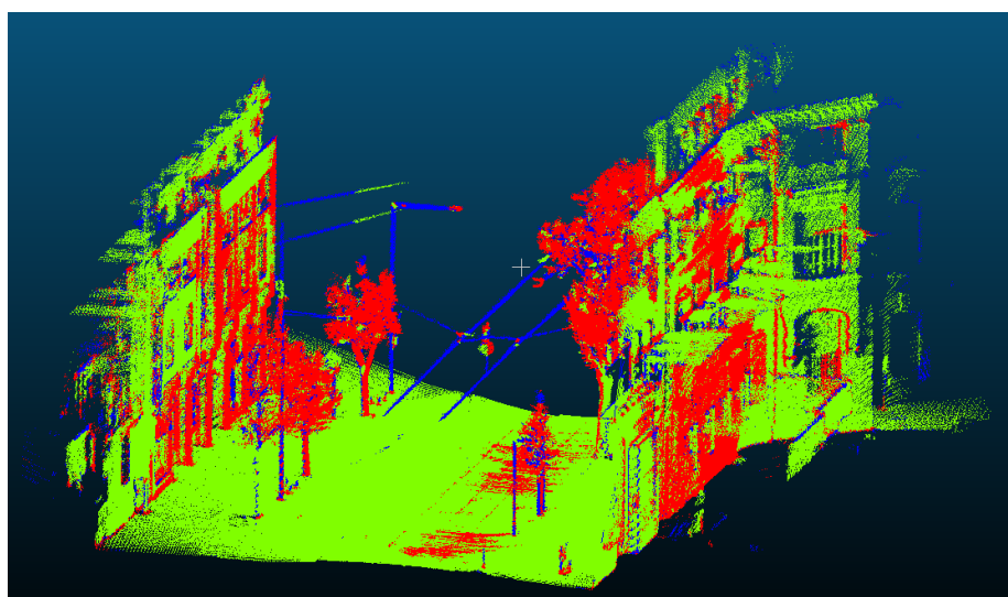
FIGURE 3.8 – Dimensionnalité calculée pour un nuage réel : en bleu, la dimensionnalité vaut 1 ; en vert, elle vaut 2, et en rouge elle vaut 3
