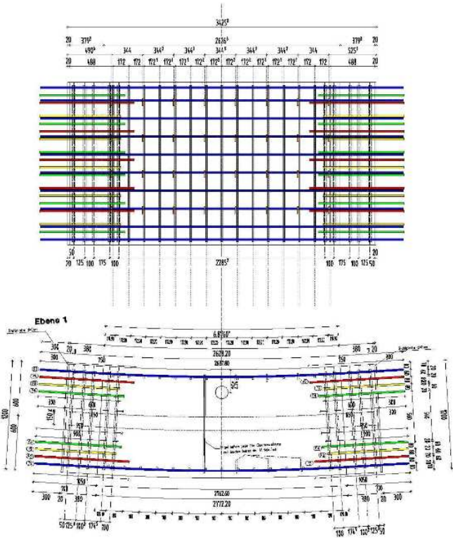
FIGURE 3.4 – Schéma de ferrailage de la structure PACE. Les armatures sont en bleu sur les faces interne et externe. Les autres barres d'acier servent à transférer les efforts entre les oreilles et le béton.
