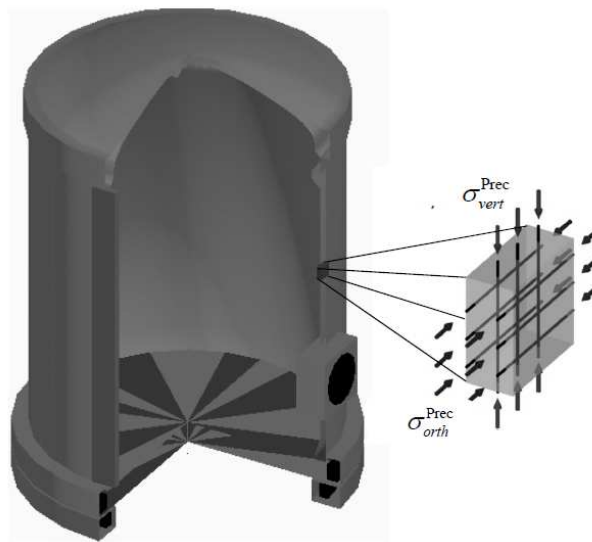
FIGURE 1.4 – Précontrainte verticale et horizontale dans l'enceinte
