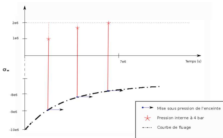
FIGURE 2.50 – Evolution de la contrainte circonférentielle dans la portion d'enceinte
