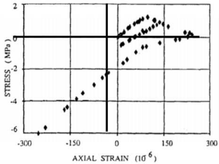
FIGURE 1.10 – Réponse du béton à une sollicitation alternée traction-compression
