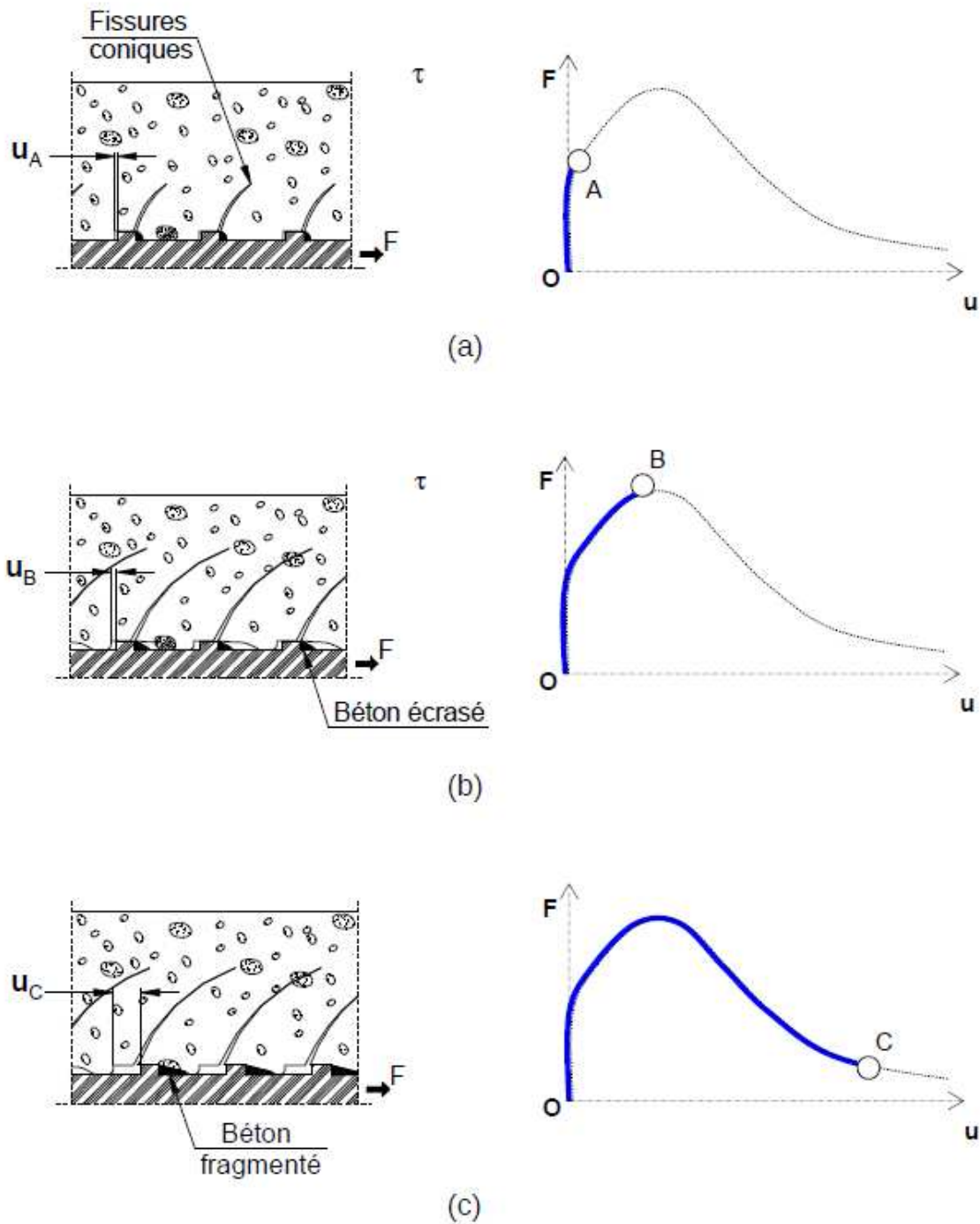
FIGURE 1.23 – Différentes étapes de dégradation de la liaison Acier-Béton
