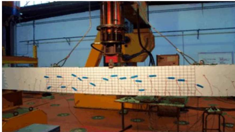
FIGURE 2.39 – Test expérimental de la poutre en flexion trois points [Giry et al., 2008]
