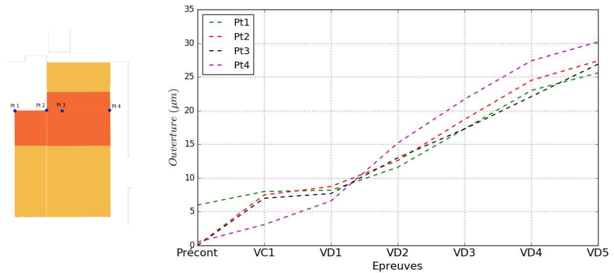
FIGURE 4.24 – Ouverture de fissure dans le temps à différents points
