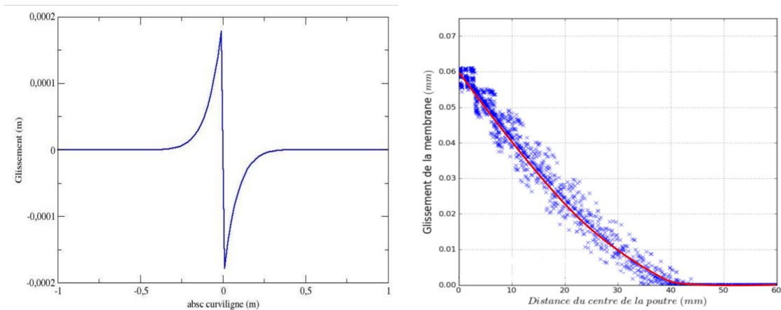
FIGURE 4.5 – Représentation de la fonction de glissement le long des armatures et comparaison au cas de la poutre de [Ghantous et al., 2016].
