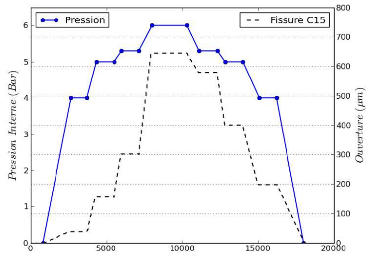
FIGURE 3.10 – Historique de pression du RUN 6 et ouverture d'une fissure C15 de la maquette PACE
