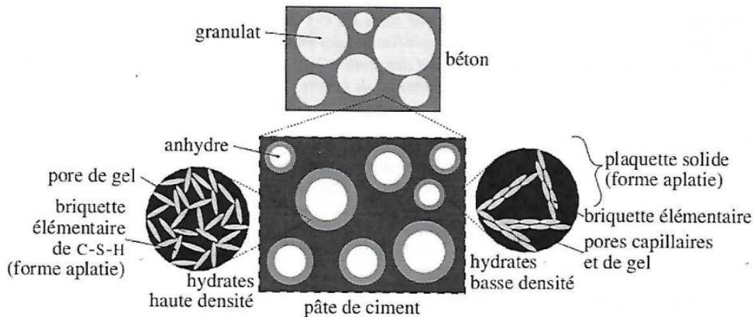
FIGURE 1.42 – Modèle morphologique multi-échelle de béton [Sanahuja, 2008]
