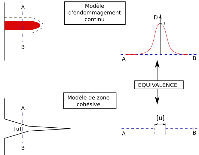
FIGURE 1.12 – Transition Endommagement - Fissure
