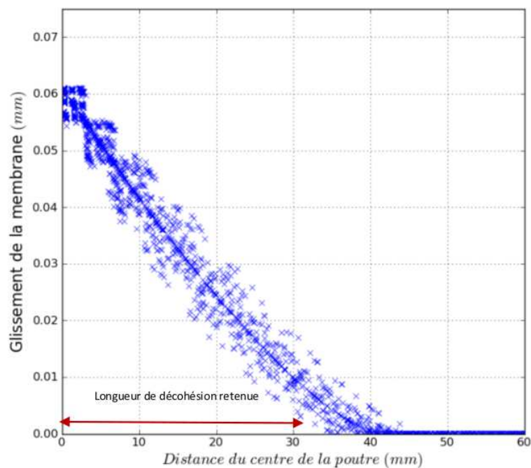
FIGURE 2.33 – Exemple de Glissement en fonction de la distance à la fissure pour tous les éléments d'interface Acier-Béton
