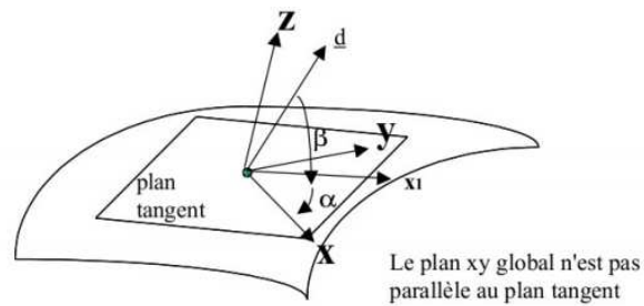
FIGURE 2.22 – Repère local des éléments membranes
