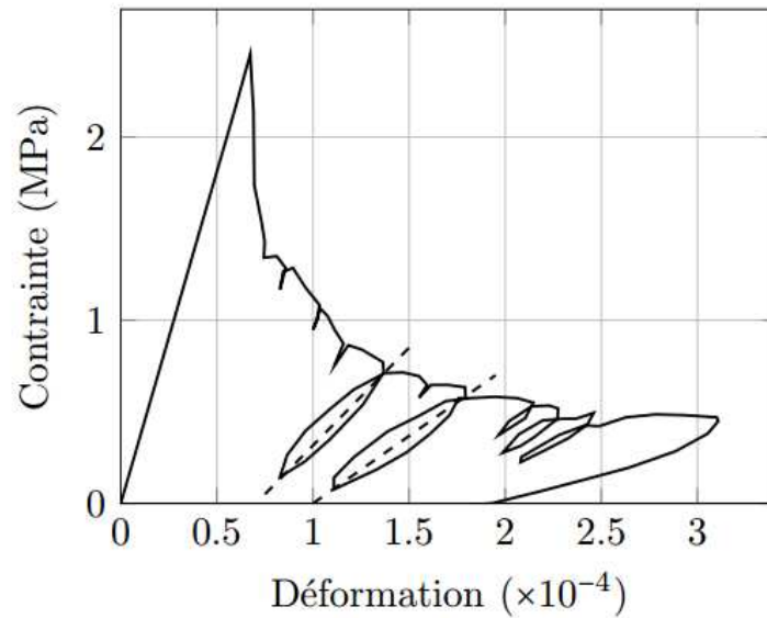
FIGURE 1.7 – Réponse contrainte-déformation en traction [Terrien, 1980]
