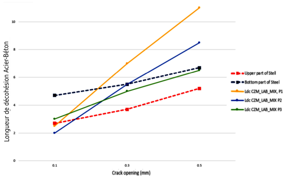
FIGURE 2.36 – Comparaison entre les longueurs de décohésion expérimentale et numérique
