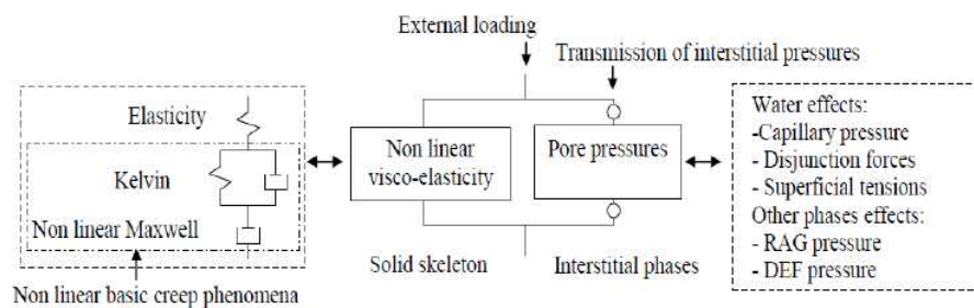
FIGURE 1.43 – Modèle poro-mécanique pour l'estimation des déformations différées [Sellier, 2006]
