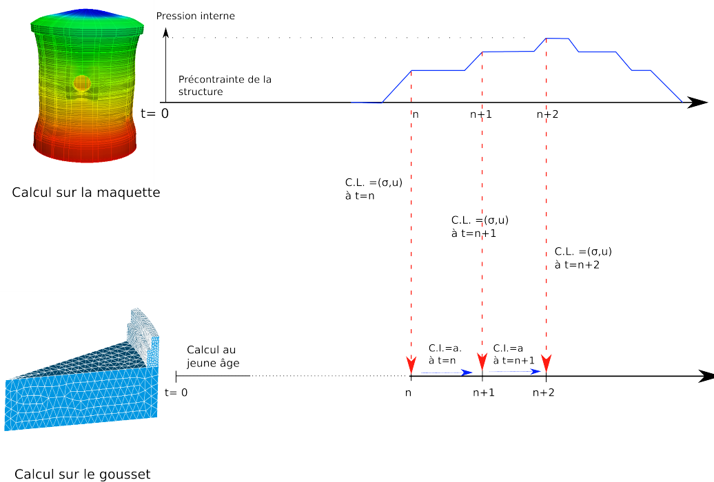
FIGURE 4.14 – Scénario de chargement lors d'une épreuve VD_n
