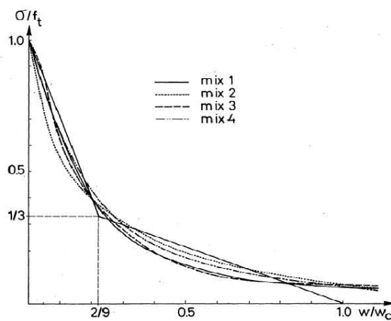
FIGURE 2.2 – Relation contrainte-ouverture uniformisée pour différents bétons et une représentation du dispositif expérimental de l'éprouvette en traction
