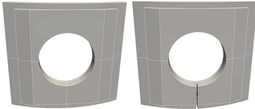
FIGURE 3.35 – Ouverture de la fissure dans le TAM à 0.7 bars
