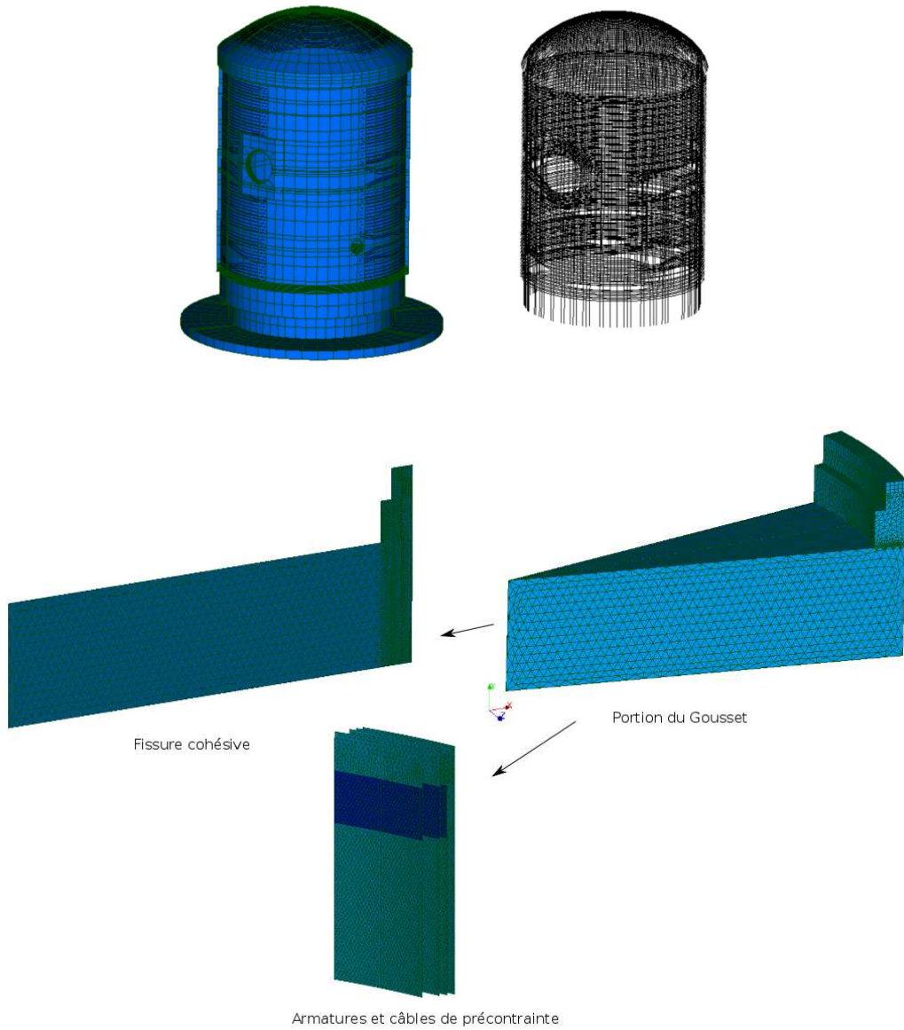
FIGURE 4.13 – Maillage de la portion de gousset
