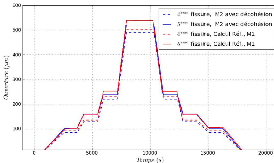
FIGURE 4.9 – Comparaison entre le calcul de référence et la méthode d'insertion de fissure avec prise en compte de la décohésion
