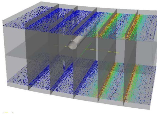
FIGURE 4.3 – Représentation de la décohésion le long des membranes pour le calcul de référence. On représente le glissement maximum le long de la membrane.
