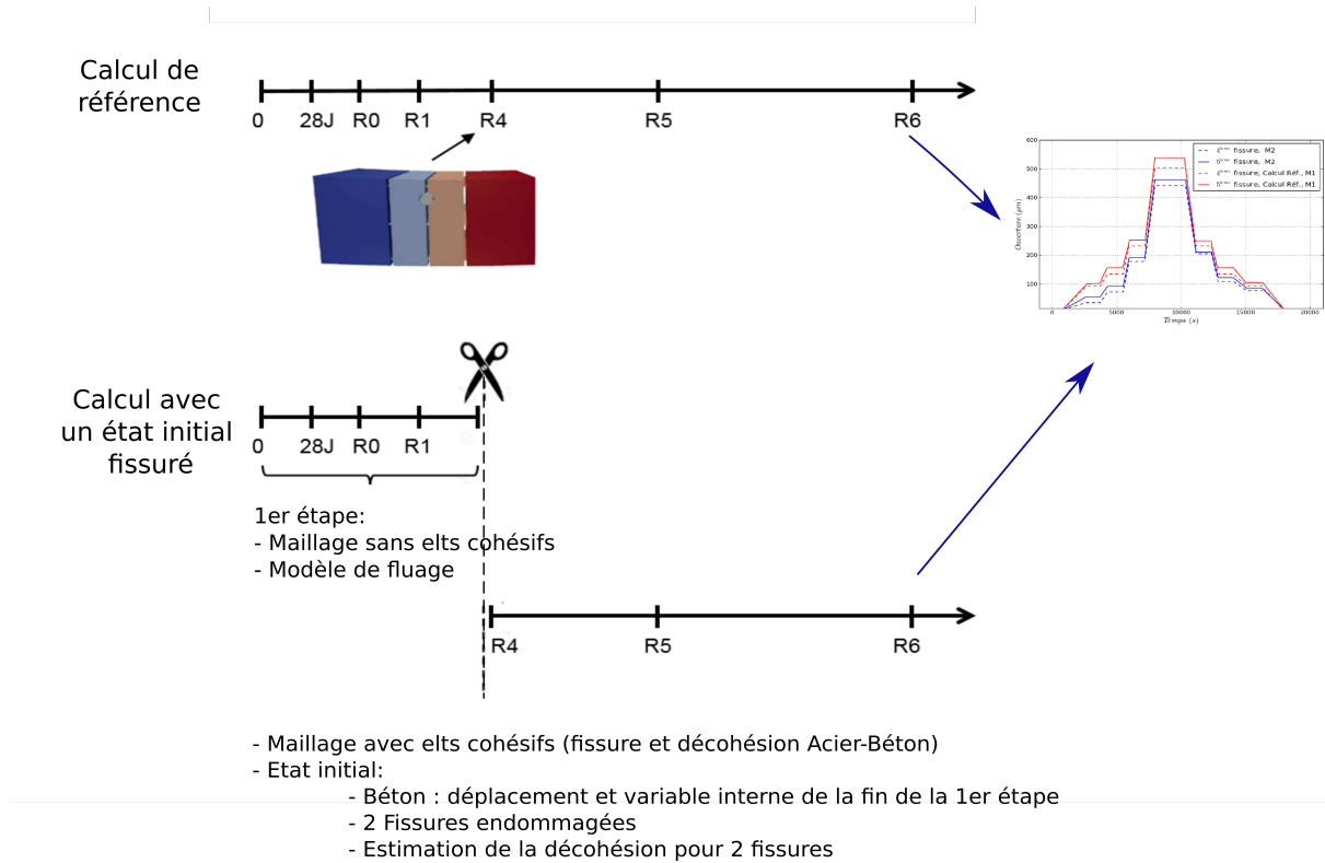
FIGURE 4.7 – Représentation des différentes étapes de modélisation de PACE1450
