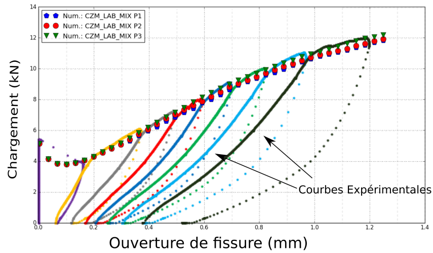
FIGURE 2.35 – Comparaison de la courbe Force-Ouverture obtenue expérimentalement (chargement cyclique) et numériquement (chargement monotone)
