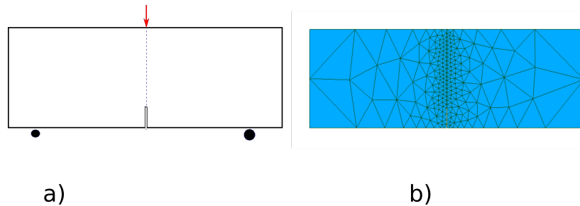
FIGURE 2.4 – Géométrie a) et Maillage b)
