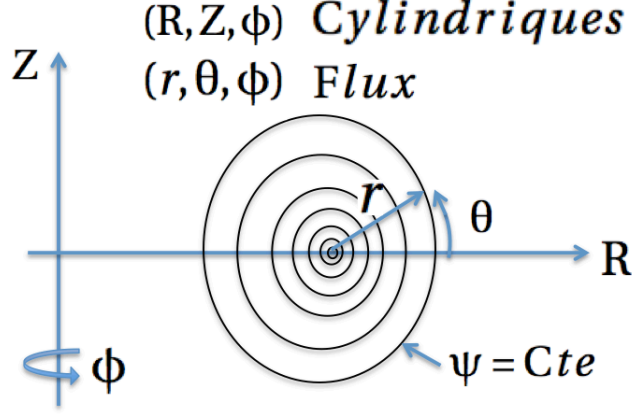
FIGURE 3.1 – Coordonnées cylindriques et alignées sur les surfaces de flux utilisées par XTOR-2F
