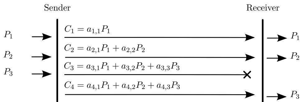
FIGURE 4 – Principe de Pipeline coding avec une taille de génération m = 3 et une combinaison redondante
