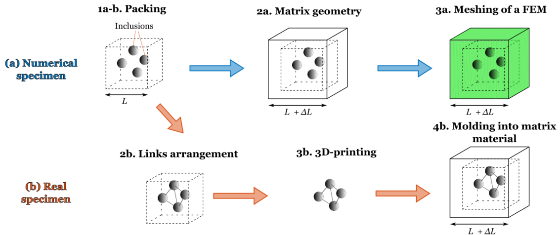
Figure 14: Représentation schématique du procédé de construction des échantillons numériques et réels.
