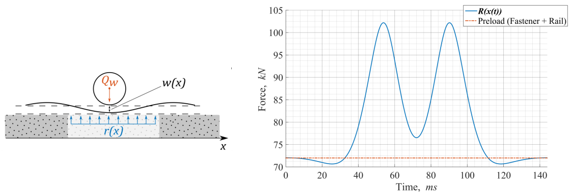
Figure 6: (a) Force de contre-réaction provoquée par la déflexion du rail ; (b) Profil Force-Temps final calculé pour la semelle
