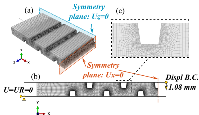
Figure 8: (a-b) Modèles géométriques 2D et 3D de la semelle; plans de symétrie ; (b) conditions aux limites appliquées ; (c) raffinement du maillage (rainures)
