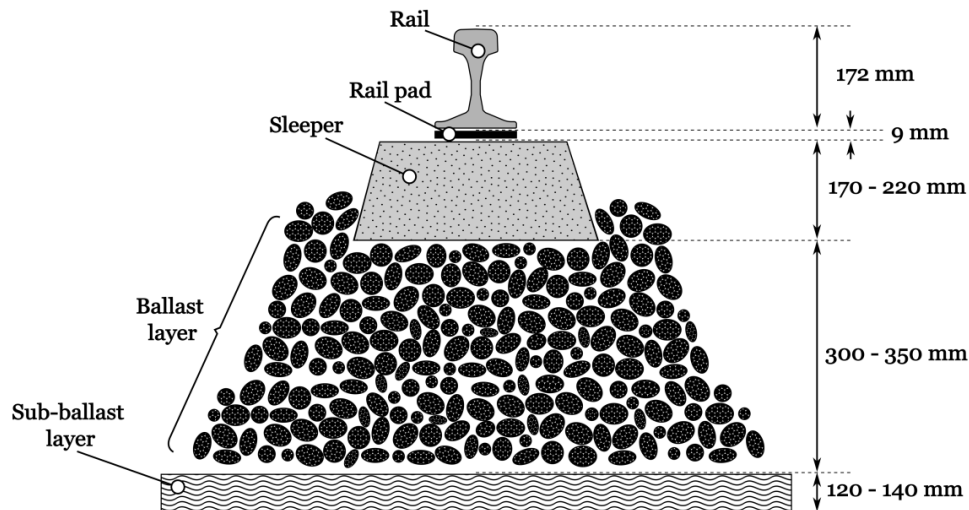
Figure 1: Coupe d'une structure de voie ferrée
