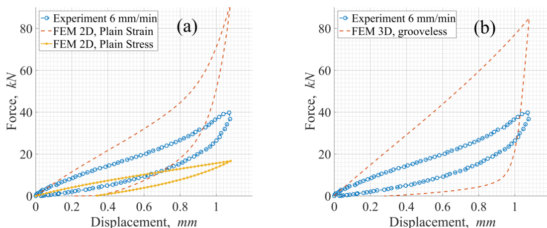
Figure 12: Comparaison entre les données expérimentales et la réponse du modèle FE de la semelle: (a) 2D en déformation plane et en contrainte plane; (b) 3D sans rainures FE
