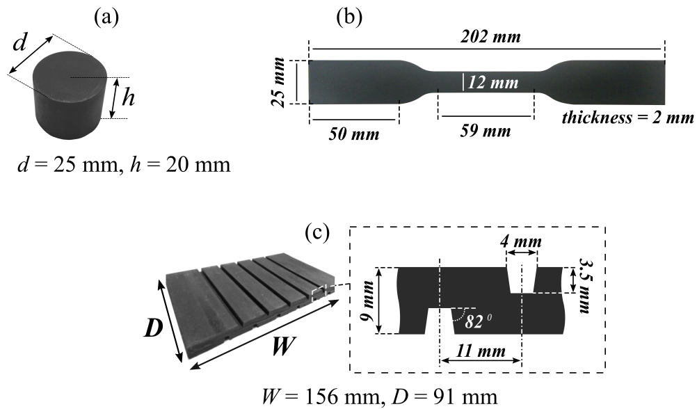
Figure 7: Dimensions des échantillons : (a) cylindrique; (b) haltère [112]; (c) demi-semelle de rail
