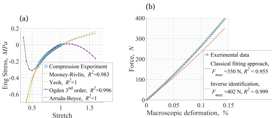
Figure 17: (a) Comparaison entre modèles hyper-élastiques et données expérimentales obtenues sur une éprouvette cylindrique en silicone testée en compression QS ; (b) le modelé d'Arruda-Boyce pour échantillon V00-D10 simulé par éléments finis
