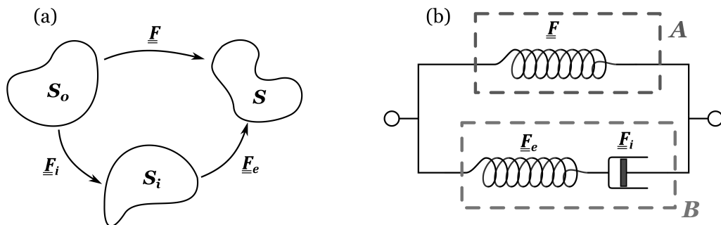
Figure 4: Représentation schématique de la division de la déformation dans l'approche du modèle-IV
