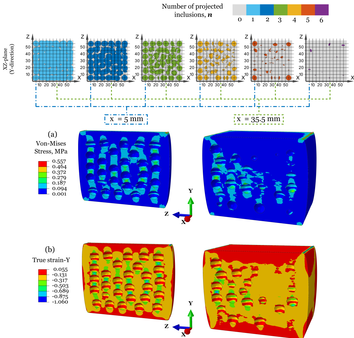
Figure 23: a-c: Échantillon Vo225Do8 sous 10 mm de compression : Contrainte de Von Mises (a) et déformation vraie YY (b) pour les sections à x = 5 \text{ mm} et x = 35,5 \text{ mm}
