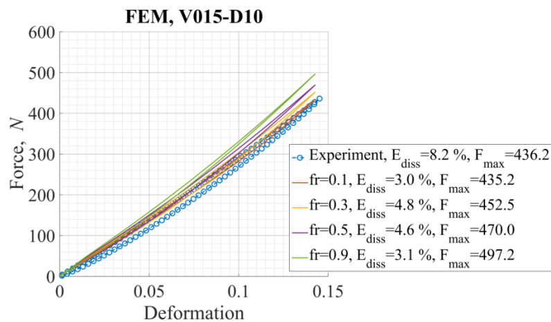
Figure 21: Influence du coefficient de frottement sur le comportement mécanique (échantillon V015-D10)
