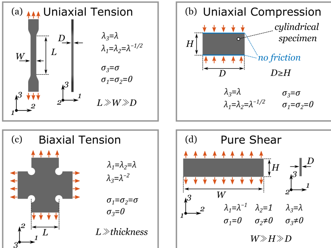
Figure 2: Essais typiques pour obtenir un état de déformation homogène pour un matériau incompressible : (a) traction uniaxiale, (b) compression uniaxiale, (c) traction biaxiale, (d) cisaillement pur [37].
