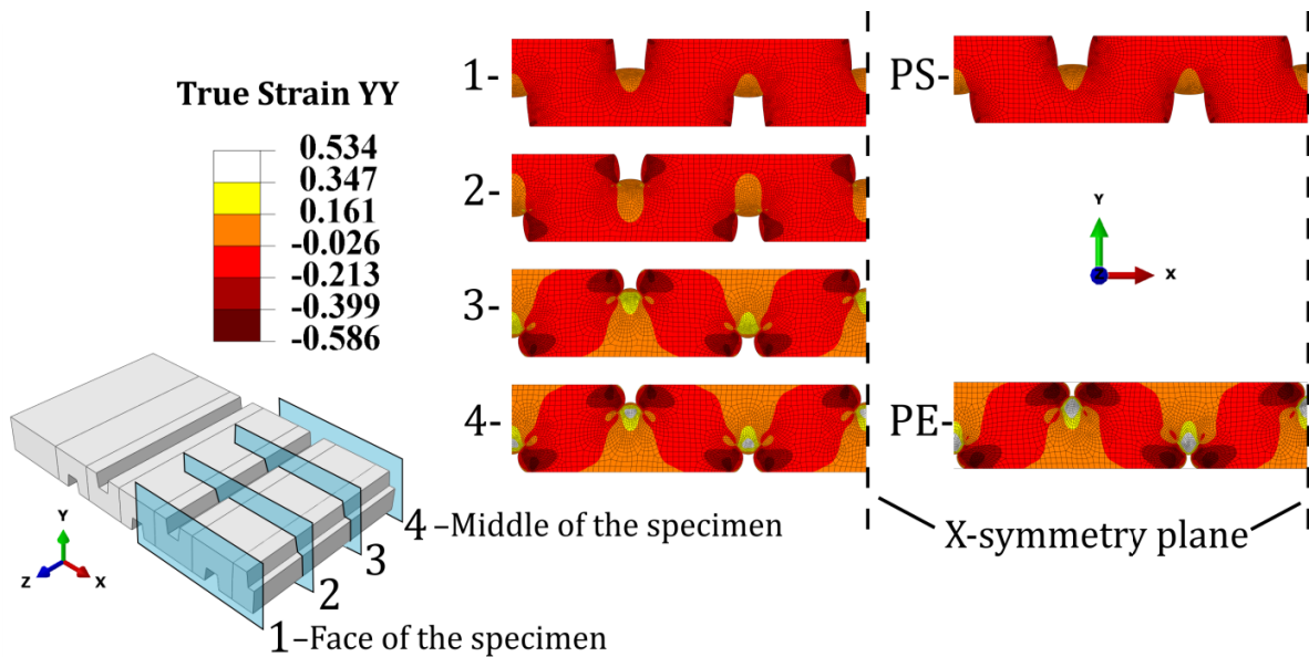
Figure 10: Déformations longitudinales (YY) pour différentes sections droites de normale Z (du bord libre au centre de la semelle) et champs de déformation obtenus en 2D (PE=déformations planes, PS= contraintes planes). L'écrasement de la semelle est de 1.08 mm.
