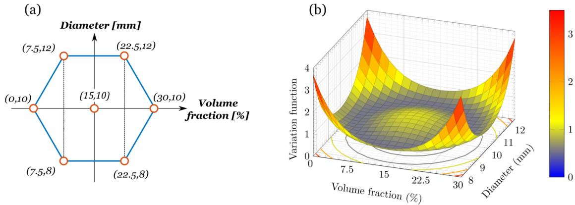
Figure 15: Caractéristiques des éprouvettes déduites du plan d'expériences de Doehlert (a) ; fonction variance (b)
