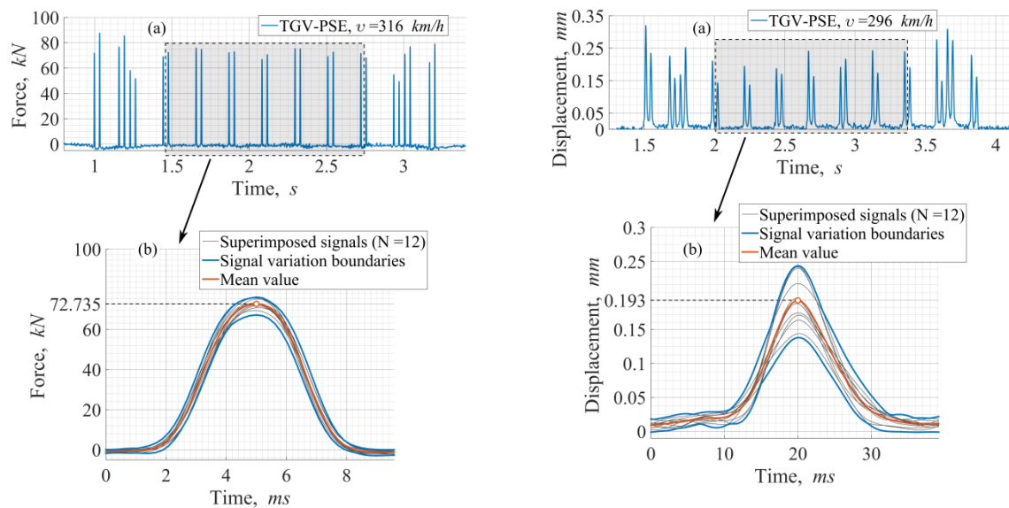
Figure 5: Passage d'un wagon de TGV-PSE : (a) charge de roue moyenne ; (b) enfoncement moyen de semelle
