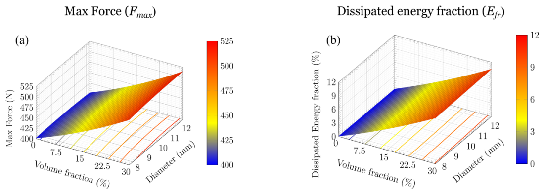
Figure 22: Surfaces de réponses construites à partir des résultats de simulation pour F_{max} (a) et E_{\%} (b) en fonction de la fraction volumique et du diamètre des inclusions
