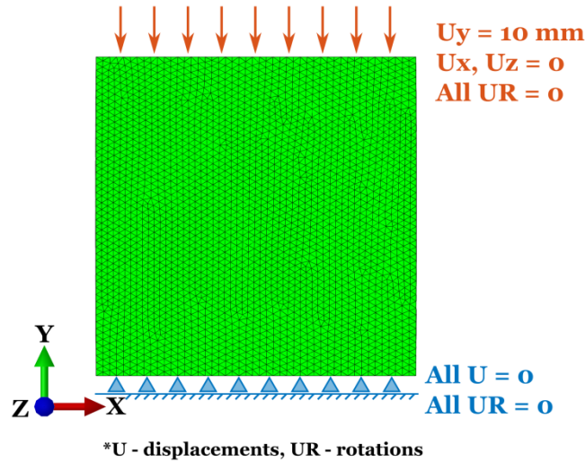
Figure 20: Conditions limites en déplacement appliquées sur les échantillons VM pour la simulation par EF
