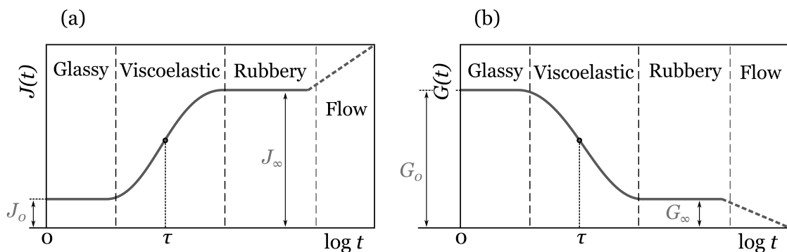
Figure 3: Module de fluage (a) et module de relaxation (b) en fonction du temps
