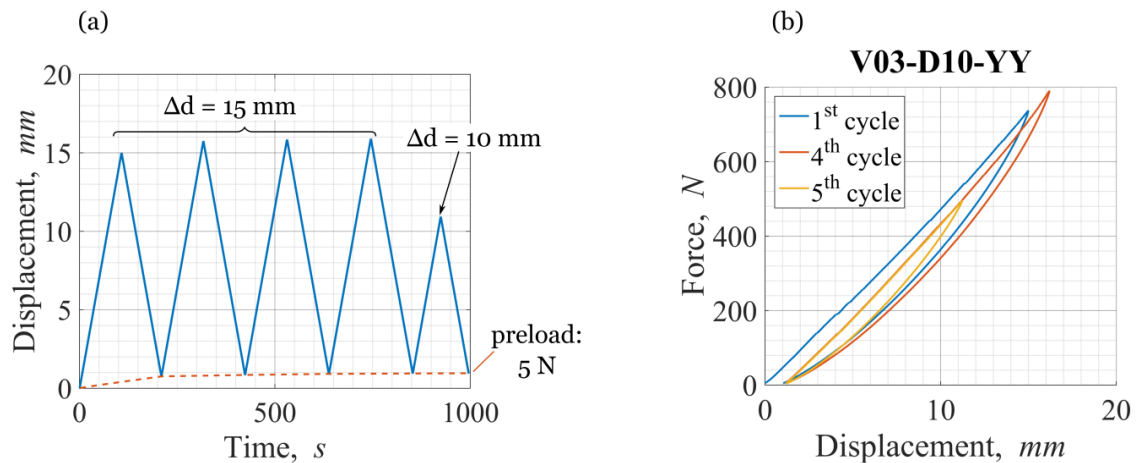
Figure 18: Programme de chargement d'un échantillon VM (a) et effet du pré-cyclage (b)
