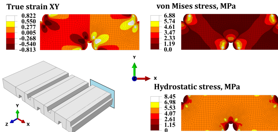
Figure 11: Champs de déformation vraie (transverses XY) et contraintes de Von Mises et hydrostatique calculés sur la section droite de la semelle. Déplacement : 1.08 mm
