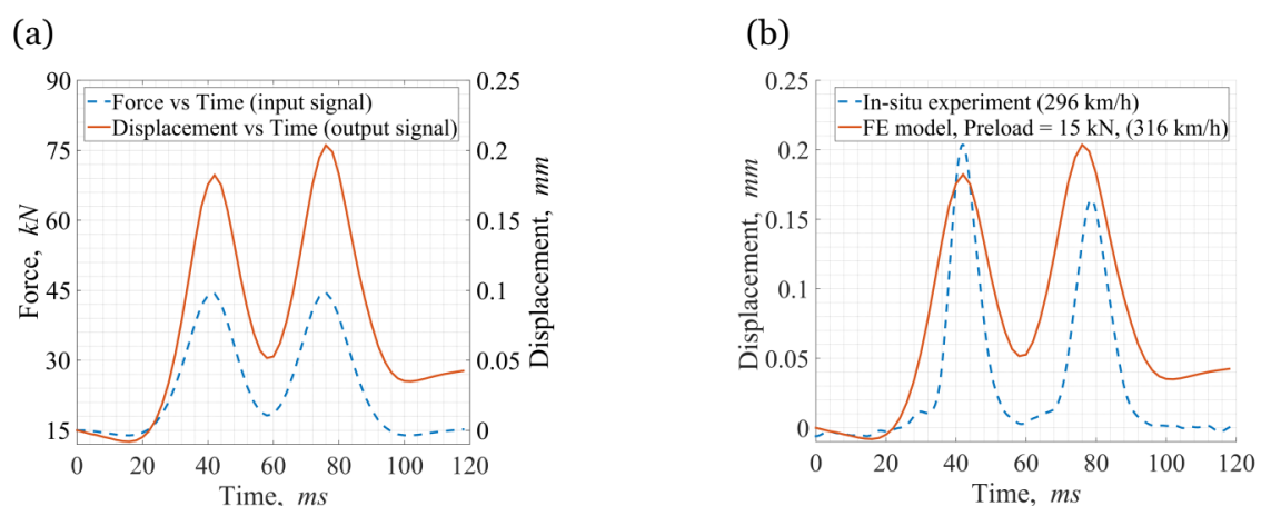
Figure 13: Chargement dynamique Force-Temps appliqué et réponse Déplacement-Temps récupérée de la simulation (a) ; comparaison des courbes Déplacement-Temps obtenues par simulation et par mesures in-situ (échelle de temps adimensionnée) (b).
