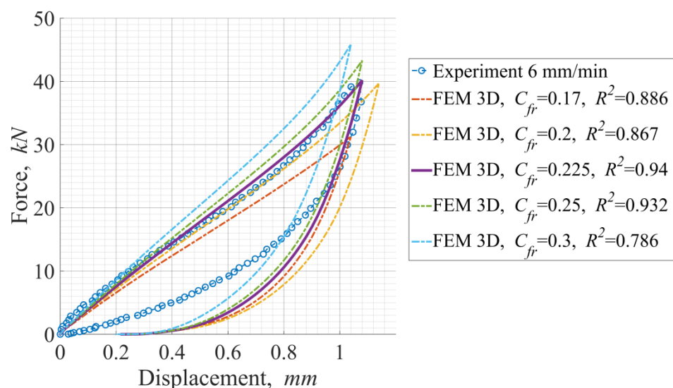
Figure 9: Courbes Force-Déplacement expérimentales et obtenues par simulation avec des coefficients de frottement compris entre 0.17 et 0.3
