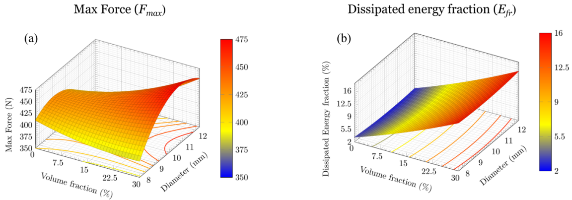
Figure 19: Surfaces de réponses expérimentales pour F_{max} (a) et E (b) en fonction de la fraction volumique et du diamètre des inclusions
