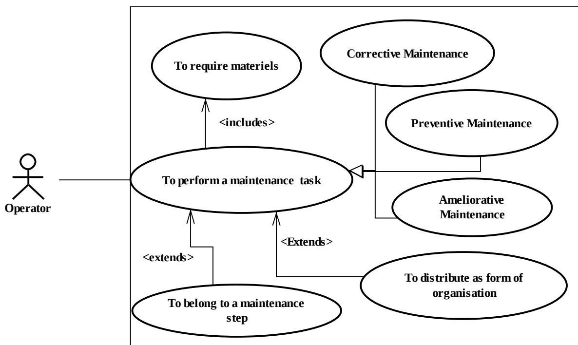
Figure IV. 7. Cas d'utilisation de l'identification du système.
