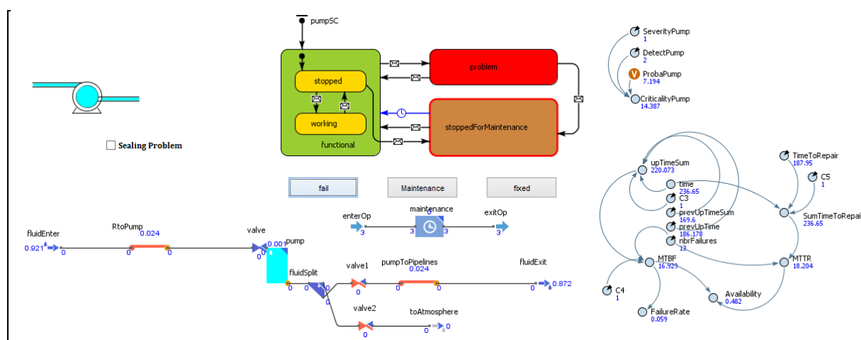
Figure VI. 13. Simulation de la pompe lors d'un arrêt.
