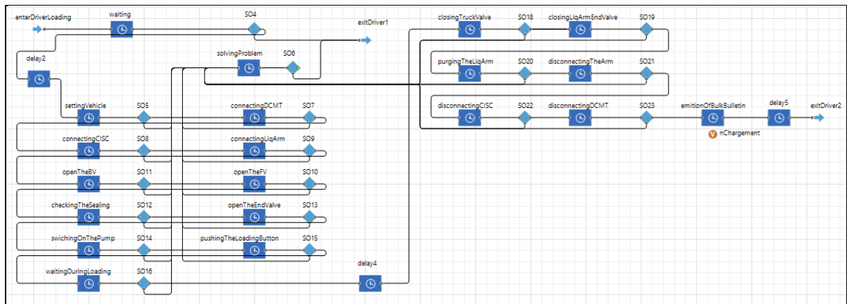
Figure VI. 9. Simulation des opérations de chargement par un actionChart.
