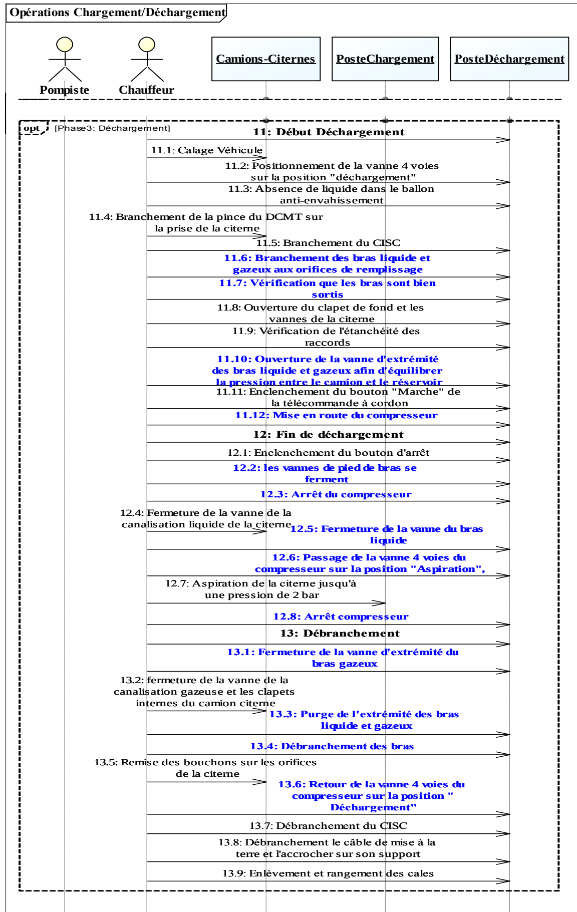
Figure II. 7. Diagramme de séquences des opérations de chargement/déchargement.
