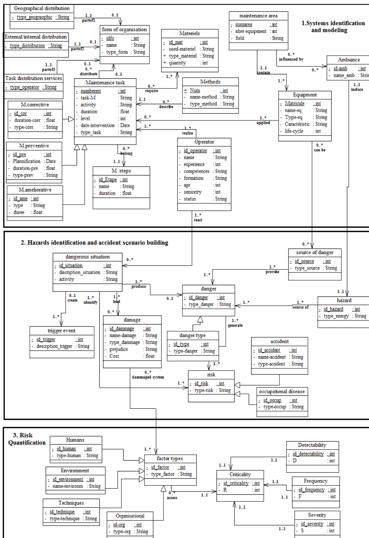
Figure IV. 5. Modèle MOSAR-UML pour l'Analyse des risques des activités de maintenance (Gallab et al. , 2017).
