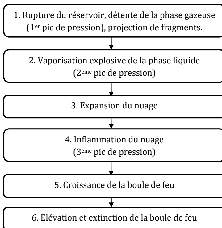
Figure II. 1. Les différentes étapes de la formation d'un BLEVE (Shield, 1993).
