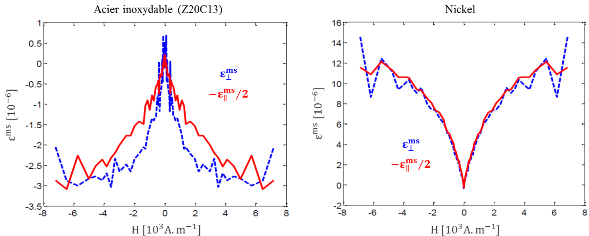
Figure 3.47 : Étude de l'hypothèse de magnétostriction isotrope et isochoire : comparaisons des déformations expérimentales de magnétostriction \epsilon_{\perp}^{ms} (bleu) et -\epsilon_{\parallel}^{ms}/2 (rouge) d'échantillons d'acier inoxydable Z20C13 (gauche) et de nickel (droite).
