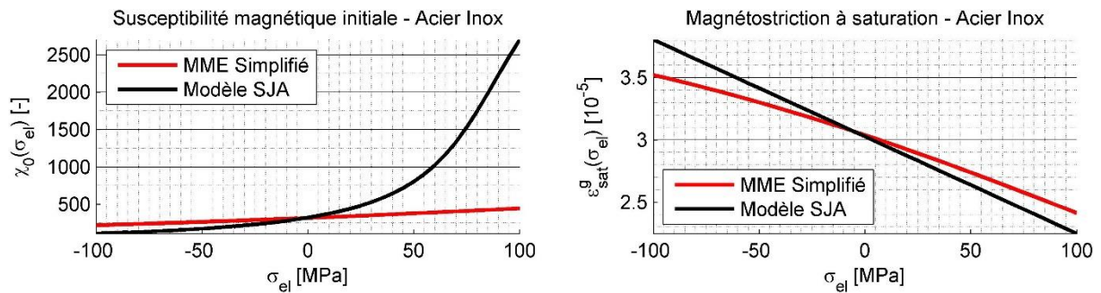
Figure 2.36 : Comparaisons des variations de la susceptibilité anhystérique initiale (gauche) et de la magnétostriction à saturation (droite) d'un acier inoxydable (AISI410) en fonction d'un niveau de contraintes mécaniques uni-axiales.
