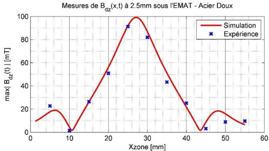
Figure 5.105 : Comparaison entre simulation et mesures des variations spatiales du maximum d'intensité de l'induction magnétique dynamique (normale) rayonnée à 2.5 mm dans l'entrefer entre l'EMAT et un échantillon d' acier doux .
