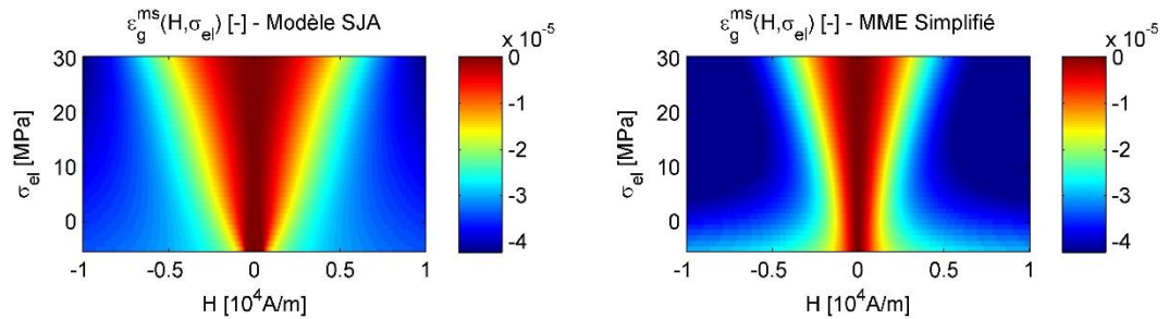
Figure 2.40 : Cartographies des courbes anhystériques de magnétostriction d'un nickel (recuit) en fonction du champ magnétique appliqué et d'une contrainte mécanique uni-axiale d'après le modèle SJA (gauche) et le MME simplifié (droite).
