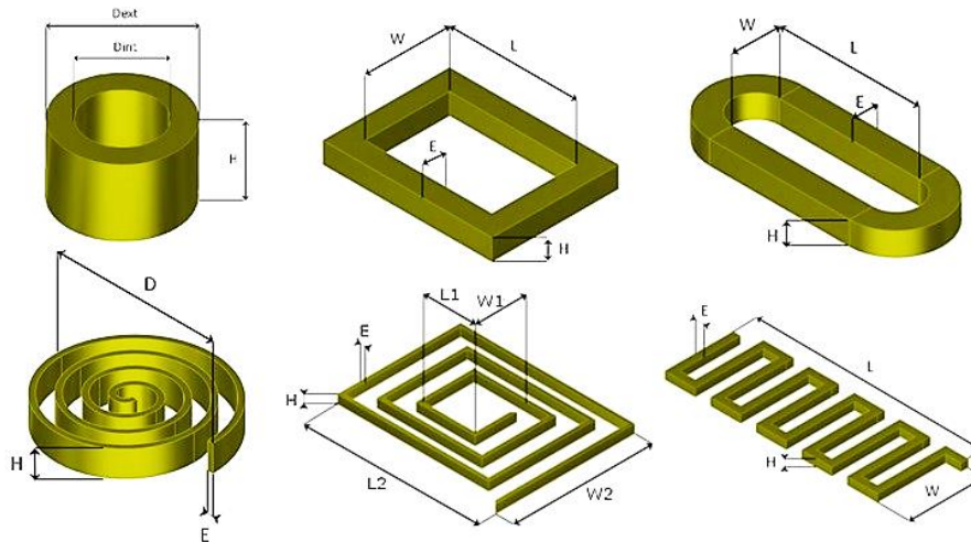
Figure 4.56 : Géométries de bobine inductrice disponibles dans le module CIVA CF.
