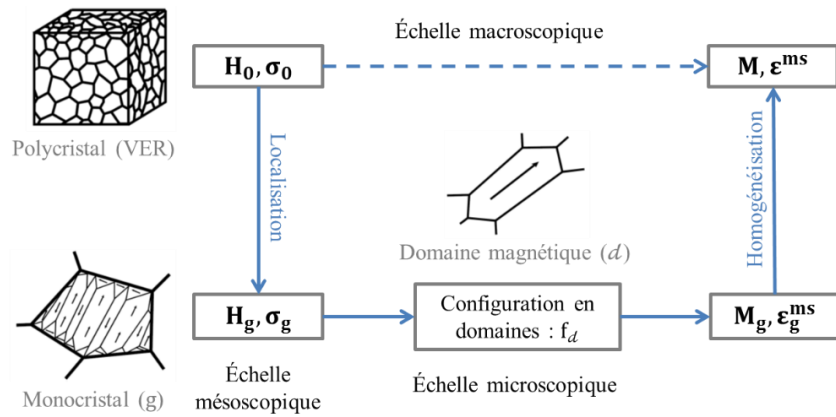
Figure 2.28 : Stratégie de modélisation multi-échelle du comportement magnéto-élastique de milieux ferromagnétiques polycristallins. Figure inspirée de [Bartok-et-al_2011].
