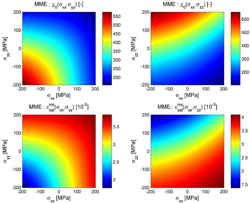
Figure 2.42 : Influence des contraintes bi-axiales (\sigma_{xx}, \sigma_{yy}, 0) (gauche) et (\sigma_{xx}, 0, \sigma_{zz}) (droite) sur la susceptibilité anhystérique initiale (haut) et la magnétostriction à saturation (bas) d'un échantillon d' acier inoxydable (AISI 410) .
