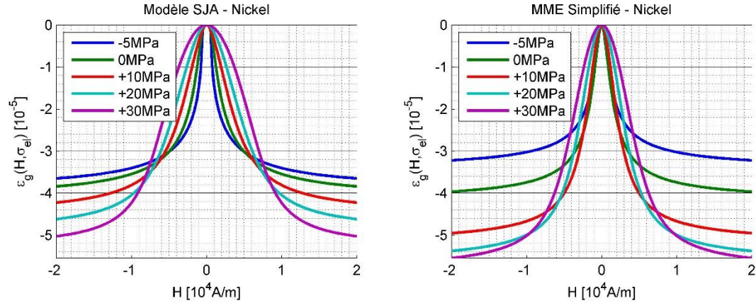
Figure 2.39 : Courbes anhystériques de magnétostriction d'un nickel (recuit) en fonction du champ magnétique appliqué et d'une contrainte mécanique uni-axiale d'après le modèle SJA (gauche) et le MME simplifié (droite).
