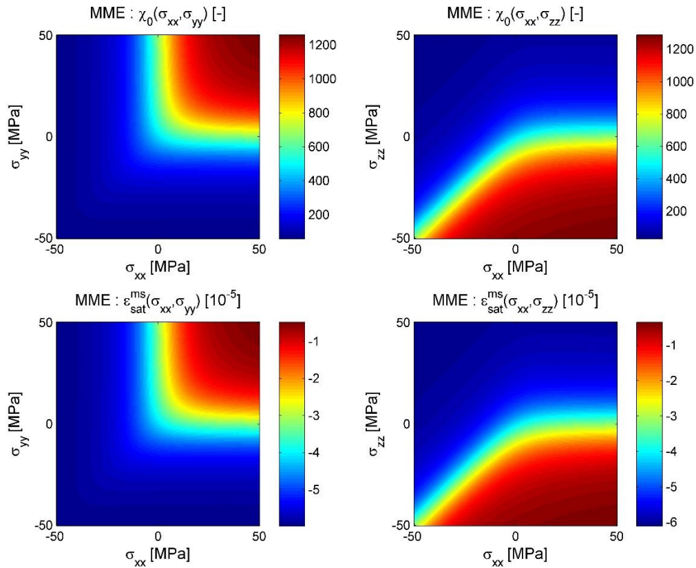
Figure 2.43 : Influence des contraintes bi-axiales (\sigma_{xx}, \sigma_{yy}, 0) (gauche) et (\sigma_{xx}, 0, \sigma_{zz}) (droite) sur la susceptibilité anhystérique initiale (haut) et la magnétostriction à saturation (bas) d'un échantillon de nickel (recuit) .
