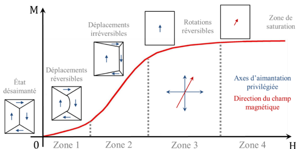
Figure 1.11 : Courbe de première aimantation et réarrangement de la structure microscopique en domaines de Weiss en fonction de l'intensité de l'excitation magnétique extérieure
