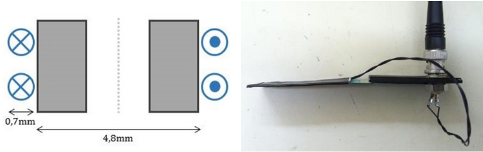
Figure 5.100 : Schéma (gauche) et photo (droite) du capteur de flux magnétique fabriqué au CETIM.
