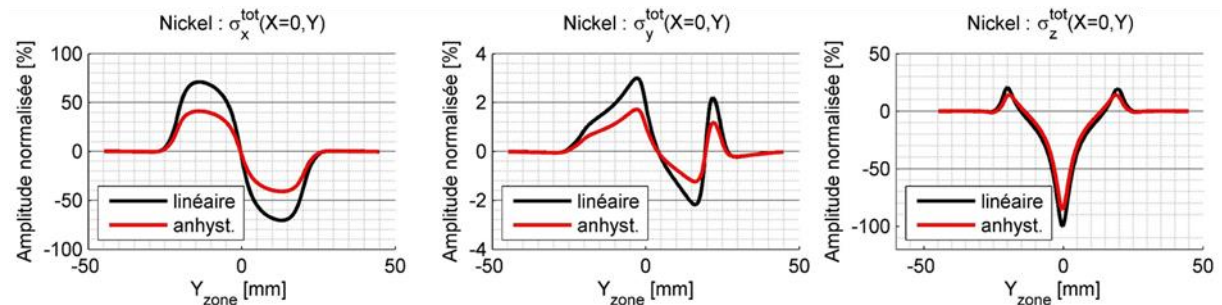
Figure 4.86 : Variations selon Y_{zone} des composantes \sigma_x^{tot} (gauche), \sigma_y^{tot} (centre), \sigma_z^{tot} (droite) des sources totales de transduction induites par EMAT pour un nickel recuit supposé linéaire (noir) ou anhystérétique (rouge).
