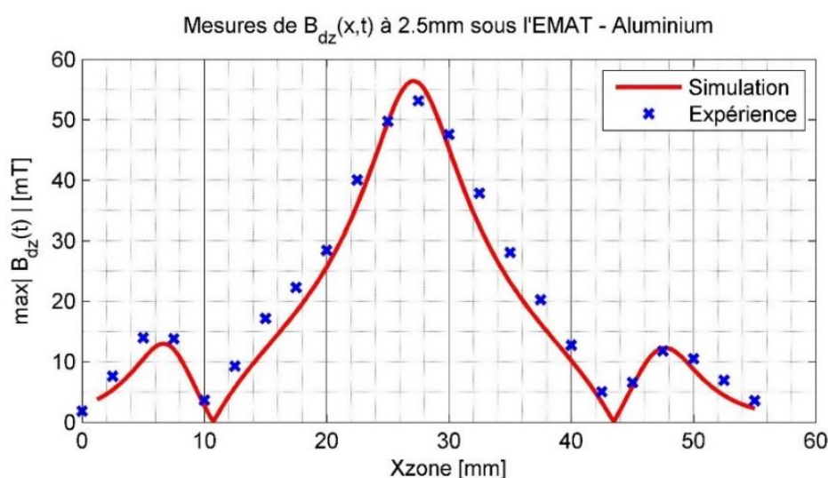
Figure 5.104 : Comparaison entre simulation et mesures des variations spatiales du maximum d'intensité de l'induction magnétique dynamique (normale) rayonnée à 2.5 mm dans l'entrefer entre l'EMAT et un échantillon d' aluminium .
