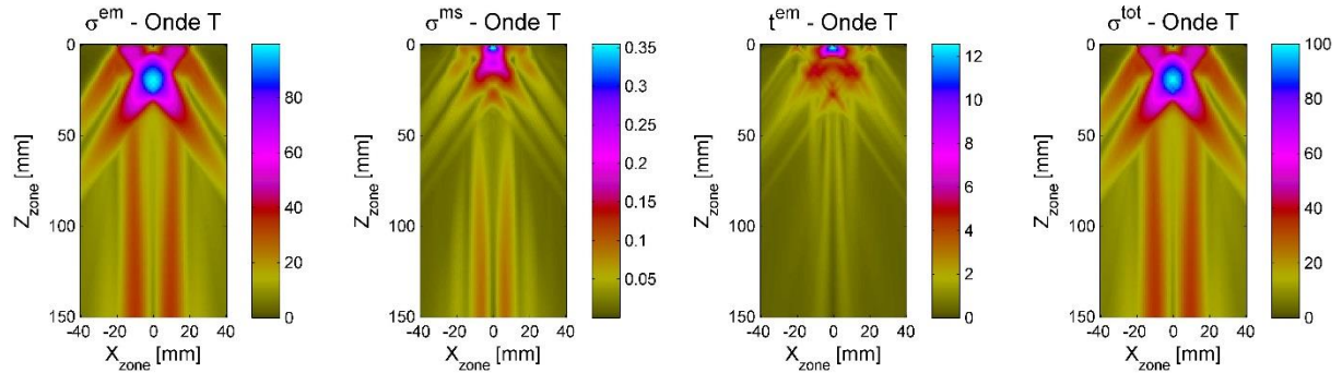
Figure 4.67 : Cartographies dans le plan (X, Z) du maximum d'amplitude ultrasonore en onde T rayonnée par EMAT dans un échantillon d' acier inoxydable Z20C13 . Les sources de rayonnement sont de gauche à droite : \tilde{\sigma}^{em} , \tilde{\sigma}^{ms} , t^{em} , et \sigma^{tot} .
