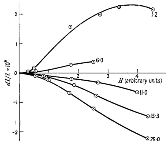
Figure 1.15 : Magnétostriction du fer soumis à différents chargements mécaniques [Lee_1955].
