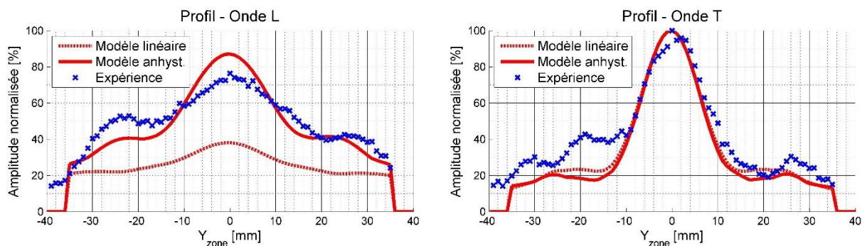
Figure 5.118 : Profils des maxima d'amplitude en ondes L (gauche) et T (droite) induits par EMAT sur un diamètre du cylindre d'acier inoxydable. Trait pointillé : modèle linéaire ; Trait plein : modèle anhystérique ; Croix : expérience.
