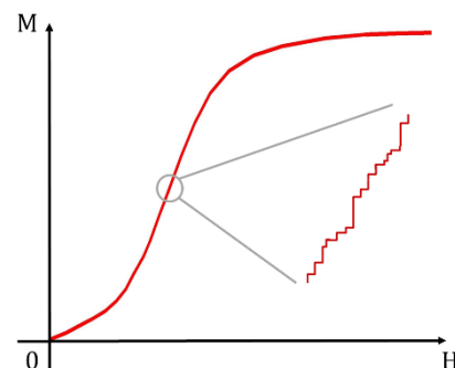
Figure 1.12 : Illustration du bruit ferromagnétique de Barkhausen
