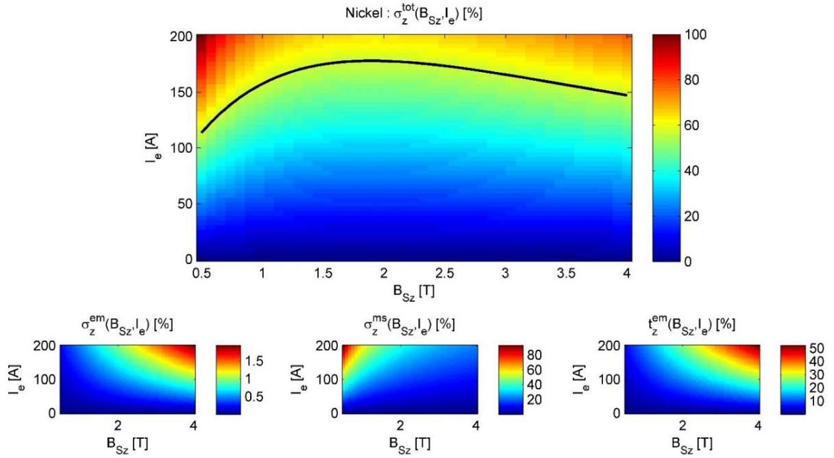
Figure 4.79 : Variations d'amplitude maximale de la source normale totale \sigma_z^{\text{tot}} (haut), composée des sources \tilde{\sigma}_z^{\text{em}} (gauche), \tilde{\sigma}_z^{\text{ms}} (centre), t_z^{\text{em}} (droite), induites par EMAT sur une pièce de nickel recuit selon les paramètres d'excitation ( I_e , B_s ). La courbe noire trace l'iso-amplitude des sources normales totales définies à partir des paramètres (175 A, 1.5 T).
