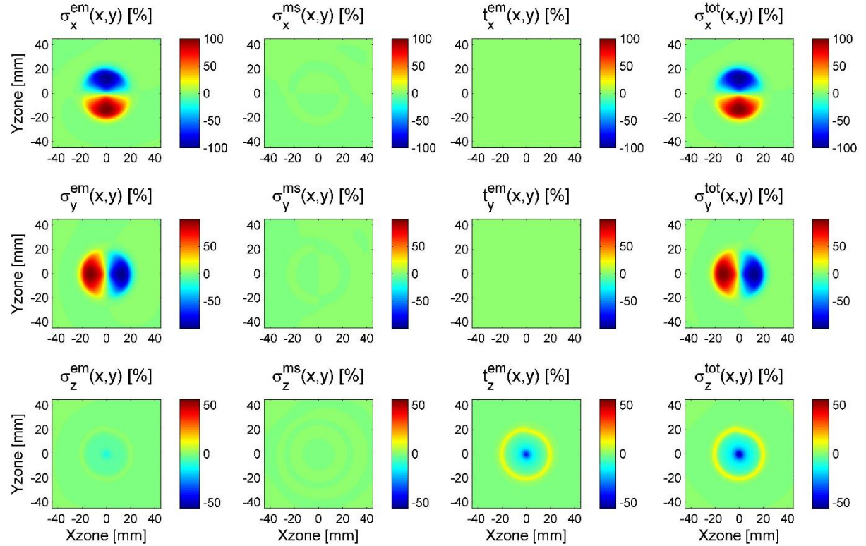
Figure 4.61 : Variations spatiales des sources de transduction ultrasonore induites par EMAT en acier inoxydable Z20C13 .
