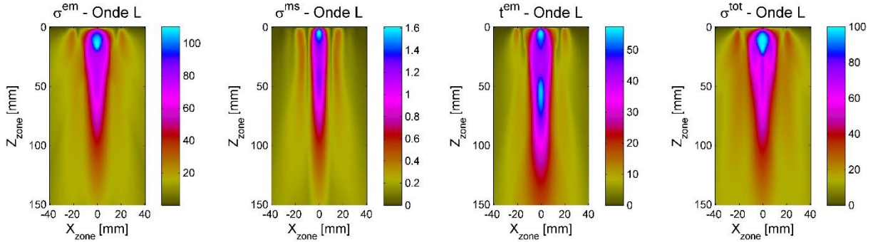
Figure 4.71 : Cartographies dans le plan (X, Z) du maximum d'amplitude ultrasonore en onde L rayonnée par EMAT dans une pièce d' acier inoxydable Z20C13 . Les sources de rayonnement sont de gauche à droite : \tilde{\sigma}^{em} , \tilde{\sigma}^{ms} , t^{em} , et \sigma^{tot} .
