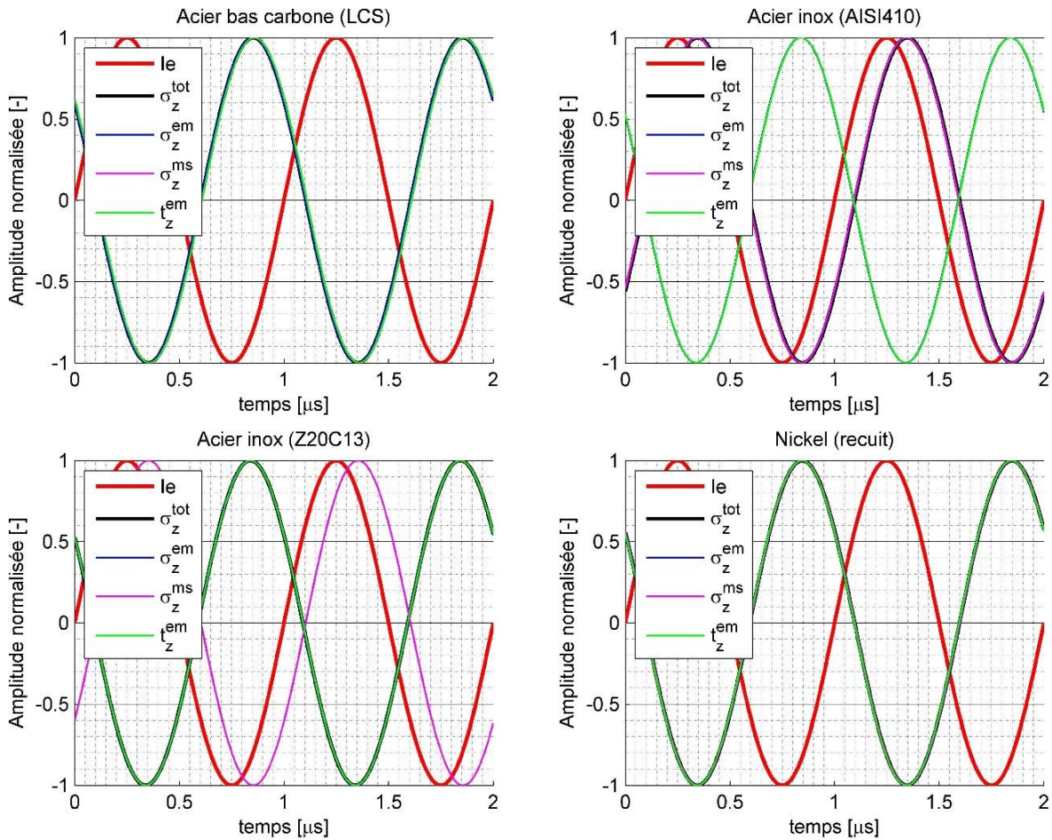
Figure 4.64 : Variations temporelles des sources de transduction induites par EMAT dans de l'acier bas carbone (haut à gauche), des aciers inoxydables AISI 410 (haut à droite) et Z20C13 (bas à gauche), et du nickel recuit (bas à droite).
