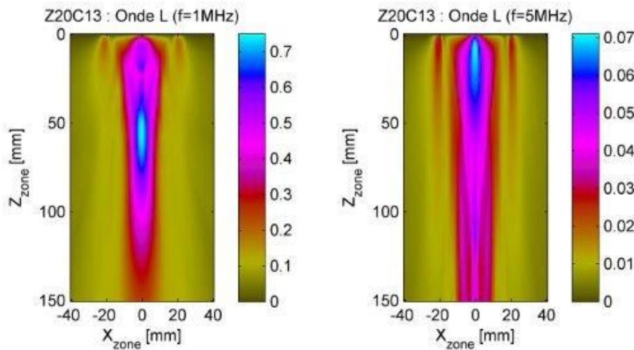
Figure 5.115 : Simulation du champ ultrasonore rayonné par l'EMAT excité à 1 MHz (gauche) et à 5 MHz (droite) dans un échantillon cylindrique d'acier inoxydable Z20C13) à partir du modèle de transduction développé dans cette étude.
