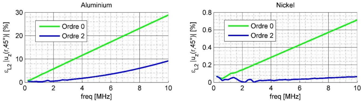
Figure 3.54 : Évolution de l'erreur L^2 des approximations |u_z^{(2)}| (courbe bleue), et |u_z^{(0)}| (courbe verte) par rapport à l'intégrale volumique |u_z^{(vol)}| en fonction de la fréquence d'inspection et du milieu inspecté.
