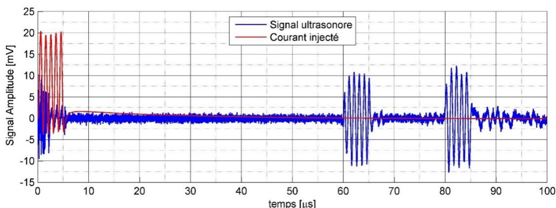
Figure 5.110 : Mesure par un traducteur piézoélectrique focalisé en immersion du champ ultrasonore transmis par EMAT dans une pièce d'acier inoxydable Z20C13 pour une intensité de courant électrique de 2.42A.
