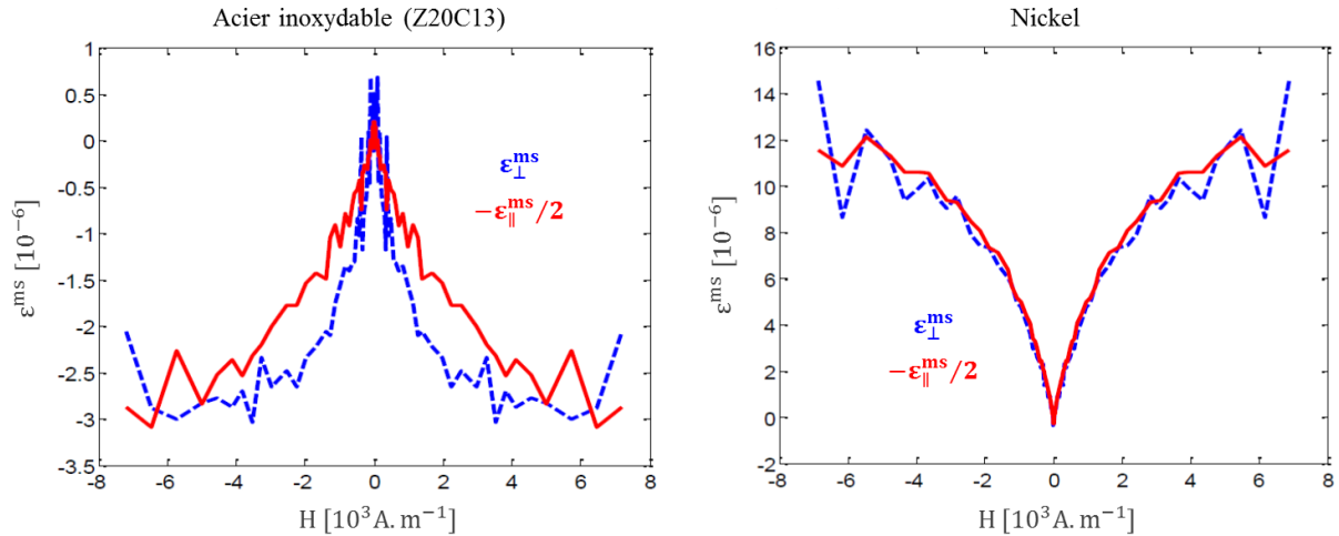
Figure 3.47 : Étude de l'hypothèse de magnétostriction isotrope et isochore : comparaisons des déformations expérimentales de magnétostriction \epsilon_{\perp}^{ms} (bleu) et -\epsilon_{\parallel}^{ms}/2 (rouge) d'échantillons d'acier inoxydable Z20C13 (gauche) et de nickel (droite).
