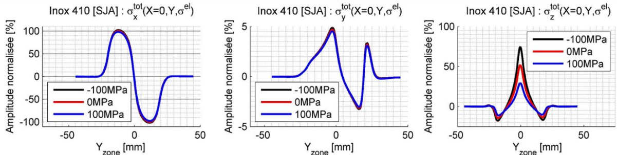
Figure 4.88 : Influence des contraintes mécaniques uni-axiales sur les variations spatiales des composantes \sigma_x^{tot} (gauche), \sigma_y^{tot} (centre) et \sigma_z^{tot} (droite) de sources induites par EMAT à la surface d'un acier inoxydable AISI 410 selon le modèle SJA .
