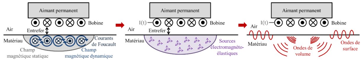
Figure 0.1 : Principe de fonctionnement d'un EMAT.
