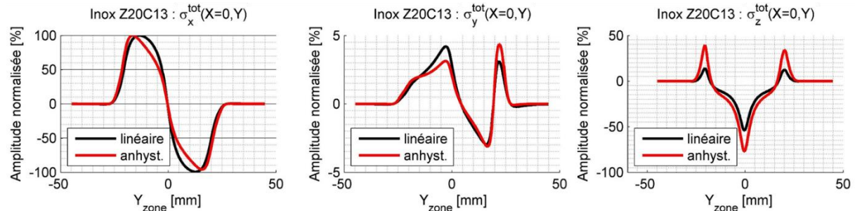
Figure 4.85 : Variations selon Y_{zone} des composantes \sigma_x^{tot} (gauche), \sigma_y^{tot} (centre), \sigma_z^{tot} (droite) des sources totales de transduction induites par EMAT pour un acier inoxydable Z20C13 supposé linéaire (noir) ou anhystérétique (rouge).
