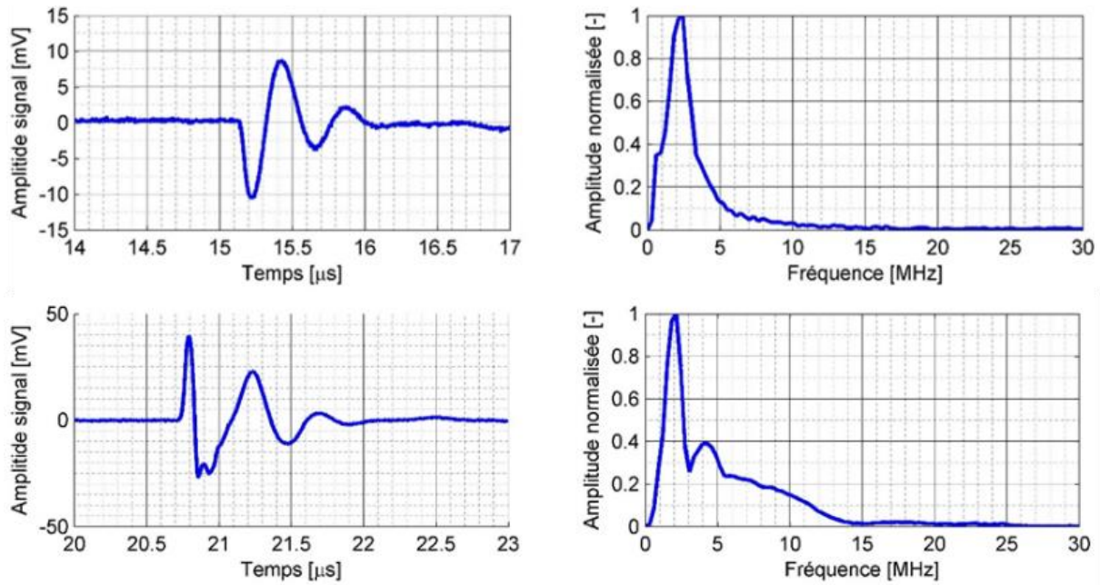
Figure 5.121 : Mesures par un capteur piézoélectrique plan du signal en ondes L (gauche), et du spectre associé (droite), transmis par un EMAT excité d'un courant de forte intensité dans des pièces d'aluminium (haut) et d'acier doux (bas).
