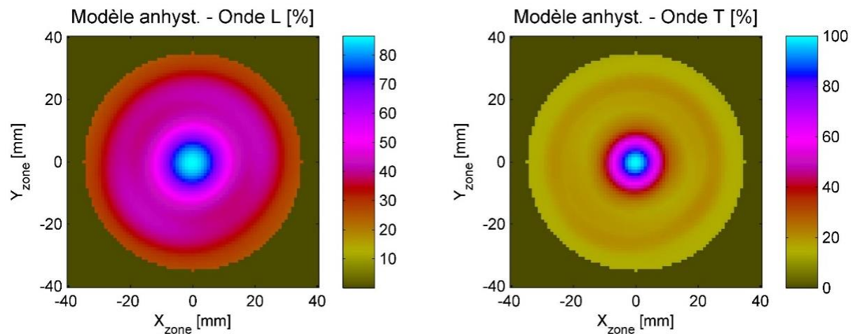
Figure 5.117 : C-scans simulés du champ ultrasonore rayonné en ondes longitudinales (gauche) et transversales (droite) par EMAT sur le fond d'un cylindre d'acier inoxydable Z20C13.
