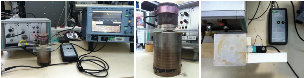
Figure 5.101 : Montage expérimental de la mesure de flux magnétique dynamique rayonné dans l'entrefer (visible au centre) par l'EMAT didactique placé sur un bloc d'acier doux (gauche et centre) et sur un bloc d'aluminium (droite).
