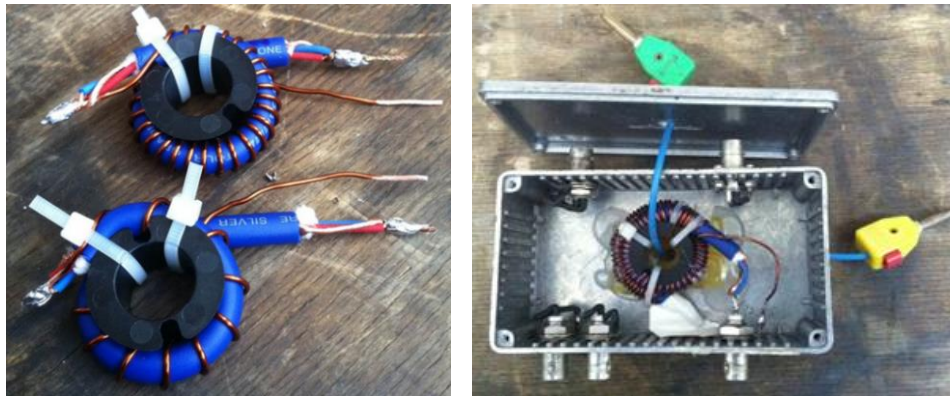
Figure 5.96 : Sondes de Rogowski fabriquées au CETIM avec différents enroulements secondaires.
