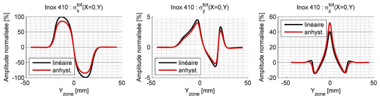
Figure 4.84 : Variations selon Y_{zone} des composantes \sigma_x^{tot} (gauche), \sigma_y^{tot} (centre), \sigma_z^{tot} (droite) des sources totales de transduction induites par EMAT pour un acier inoxydable AISI 410 supposé linéaire (noir) ou anhystérétique (rouge).
