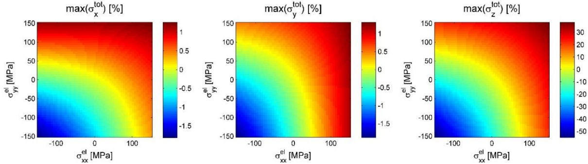
Figure 4.91 : Cartographie des variations d'amplitude maximale des composantes \sigma_x^{tot} (gauche), \sigma_y^{tot} (centre) et \sigma_z^{tot} (droite) de sources induites par EMAT à la surface d'un acier inoxydable AISI 410 en fonction de contraintes bi-axiales ( \sigma_{xx}^{el} , \sigma_{yy}^{el} ).
