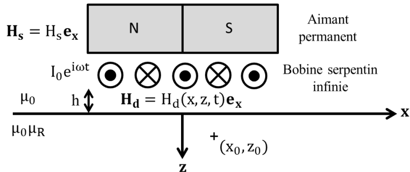
Figure 3.49 : Configuration EMAT élémentaire 2D de Thompson.
