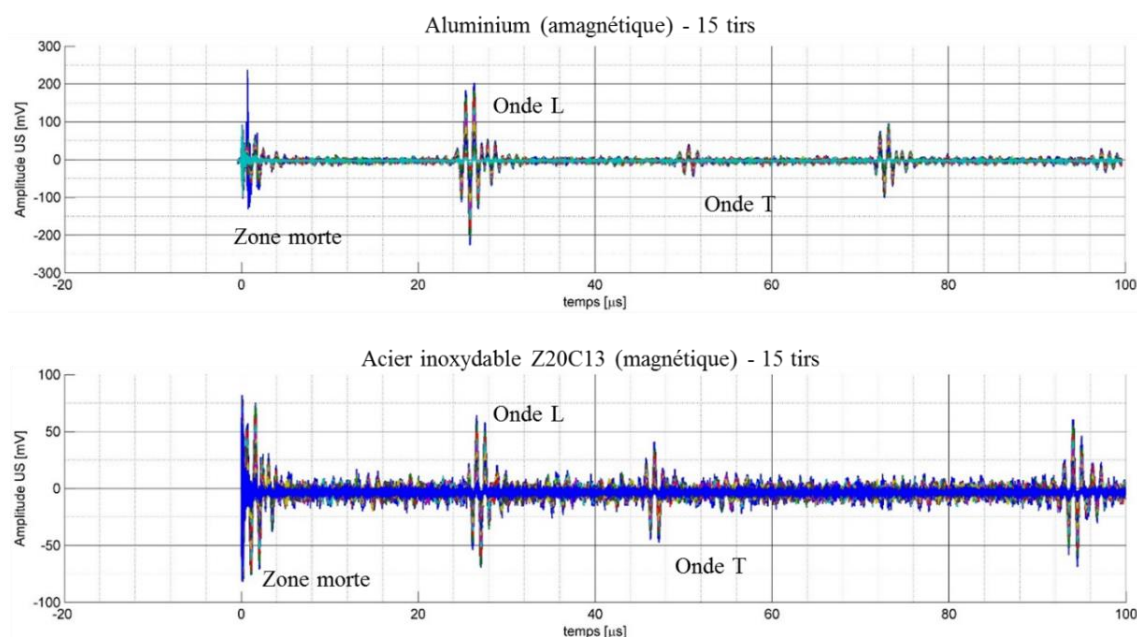
Figure 5.107 : Mesure par un transducteur piézoélectrique plan au contact du champ ultrasonore transmis par EMAT dans des pièces d'aluminium (haut) et d'acier inoxydable Z20C13 (bas) en fonction de l'intensité du courant d'excitation.
