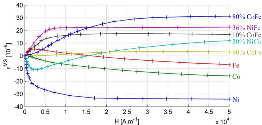
Figure 1.18 : Déformations de magnétostriction en fonction de l'excitation magnétique du fer, du nickel, du cobalt, et de quelques-uns de leurs alliages, adaptées de [Lee_1955] et [Bozorth_1964]
