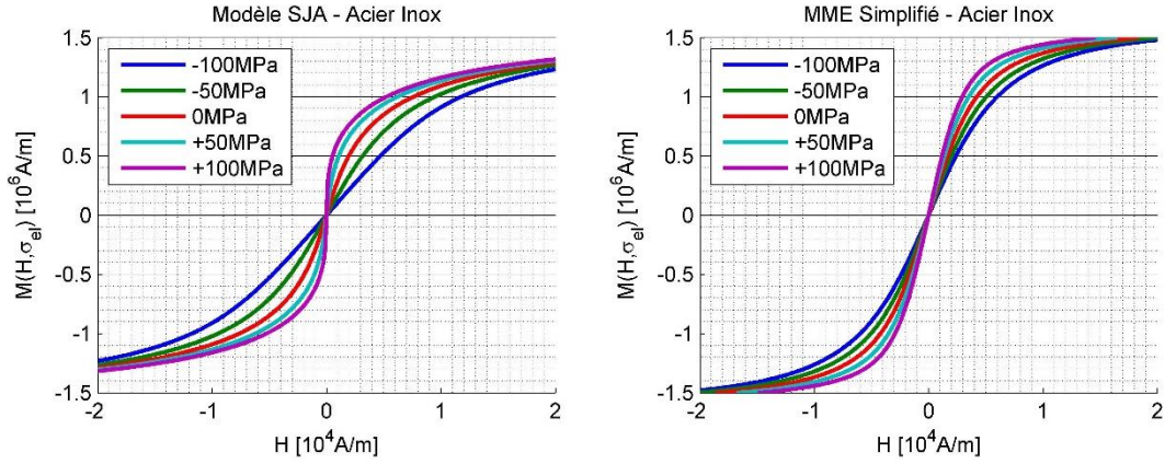
Figure 2.32 : Courbes anhystériques d'aimantation d'un acier inoxydable (AISI410) en fonction du champ magnétique appliqué et d'une contrainte mécanique uni-axiale d'après le modèle SJA (gauche) et le MME simplifié (droite).
