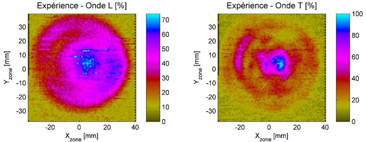
Figure 5.116 : C-scans mesurés du champ ultrasonore rayonné en ondes longitudinales (gauche) et transversales (droite) par EMAT sur le fond d'une pièce cylindrique d'acier inoxydable Z20C13.
