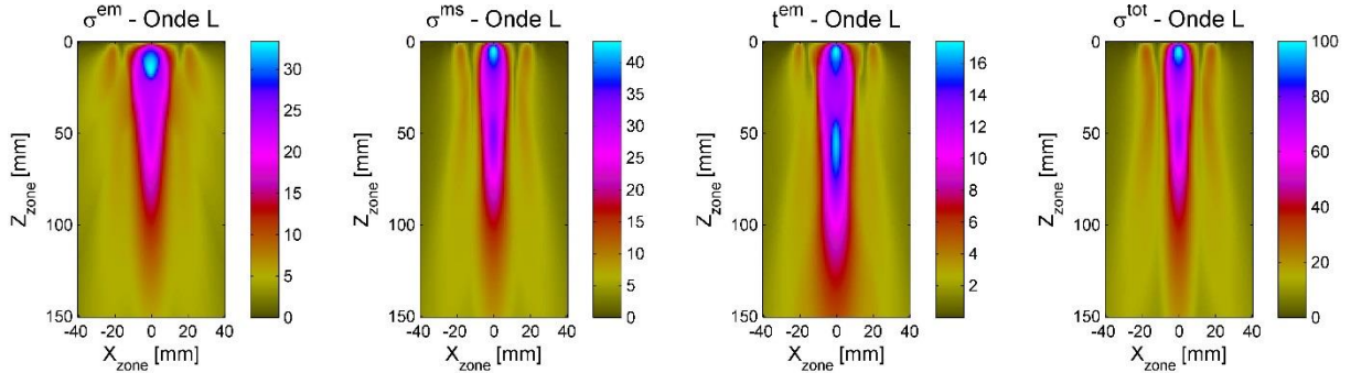
Figure 4.72 : Cartographies dans le plan (X, Z) du maximum d'amplitude ultrasonore en onde L rayonnée par EMAT dans une pièce d' acier inoxydable AISI410 . Les sources de rayonnement sont de gauche à droite : \tilde{\sigma}^{em} , \tilde{\sigma}^{ms} , t^{em} , et \sigma^{tot} .
