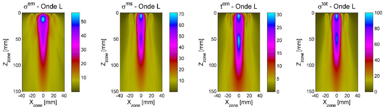
Figure 4.73 : Cartographies dans le plan (X, Z) du maximum d'amplitude ultrasonore en onde L rayonnée par EMAT dans une pièce de nickel recuit . Les sources de rayonnement sont de gauche à droite : \tilde{\sigma}^{em} , \tilde{\sigma}^{ms} , t^{em} , et \sigma^{tot} .
