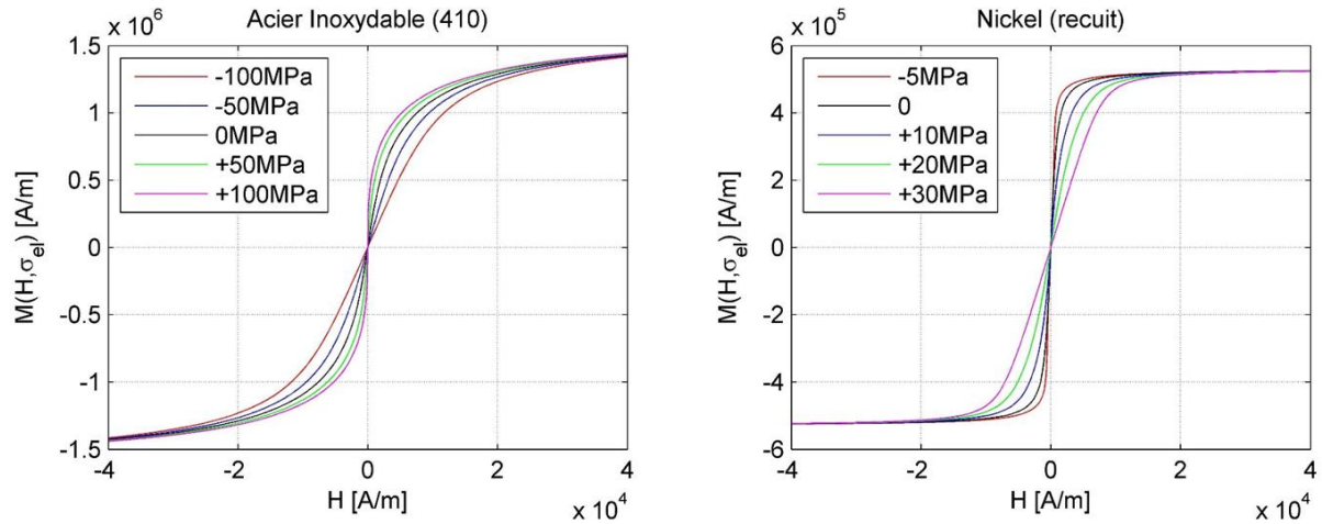
Figure 2.25 : Courbes anhystériques d'aimantation d'échantillons d'acier inoxydable (gauche) et de nickel (droite) en fonction du champ magnétique appliqué et d'une contrainte mécanique uni-axiale d'après le modèle SJA.
