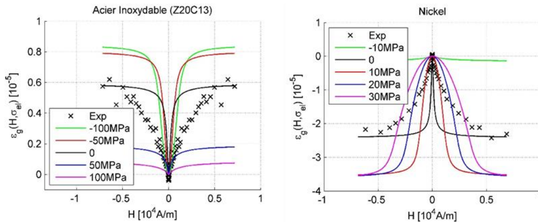
Figure 2.30 : Courbes anhystérétiques de magnétostriction d'un acier inoxydable (gauche) et du nickel (droite) en fonction du champ magnétique appliqué et d'une contrainte mécanique uni-axiale d'après le MME simplifié.
