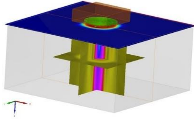
Figure 4.57 : Simulation des ondes volumiques ultrasonores rayonnées par une source surfacique EMAT dans CIVA US.
