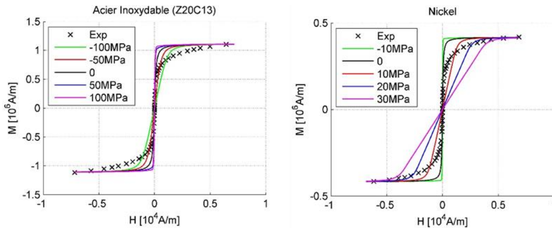
Figure 2.29 : Courbes anhystérétiques d'aimantation d'un acier inoxydable (gauche) et du nickel (droite) en fonction du champ magnétique appliqué et d'une contrainte mécanique uni-axiale d'après le MME simplifié.
