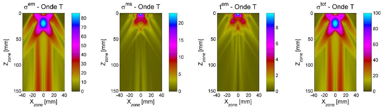
Figure 4.69 : Cartographies dans le plan (X, Z) du maximum d'amplitude ultrasonore en onde T rayonnée par EMAT dans un échantillon de nickel recuit . Les sources de rayonnement sont de gauche à droite : \tilde{\sigma}^{em} , \tilde{\sigma}^{ms} , t^{em} , et \sigma^{tot} .
