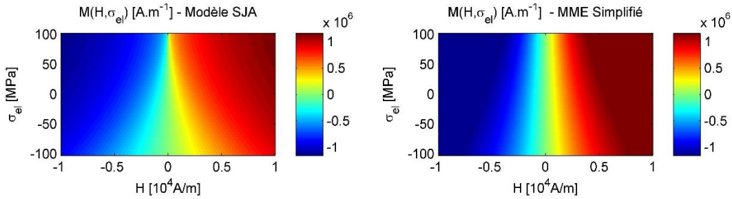
Figure 2.33 : Cartographies des courbes anhystériques d'aimantation d'un acier inoxydable (AISI410) en fonction du champ magnétique et d'une contrainte mécanique uni-axiale d'après le modèle SJA (gauche) et le MME simplifié (droite).
