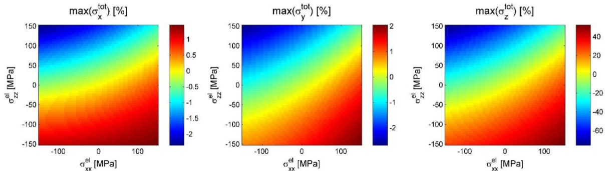
Figure 4.92 : Cartographie des variations d'amplitude maximale des composantes \sigma_x^{tot} (gauche), \sigma_y^{tot} (centre) et \sigma_z^{tot} (droite) de sources induites par EMAT à la surface d'un acier inoxydable AISI 410 en fonction de contraintes bi-axiales ( \sigma_{xx}^{el} , \sigma_{zz}^{el} ).
