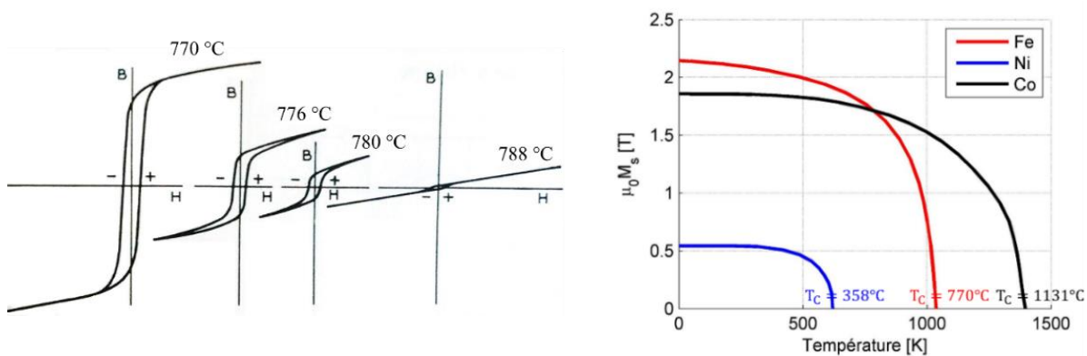
Figure 1.8 : Évolution du cycle d'hystérésis du fer au passage de la température de Curie (gauche [Bozorth_1964]) et variation de l'aimantation à saturation du fer, du nickel, et du cobalt en fonction de la température (droite [Coudérechon_1979]).
