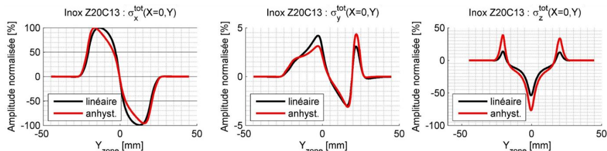
Figure 4.85 : Variations selon X_{zone} des composantes \sigma_x^{tot} (gauche), \sigma_y^{tot} (centre), \sigma_z^{tot} (droite) des sources totales de transduction induites par EMAT pour un acier inoxydable Z20C13 supposé linéaire (noir) ou anhystérétique (rouge).
