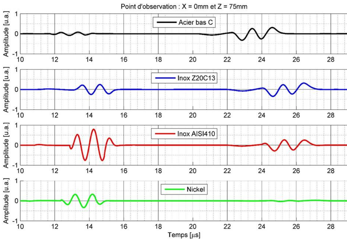
Figure 4.65 : A-scans en champ total (L+T) simulés à partir des sources surfaciques \sigma^{tot} induites par EMAT dans quatre milieux ferromagnétiques différents : acier bas carbone, aciers inoxydables Z20C13 et AISI 410, et nickel (recuit).
