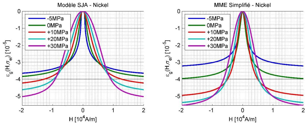
Figure 2.39 : Courbes anhistériques de magnétostriction d'un nickel (recuit) en fonction du champ magnétique appliqué et d'une contrainte mécanique uni-axiale d'après le modèle SJA (gauche) et le MME simplifié (droite).
