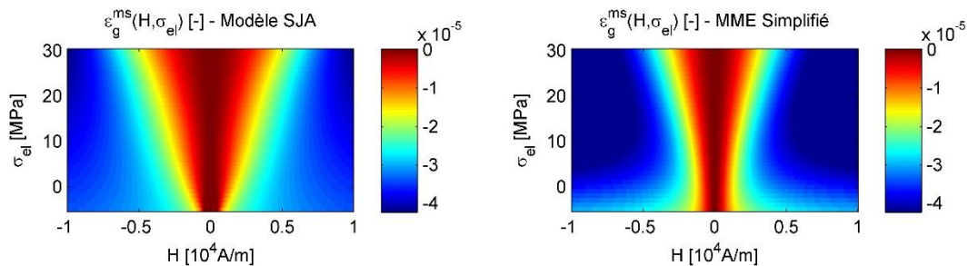
Figure 2.40 : Cartographies des courbes anhistériques de magnétostriction d'un nickel (recuit) en fonction du champ magnétique appliqué et d'une contrainte mécanique uni-axiale d'après le modèle SJA (gauche) et le MME simplifié (droite).
