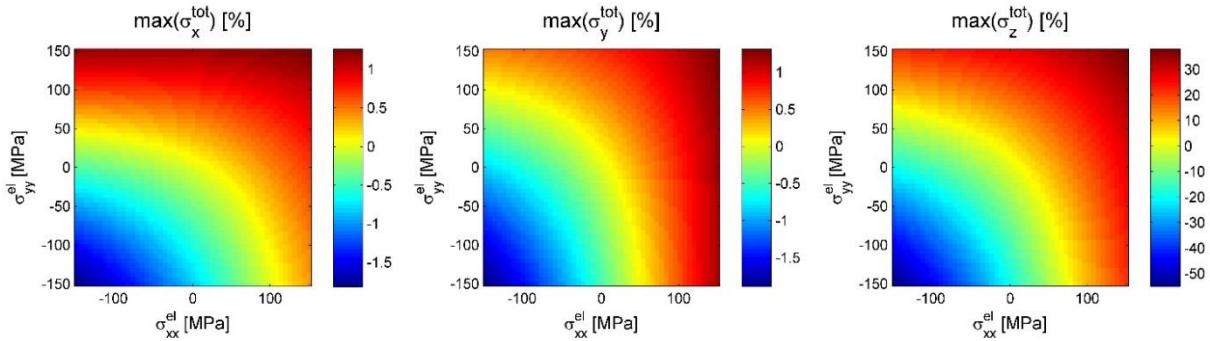
Figure 4.91 : Cartographie des variations d'amplitude maximale des composantes \sigma_x^{tot} (gauche), \sigma_y^{tot} (centre) et \sigma_z^{tot} (droite) de sources induites par EMAT à la surface d'un acier inoxydable AISI 410 en fonction de contraintes bi-axiales ( \sigma_{xx}^{el} , \sigma_{yy}^{el} ).
