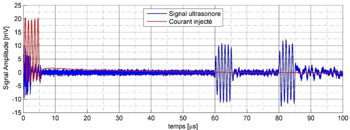
Figure 5.110 : Mesure par un transducteur piézoélectrique focalisé en immersion du champ ultrasonore transmis par EMAT dans une pièce d'acier inoxydable Z20C13 pour une intensité de courant électrique de 2.42A.
