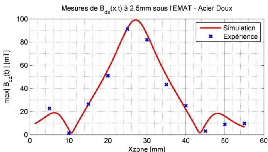
Figure 5.105 : Comparaison entre simulation et mesures des variations spatiales du maximum d'intensité de l'induction magnétique dynamique (normale) rayonnée à 2.5 mm dans l'entrefer entre l'EMAT et un échantillon d' acier doux .
