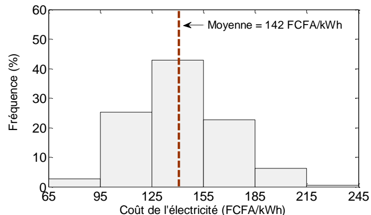
Figure 4-19: Analyse de sensibilité globale montrant la variance du coût de l'électricité pour pour le scénario SC4 (Groupe syngaz 325 kW )
