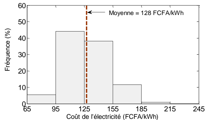
Figure 4-23: Analyse de sensibilité globale montrant la variance du coût de l'électricité pour pour le scénario SC8 (Groupe syngaz 225 kW )
