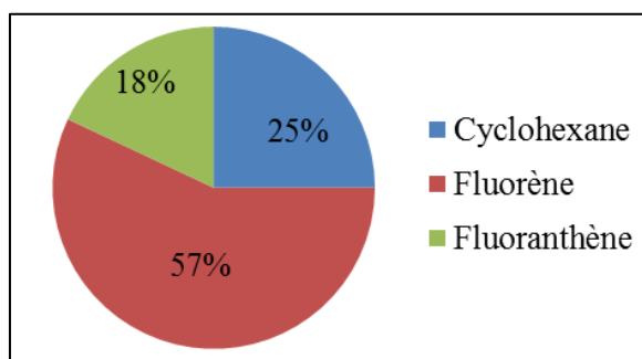
Figure 4-13: Contributeurs à l'impact de la toxicité humaine non cancérigène (THNC)
