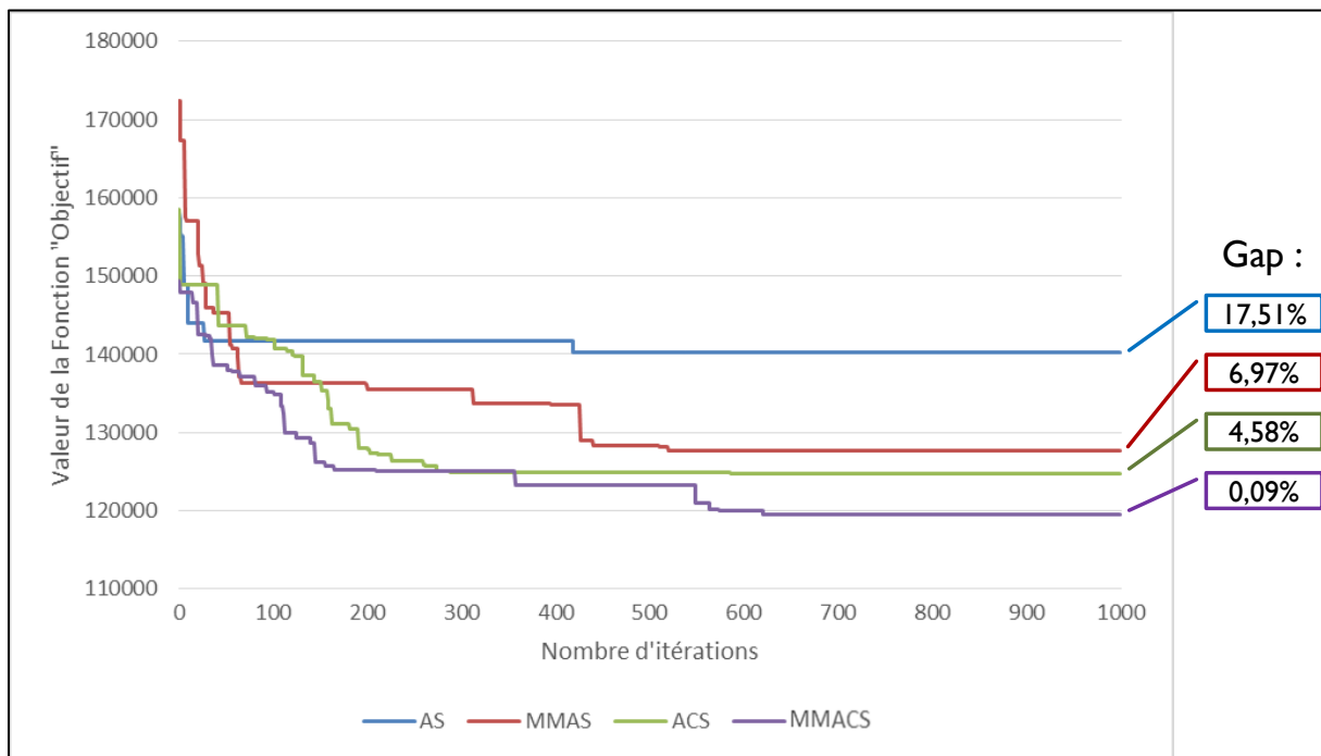
Figure VI.9 : Comparaison de convergence des différentes variantes
