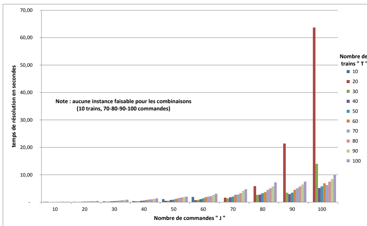
Figure VI.1 : Influence du nombre de trains sur les temps de résolution du PLVM
