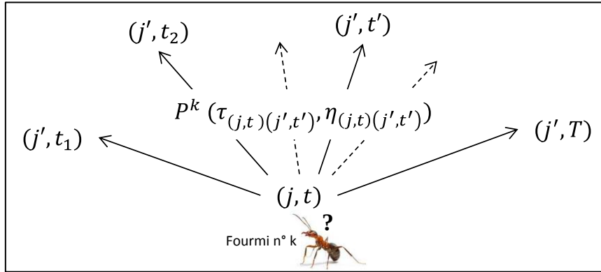
Figure V.3 : Une étape durant le processus de construction d'une solution par une fourmi
