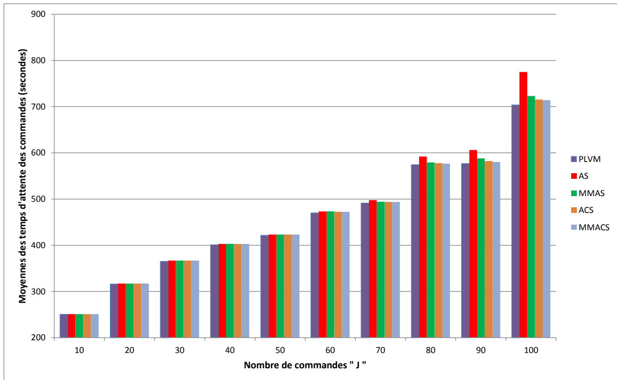
Figure VI.7 : Moyennes des temps d'attente des commandes – Colonies de fourmis VS PLVM
