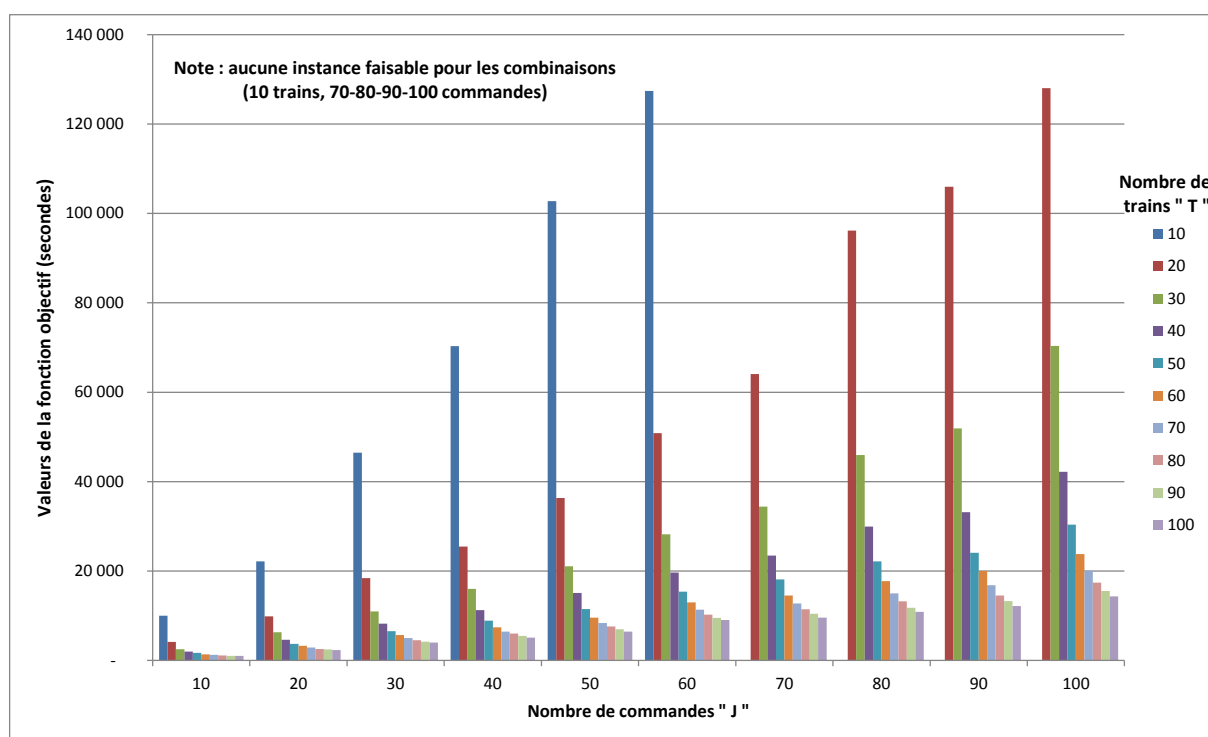
Figure VI.2 : Influence du nombre de trains sur les temps d'attente
