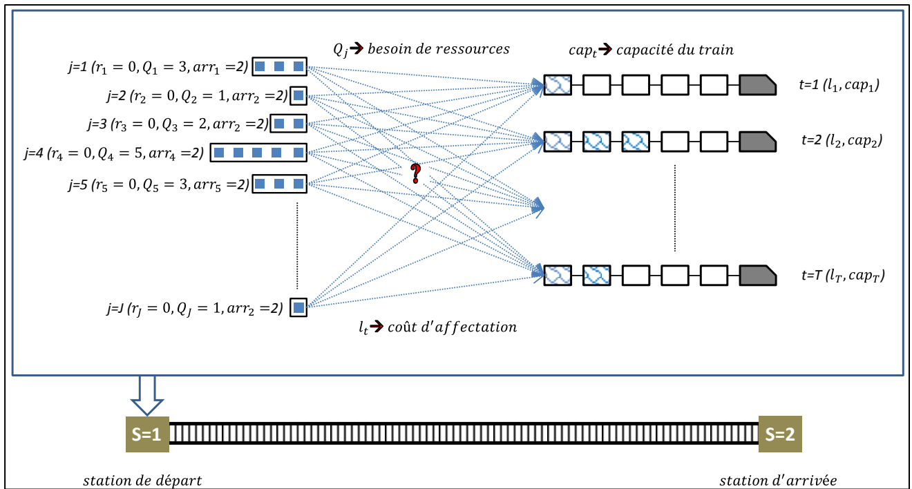
Figure V.2 : Réduction du problème FRTSP à un problème d'affectation généralisée
