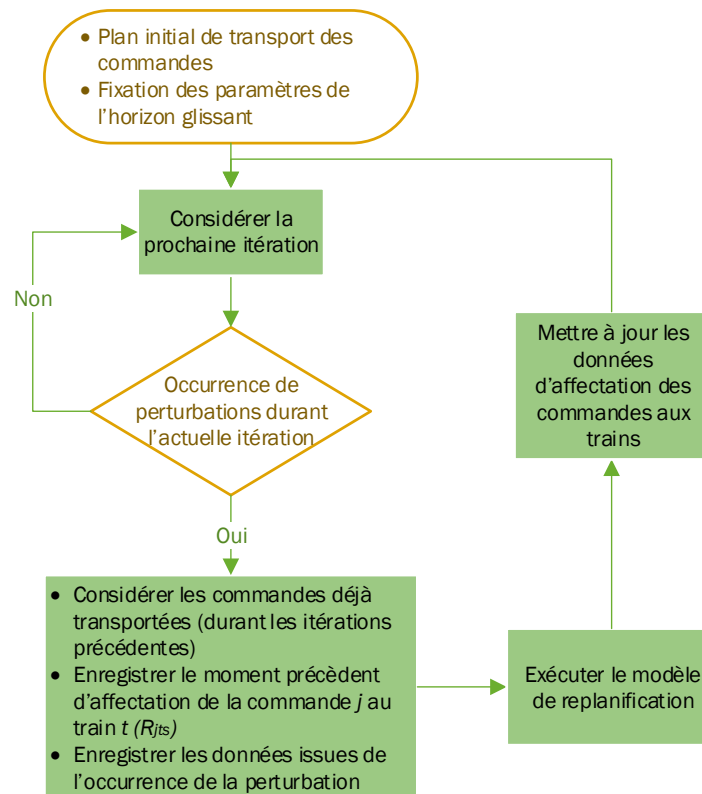
Figure V.4 : La replanification du FRTSP par horizon glissant
