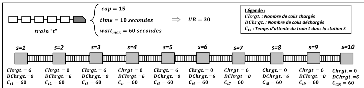
Figure VI.6 : illustration du calcul de « UB »
