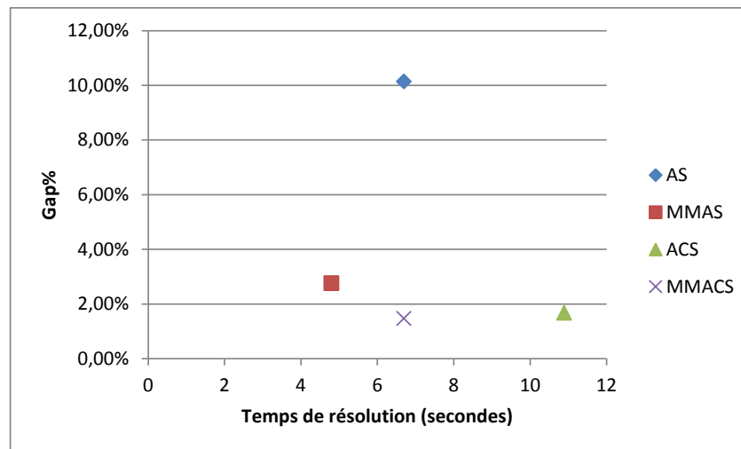
Figure VI.8 : Etude bi-critère des performances des colonies de fourmis
