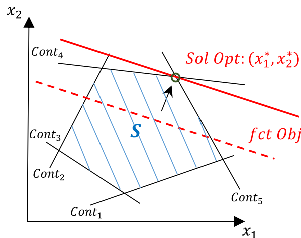
Figure III.3 : Exemple d'une résolution graphique d'un PL à 5 contraintes
