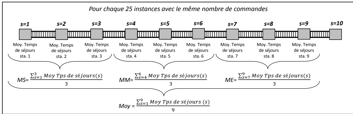
Figure VI.4 : Calculs des temps d'attente moyens
