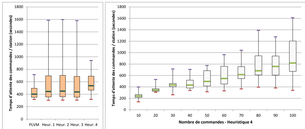
Figure VI.5 : Boîtes à moustaches des temps d'attente des commandes dans les stations – (gauche) comparaison entre les différentes approches, (droite) heuristique 4
