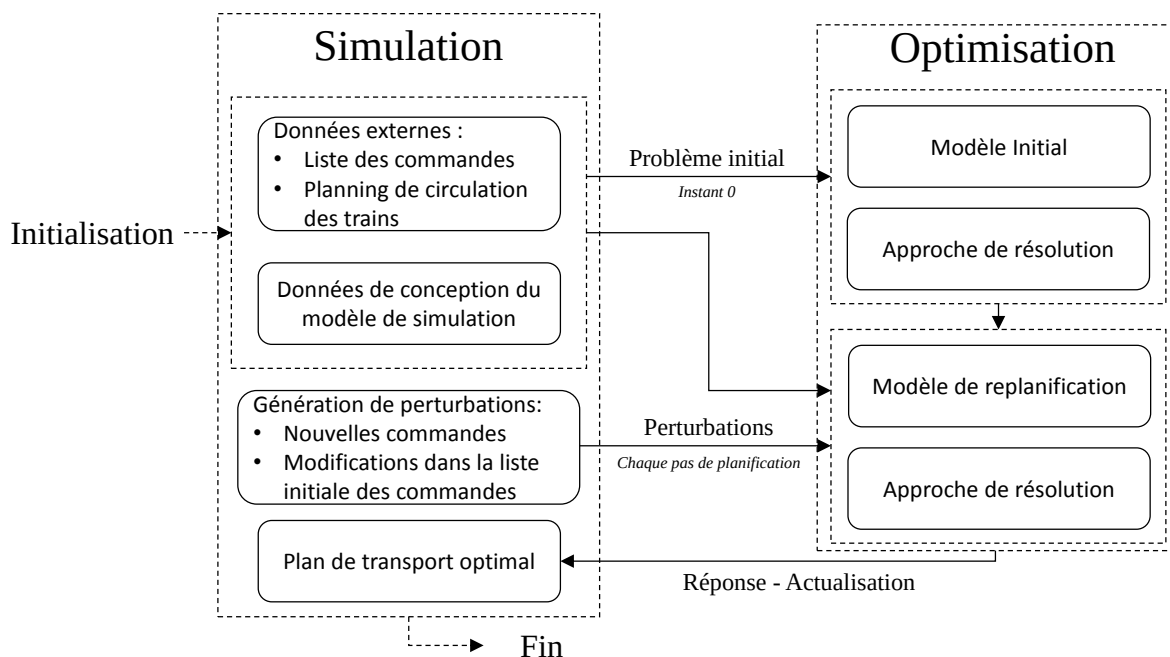
Figure V.6 : Le schéma de couplage dans le cas de la replanification
