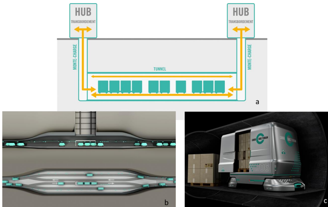
Figure II.2 : Modélisations de Cargo Sous Terrain : a- principe de fonctionnement, b- coupes latérale et horizontale, c- modèle 3D des véhicules en développement (CST, 2016)
