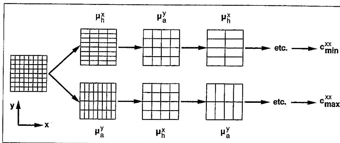
FIGURE 2.6 – Illustration du procédé itératif de le Loc'h (1987) permettant le calcul des bornes c_{max}^{uu} et c_{min}^{uu} à deux dimensions. D'après Renard (1997). La direction principale de l'écoulement est supposée être selon la direction x
