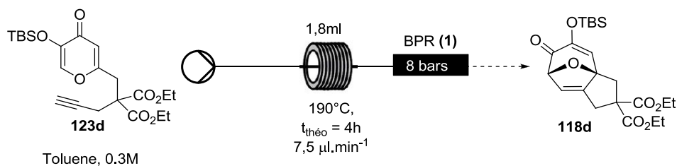
Schéma 122: Première réaction de cycloaddition [5 + 2] en flux continu à 190°C avec l'utilisation du BPR Asia (1) et avec un débit de 7,5 \mu\text{l}.\text{min}^{-1}
