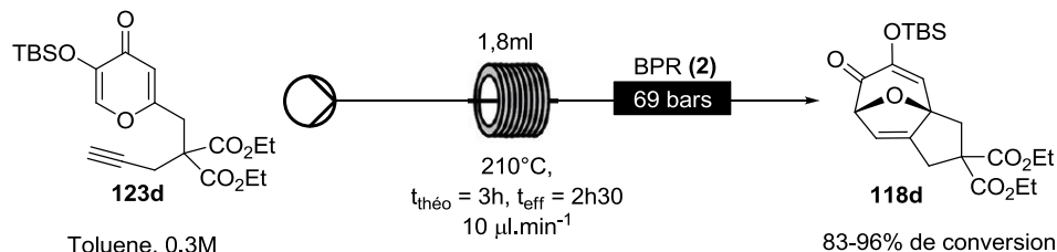
Schéma 124: Cycloaddition en flux continu à 210 °C avec l'utilisation du BPR (2) de 69 bars et avec un débit de 10 \mu l \cdot min^{-1}
