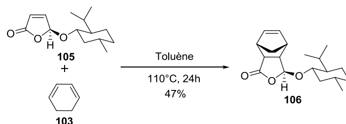
Schéma 43: Synthèse de dérivé de type buténolide chirale 106 par réaction de Diels-Alder 109
