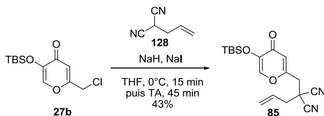
Schéma 63: Alkylation de l'acide chlorokojaïque protégé 27b par l'allylmalononitrile ( 128 )
