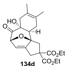
Schéma 133: Structure du composé 134d
