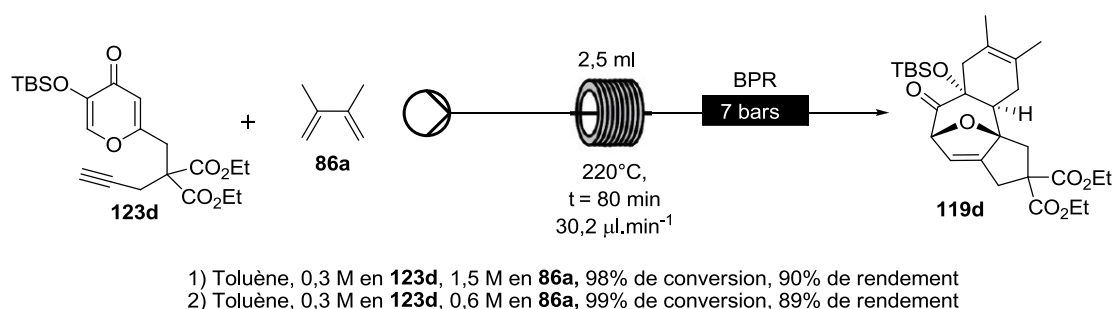
Schéma 130: Réactions de cycloaddition tandem [5 + 2]/[4 + 2] entre l'alcyne 123d et le diène 86a en flux continu avec le dispositif (B) avec variation de la concentration en diène 86a
