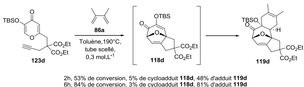
Schéma 119: Réaction de cycloaddition tandem [5 + 2]/[4 + 2] entre l'alcyne 123d et le diène 86a en tube scellé avec variation du temps de réaction
