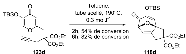
Schéma 93: Réaction de cycloaddition [5 + 2] sur l'alcyne 123d en tube scellé avec variation du temps de réaction
