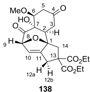
Schéma 117: Structure de la molécule 137d et numérotation pour l'attribution en RMN
