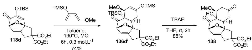
Schéma 116: Réaction de Diels-Alder entre le cycloadduit 118d et le diène de Danieshefsky suivi de la déprotection des éthers d'énol silylés conduisant au tricyclic 138
