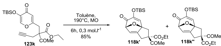
Schéma 98: Cycloaddition [5 + 2] de l'alcyne 123k possédant comme substituant COMe et CO 2 Et et conduisant aux deux adduits 118k' et 118k''
