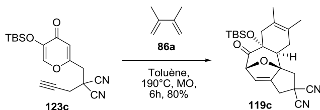
Schéma 120: Cycloaddition tandem [5 + 2]/[4 + 2] entre l'alcyne 123c et le diméthylbutadiène 86a pour l'accès au tricycle ponté 119c
