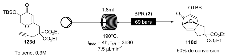
Schéma 123: Réaction de cycloaddition [5 + 2] en flux continu à 190°C avec l'utilisation du BPR Asia (2) et avec un débit de 7,5 \mu l \cdot min^{-1}
