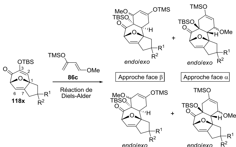
Schéma 106: Cycloadduits théoriques formés par réaction de Diels-Alder entre le cycloadduit 118x et le diène de Danieshefsky 86c
