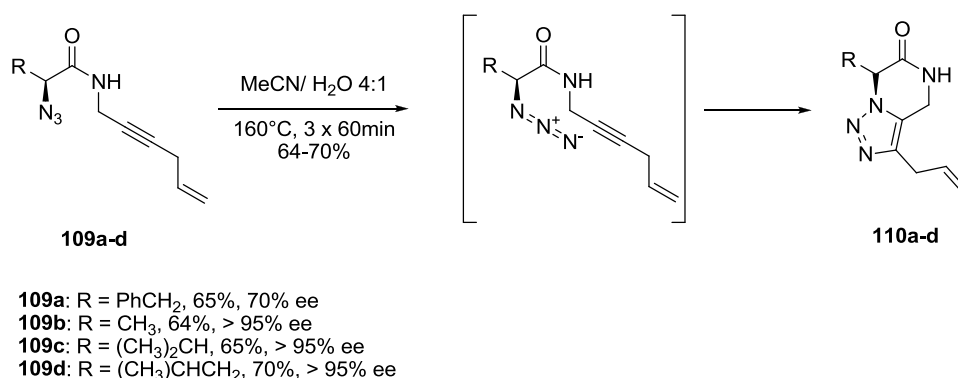
Schéma 45: Synthèse des triazoles 110a-d par cycloaddition de Huisgen
