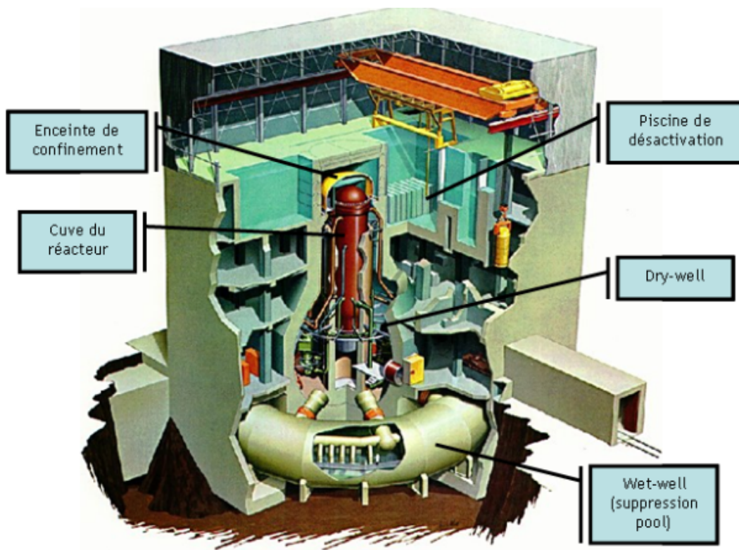
Figure n°14 : schéma de l'intérieur d'un bâtiment d'un REB ( Ibid. ).
