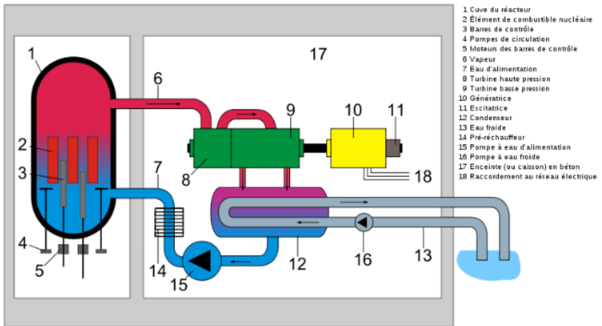
Figure n°13 : schéma des éléments composant un réacteur à eau bouillante (IRSN, 2012a).
