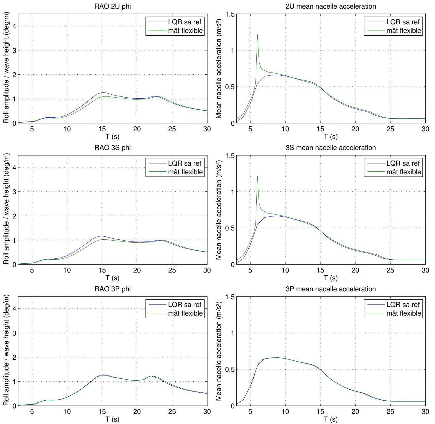
FIGURE D.3 – RAO en roulis, à gauche, accélération moyenne de la nacelle, à droite, sur le modèle complet en “LQR saturé” pour une houle monochromatique, pour un mât flexible
