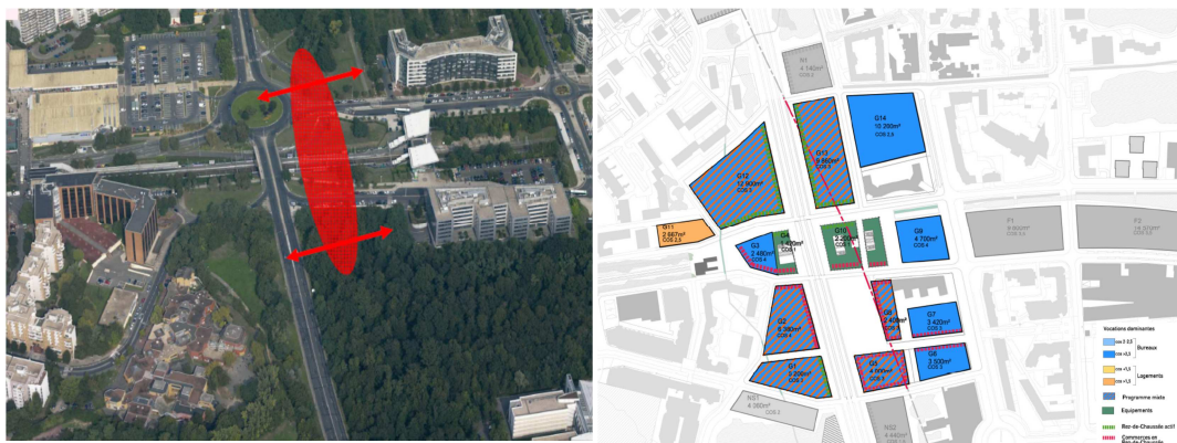
Figure 8.2 : (a) État actuel et zone d'implantation de la gare (source : SGP, 2012), (b) Son plan programme (source : Ateliers Lion, avril 2013).
