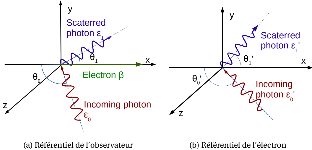
FIGURE 6.1 – Diffusion d'un photon dans le référentiel de l'observateur (a) et dans le référentiel de l'électron (b).
