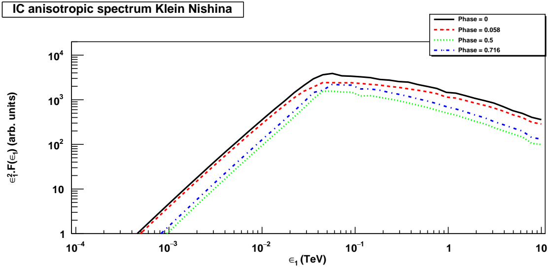
FIGURE 6.6 – Modélisation du spectre LS 5039 dans le cas d'une diffusion inverse Compton en régime de Klein-Nishina pour une inclinaison de 30^\circ et aux mêmes positions particulières de l'objet compact que pour la figure 6.5. Les échelles d'énergie sont différentes. Les fluctuations de la courbe correspondant à la conjonction supérieure correspondent à des incertitudes de la simulation.
