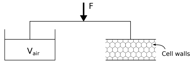
FIGURE 3.10 – Modèle proposé par SKOCHDOPOLE et RUBENS [1965] parallélisant la contribution de la microstructure, et de la pression de l'air dans les cellules.
