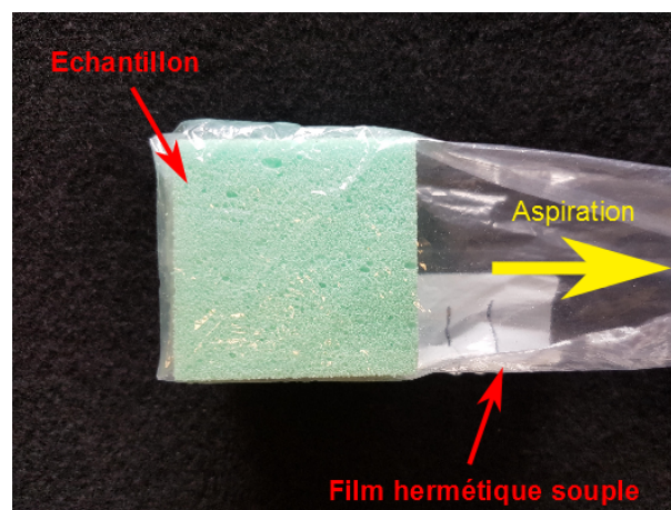
FIGURE 3.12 – Illustration du film hermétique utilisé pour envelopper les échantillons.
