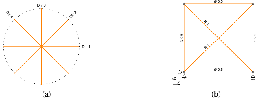
FIGURE 4.43 – Illustration des directions de discrétisation d'un élément 2D, utilisées dans cette étude (a). Maillage éléments finis reprenant les directions de discrétisation (b).
