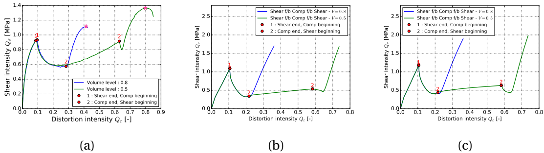
FIGURE 4.60 – Contribution en changement de volume obtenue expérimentalement (a), par simulation avec une loi de comportement Hyperélastique (b) et Hyperélasto-Visqueuse (c), pour une sollicitation "Shear f/b Comp f/b shear".
