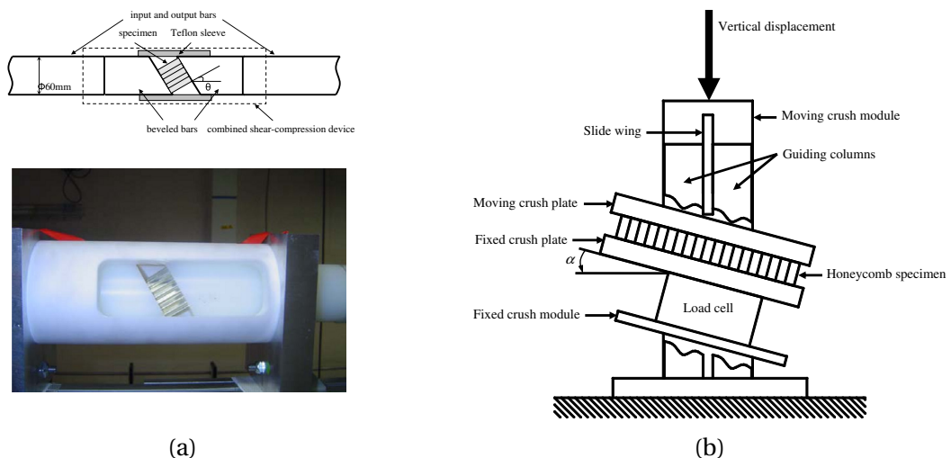
FIGURE 4.2 – Système de sollicitation par plateaux inclinés développé par HOU et collab. [2011] (a), et HONG et collab. [2008] (b).
