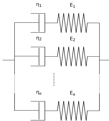
FIGURE 4.46 – Modèle rhéologique de Maxwell généralisé
