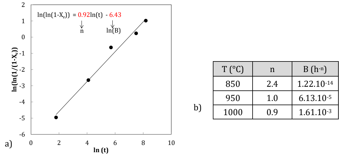
Figure 2.32 – a) Courbe permettant l'obtention des coefficients n et B à partir de la fraction de grains recrystallisés et du temps de maintien à 1000°C et b) tableau récapitulatif des coefficients de la loi JMAK pour différentes températures.
