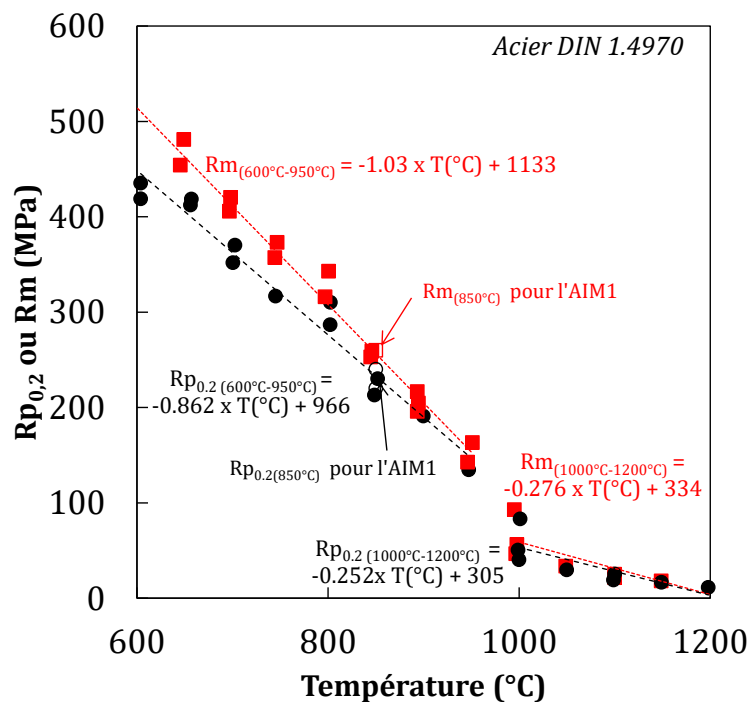
Figure 4.1- Evolutions de la limite d'élasticité et de la résistance mécanique maximale avant rupture en fonction de la température (vitesse de déformation initiale = 3.10^{-4}s^{-1} ), données tirées de (Petersen, Schanz, et Leistikow 1988).
