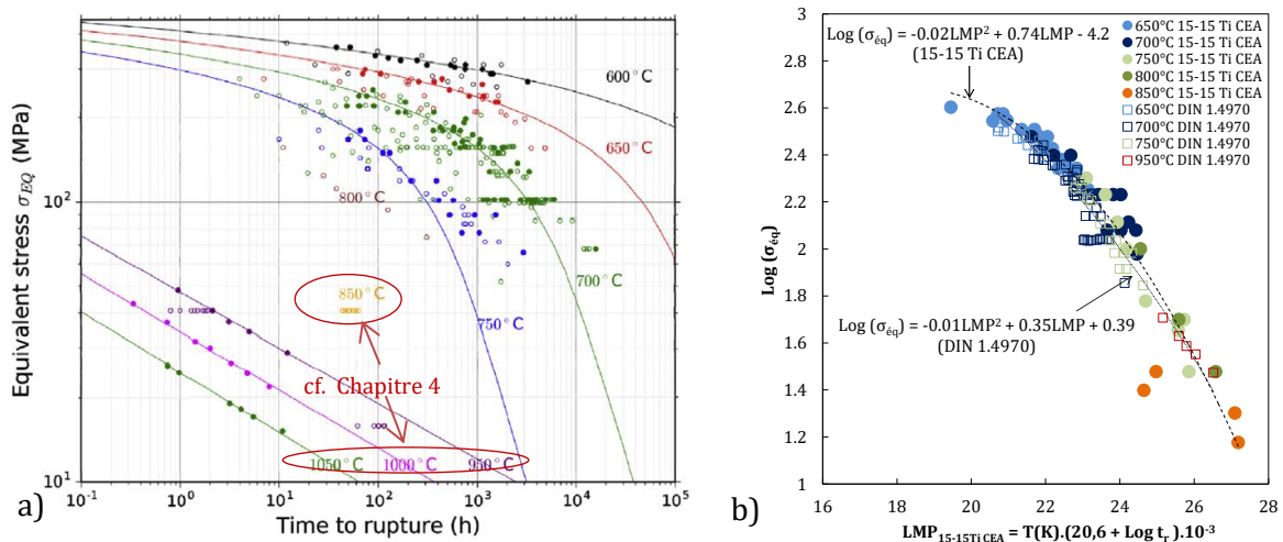
Figure 3.11 – a) Graphique représentant la contrainte équivalente en fonction du temps à rupture, d'après (Cautaeys et al. 2017) tiré des données de (Schäfer et Kempe 1983) et b) représentation permettant la prédiction du temps à rupture en fonction de la contrainte équivalente et du paramètre LMP pour les 15-15Ti testés au CEA (marqueurs circulaires et pleins) et pour le DIN 1.4970 (marqueurs rectangulaires et vides), d'après le graphique de la Figure 3.9 a.
