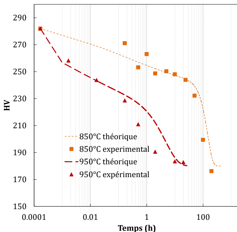
Figure 2.41 - Evolutions de la dureté modélisée et expérimentale en fonction du temps à 850°C et à 950°C.
