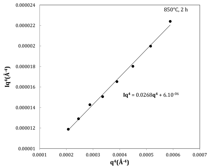
Figure A3.4 – Détermination du bruit de fond pour l'échantillon 850°C, 2 h.
