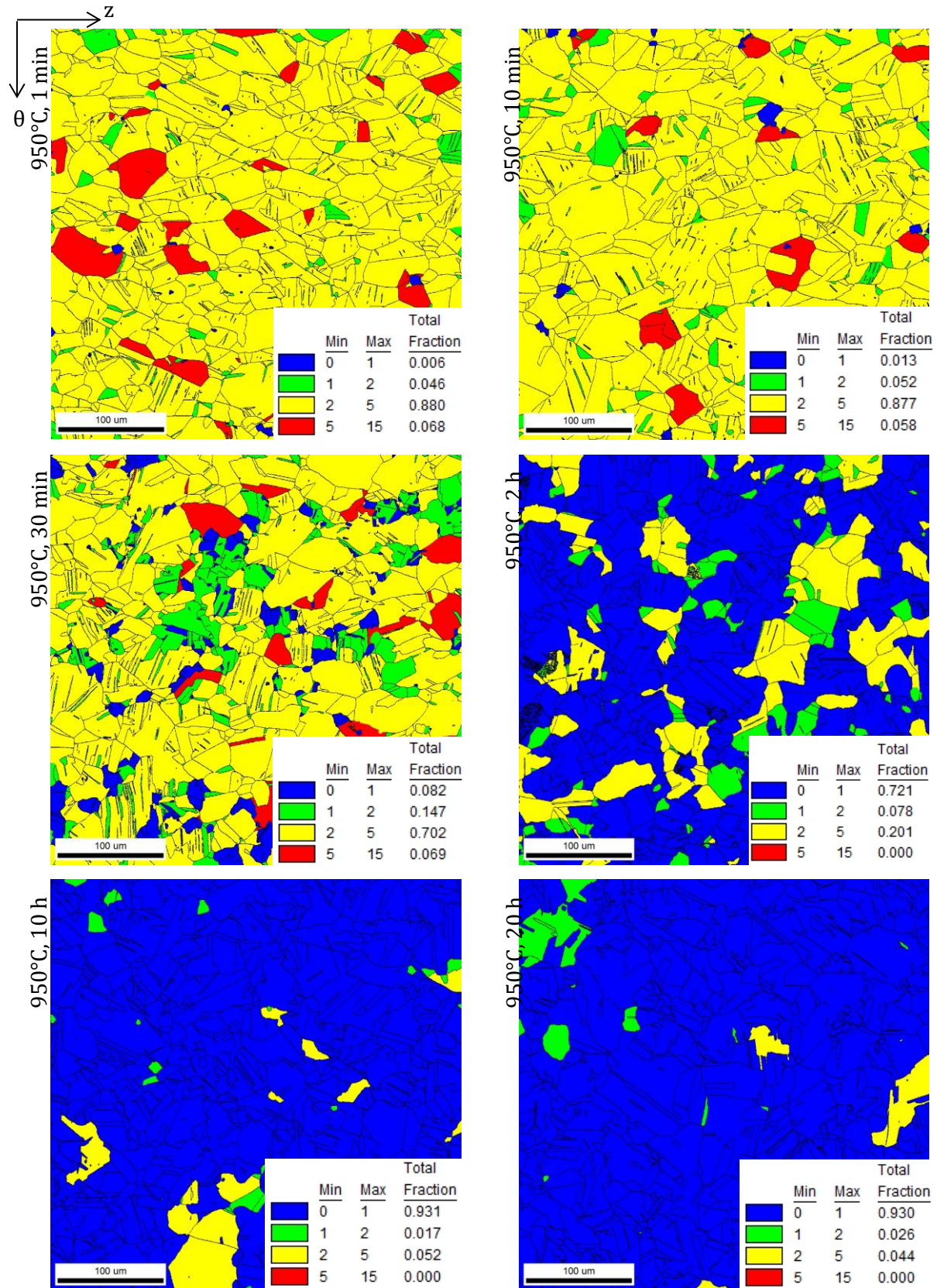
Figure 2.30 – Cartographies GOS dans le plan ( \theta, z ) montrant l'évolution de la recrystallisation en fonction du temps de maintien à 950°C.
