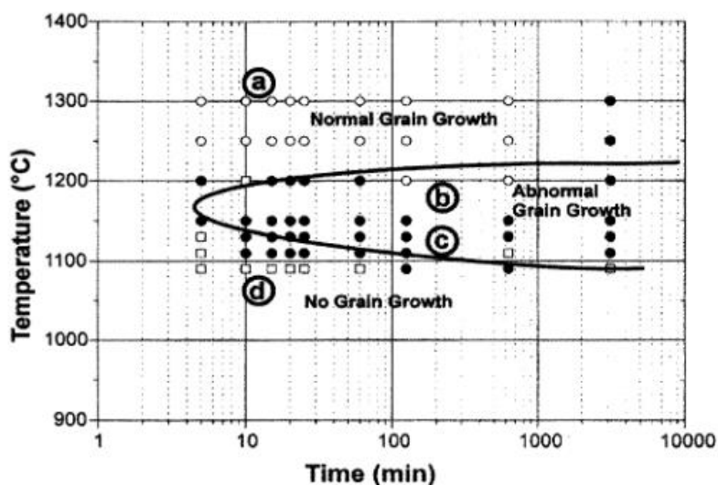
Figure 2.12 – Diagramme température-temps représentant les domaines de croissance normale et anormale des grains recristallisés pour un acier DIN 1.4970 (taux d'écroissage à froid non mentionné) (Padilha, Plaut, et Rios 2003).
