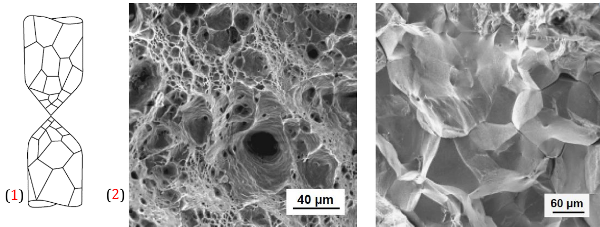
Figure 3.5 – (1) Schéma d'une rupture 100% ductile (Courtney 2000) et fractographies montrant (2) une rupture transgranulaire ductile d'un acier 316L(N) hypertrempé et testé en traction à 600°C (vitesse de déformation = 5.10^{-4}s^{-1} ) et (3) une rupture intergranulaire fragile sur une éprouvette en acier 316H hypertrempé testée à 600°C ( t_r = 45,7 h), d'après (Auzoux 2004).
