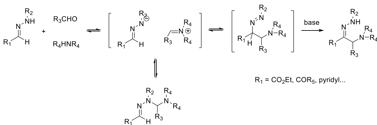
schéma 5
