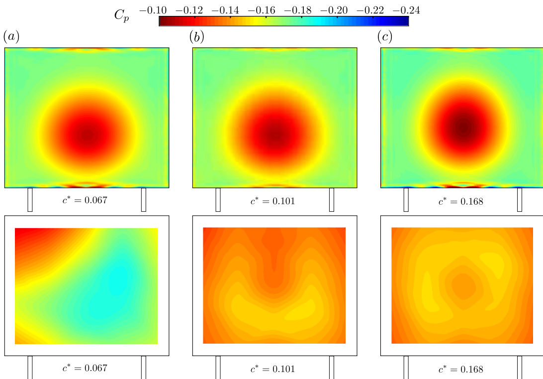
Figure 9 – En haut, distributions de pression moyenne au culot C_p(y^*, z^*) pour le corps d'Ahed à culot droit ( \alpha = \beta = 0^\circ ) à différentes gardes au sol : (a) c^* = 0.067 (b) c^* = 0.101 (c) c^* = 0.168 . En bas, distributions équivalentes pour le cas avec cavité de profondeur d = 0.285 H observées expérimentalement (voir annexe B).
