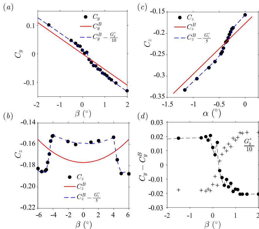
Figure 5 – Coefficient d’effort transverse en fonction de l’angle du corps : (a) effort latéral C_y en fonction de l’angle de dérapage \beta (instabilité y ), (b) effort latéral C_y en fonction de l’angle de dérapage \beta (instabilité z ), (c) coefficient de portance C_z en fonction de l’angle d’assiette \alpha (instabilité z ). (d) Contribution de l’instabilité au chargement aérodynamique du cas (a) et gradient de pression au culot. Points noirs : mesures ; ligne continue rouge : chargement de l’écoulement de base sans instabilité ; ligne discontinue bleue : modèle des équations (3b) et (3a).
