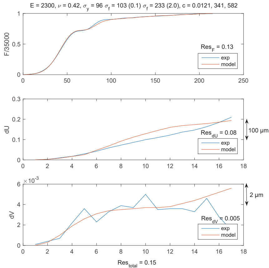
Figure V.14: Comparaison expérience/identification de F , dU et dV . Boucle d'identification 1 bis. Essai à 45°
