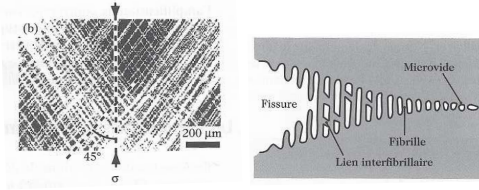
Figure I.2: Bandes de cisaillement en microscopie (gauche) et schéma d’une craquelure (droite) [Halary and Lauprêtre, 2015]
