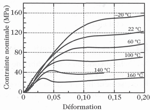
Figure I.1: Courbe contrainte-déformation à 10^{-3} s^{-1} pour une résine époxy [Halary and Lauprêtre, 2015]
