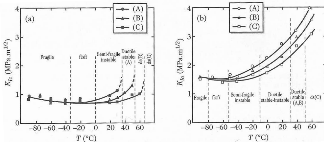
Figure I.3: Variation de K_{IC} avec la température pour une résine époxy/élastomère à trois vitesses de déplacement : (A) : 8.33 \cdot 10^{-7} , (B) : 1.67 \cdot 10^{-5} (C) : 1.67 \cdot 10^{-4} \text{ m}\cdot\text{s}^{-1} . (a) résine pure; (b) résine avec élastomère [Halary and Lauprêtre, 2015]
