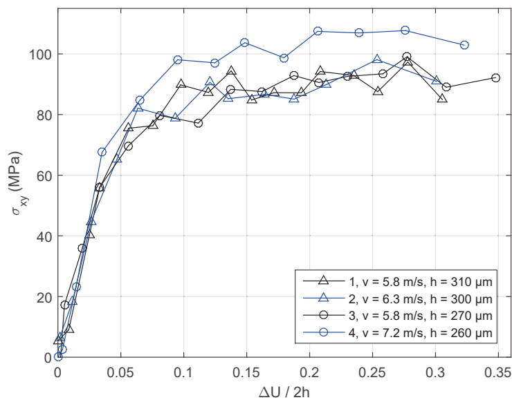
Figure III.14: Contrainte de cisaillement dérivée de la corrélation d'images en fonction de la déformation de cisaillement au milieu du joint adhésif. Essais à 45°
