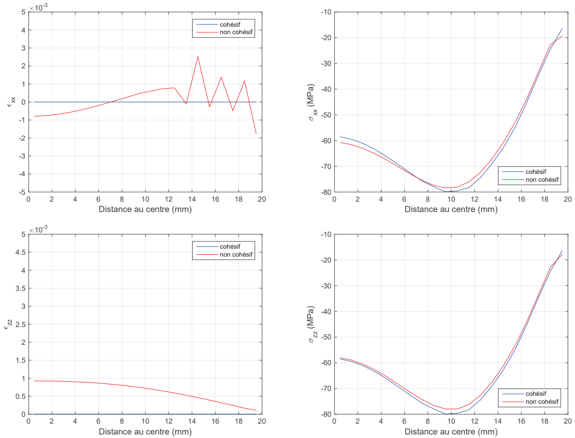
Figure F.2: États de déformation et de contrainte secondaires dans le joint
