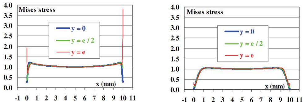
Figure I.9: Contrainte de Von Mises normalisée le long du joint ;gauche : éprouvette TAST, droite : éprouvette TAST avec becs fins [Cognard et al., 2008]
