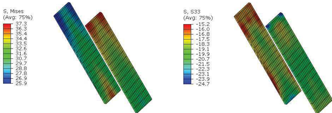
Figure VI.4: Simulation numérique : états de contrainte des deux joints dans l'éprouvette BIADH45 en compression dynamique
