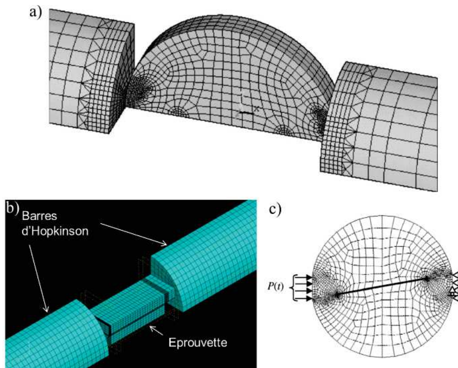
Figure IV.1: Différentes modélisations numériques utilisées aux barres d'Hopkinson : a) Dong et al. [2006], b) Challita and Othman [2010], c) Wang et al. [2011]
