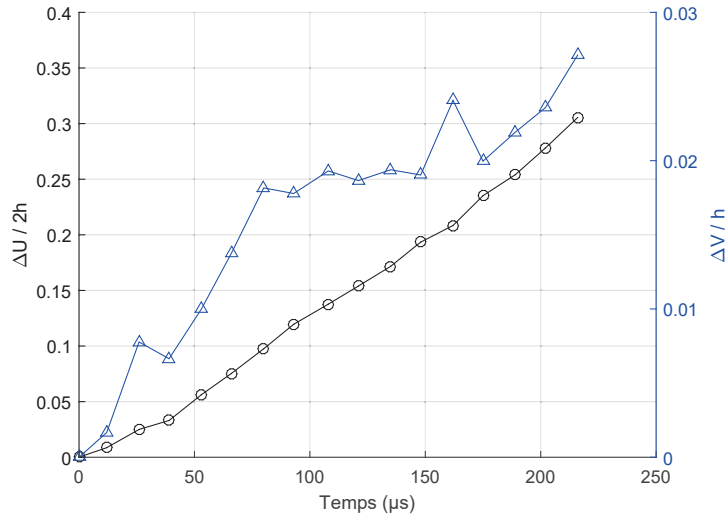
Figure III.3: Évolutions temporelles des déformations de cisaillement et de compression au milieu du joint adhésif pour un essai à 45° à v = 5.8 \text{ m/s}
