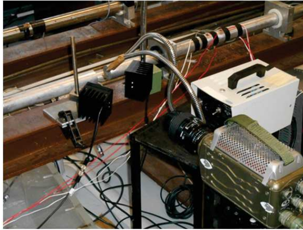
Figure B.1: Photo du dispositif expérimental avec l'éclairage e1 : 2 panneaux LED + 2 flexibles
