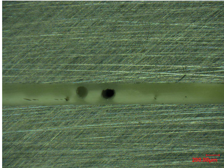
Figure III.11: Photo du milieu du joint après essai à 75^\circ sur éprouvette DODECA complète
