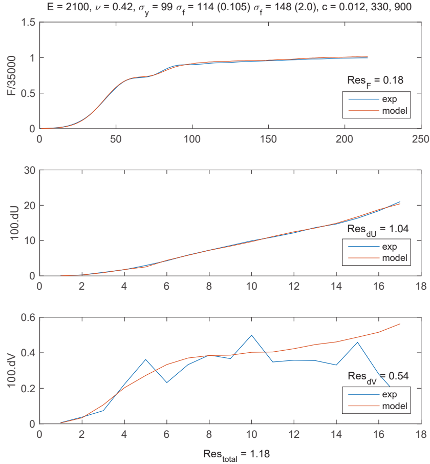
Figure V.16: Comparaison expérience/identification de F , dU et dV . Essai à 45^\circ
