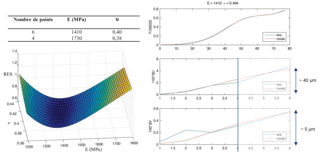
Figure V.7: Résultats du calcul inverse sur E et \nu
