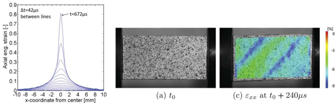
Figure II.8: Évolution de la déformation axiale en fonction de la distance au centre de l'éprouvette [Roth et al., 2015]; Champ de déformation d'un composite aux barres d'Hopkinson [Koerber et al., 2010]
