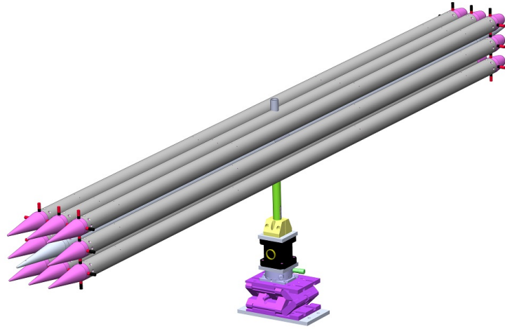
Fig. 3.19 – Aperçu CAO de la maquette FICEL, sans les parois de la veine (réalisé par Nicolas de Buretel de Chassesey dans SolidWorks).
