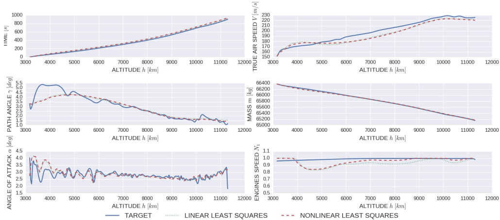
Figure 1.7 – Resimulation d'un vol réel (bleu) en utilisant les dynamiques estimées par des moindres carrés linéaires (vert) et non linéaires (rouge).
