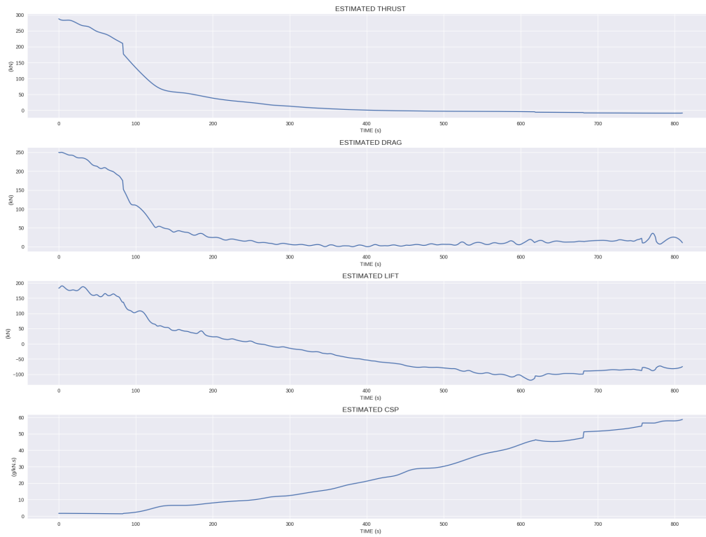
Figure 4.13 – Estimated forces using the ALS solutions.
