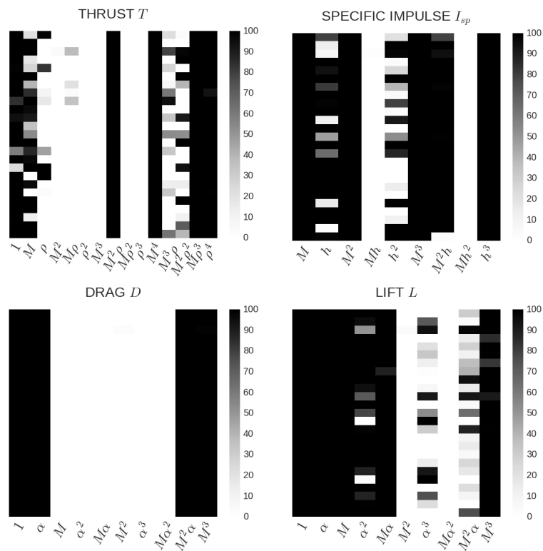
Figure 1.8 – Variables sélectionnées pour la poussée, traînée, portance and impulsion spécifique. Les lignes correspondent à des avions différents, tandis que les colonnes correspondent aux monômes possibles pour T/N_1 , D/q , L/q and I_{sp}/SAT . La couleur des cellules encode la fréquence de sélection de chaque variable pour chaque avion.
