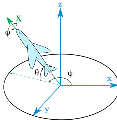
Figure 1.5 – Angles d'Euler avec certaines conventions. 12
