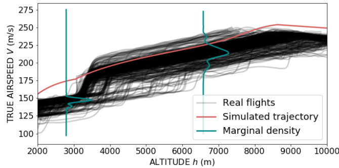
Figure 1.9 – Illustration des vraisemblances marginales.
