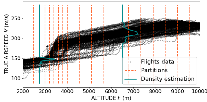
Figure 1.10 – Illustration de l'estimation de vraisemblances marginales.
