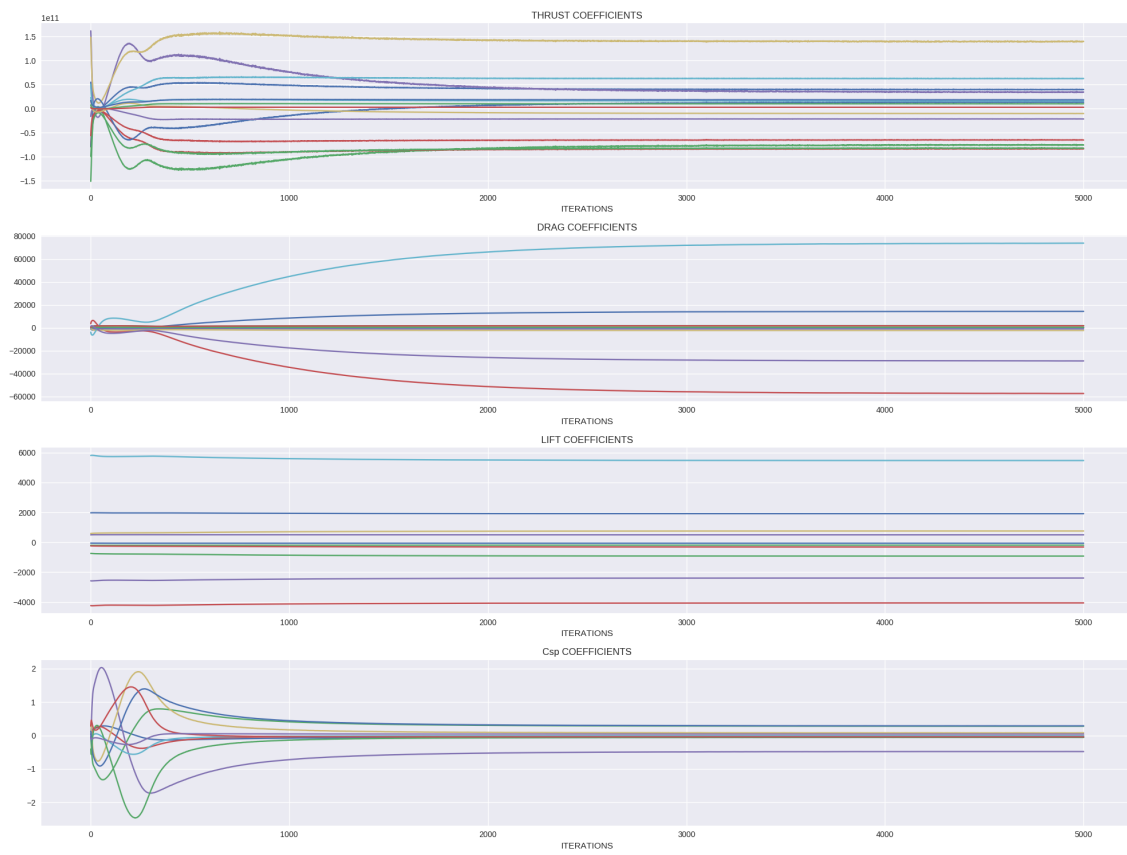
Figure 4.11 – Evolution of the parameters over ALS iterations.
