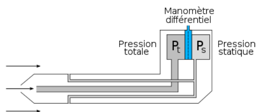
Figure 1.4 – Fonctionnement d’une sonde de Pitot. 11
