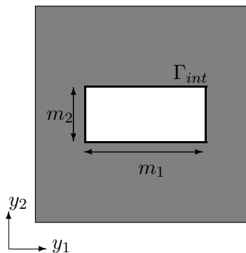
Figure 3: Exemple d'un matériau lattice périodique paramétré : une cellule périodique carrée est percée d'un trou rectangulaire, dont les dimensions paramètrent la géométrie de la microstructure
