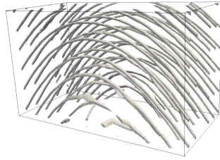
(d) \Omega_{12} = \Omega_1 \cap \Omega_2
