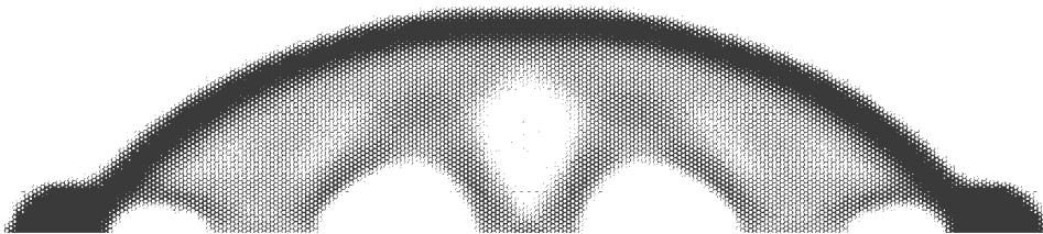
(d) \varepsilon = 0.5
