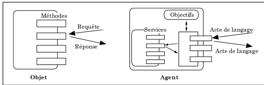
Figure 27. Comparaison de fonctionnement entre un objet et un agent (Ferber, 1997)
