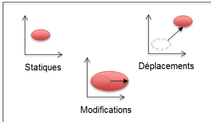
Figure 25. Typologie des dynamiques spatiales
