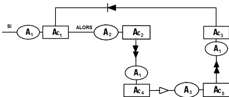
Figure 24 : Algorithme de l'instrument I_0
