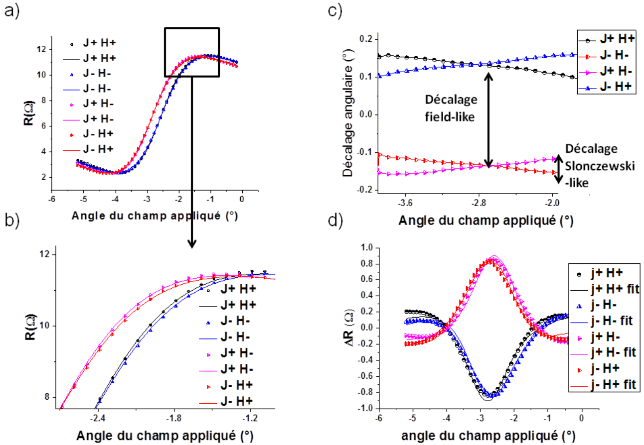
FIGURE 6.17 – Mesures et ajustements numériques des variations angulaires hors-plan de la résistance [selon les 4 protocoles : (H+,j+), (H-,j+), (H-,j-), (H-,j+)] du pont mettant en évidence les couples de transfert de spin dans la structure P9528. Le champ magnétique appliqué est de 380 mT, le courant injecté est de 60mA, et la température est de T=12K . Nous faisons figurer ici les mesures expérimentales (symboles) et les ajustements numériques (traits continus) impliquant les couples de transfert de spin. La sous-figure a) représente la variation angulaire aux abords de la configuration champ perpendiculaire hors du plan. La sous-figure b) est un agrandissement de la sous-figure a) faisant apparaître les différences entre les 4 protocoles. La sous-figure c) représente les décalages angulaires mesurés (décalage en abscisse avec la courbe moyenne des 4 protocoles) et la sous-figure d) représente les décalages en résistance (décalage en ordonnée avec la courbe moyenne des 4 protocoles)
