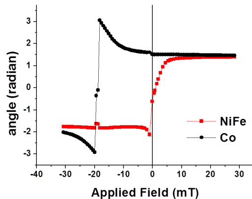
(d) Angles d'aimantation des couches NiFe et Co : reconstitution du comportement des couches magnétiques au cours du cycle R(H) .
