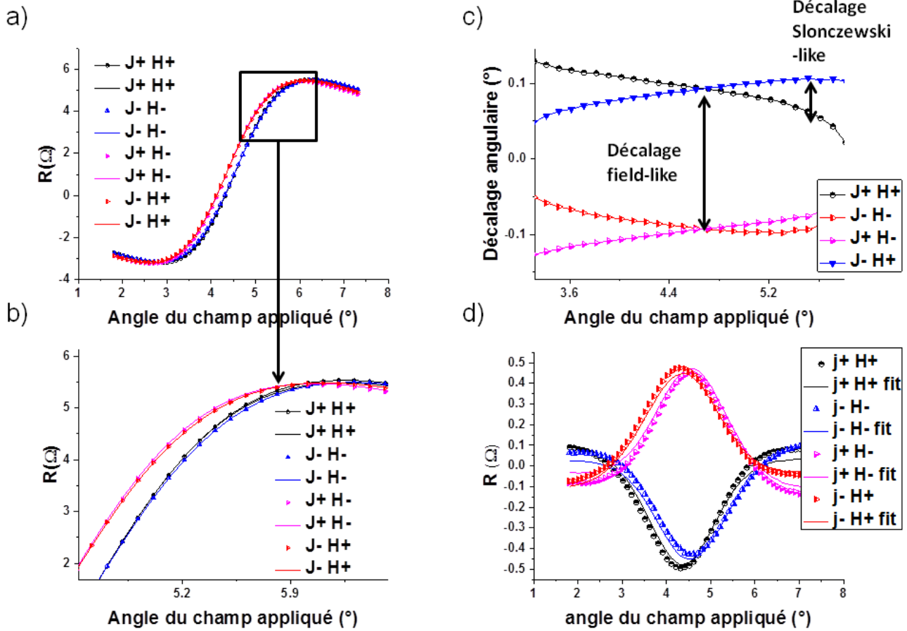
FIGURE 6.18 – Mesures et ajustements numériques des variations angulaires hors-plan de la résistance [selon les 4 protocoles : (H+,j+) , (H-,j+) , (H-,j-) , (H+,j-) ] du pont mettant en évidence les couples de transfert de spin dans la structure P9530. Le champ magnétique appliqué est de 380 mT, le courant injecté est de 60mA, et la température est de T=12 K. Nous faisons figurer ici les mesures expérimentales (symboles) et les ajustements numériques (traits continus) impliquant les couples de transfert de spin. La sous-figure a) représente la variation angulaire aux abords de la configuration champ perpendiculaire hors du plan. La sous-figure b) est un agrandissement de la sous-figure a) faisant apparaître les différences entre les 4 protocoles. La sous-figure c) représente les décalages angulaires mesurés (décalage en abscisse avec la courbe moyenne des 4 protocoles) et la sous-figure d) représente les décalages en résistance (décalage en ordonnée avec la courbe moyenne des 4 protocoles)
