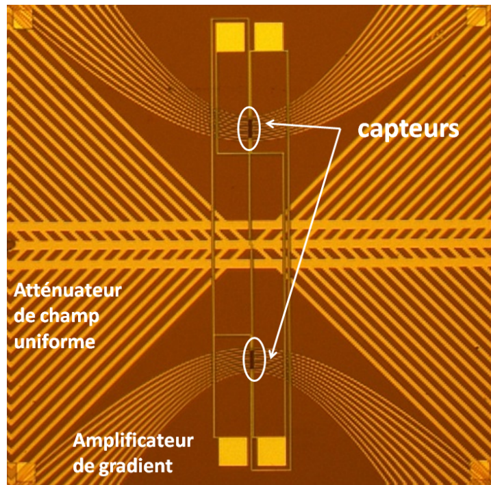
FIGURE 5.24 – Gradiomètre doté de concentrateurs de flux (5 mm × 5 mm). On distingue les bandes droites servant à dévier le champ uniforme et les bandes en forme d'hyperboles destinées à amplifier le gradient
