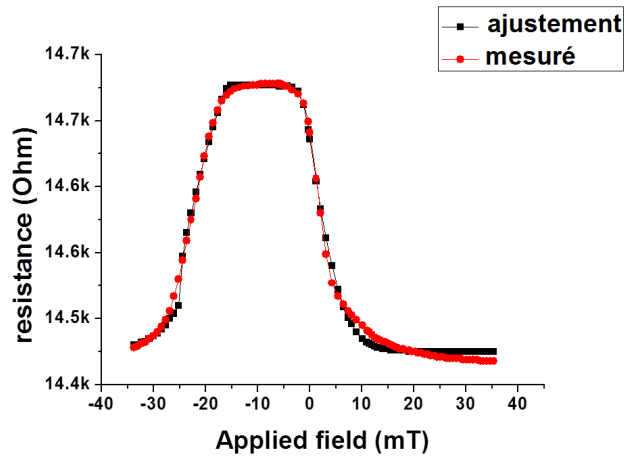
(b) Courbe de transfert d'un capteur W2G5 et ajustement numérique obtenu pour H_{s1} = 37 \text{ G} , H_{s2} = 70 \text{ G} , K_{exc} = 22 \text{ G} , H_{exc} = 198 \text{ G} , H_p = 29 \text{ G} , H_m = 41 \text{ G} , \delta = 9^\circ (désorientation de recuit), R_m = 14 \text{ k}\Omega , GMR = 1.3\% .
