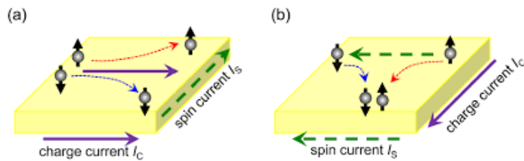
FIGURE 6.6 – Schemas de principe de l'effet Hall de spin et l'effet Hall de spin inverse a) Effet Hall de spin et b) effet Hall de spin inverse. Dans le cas de l'effet Hall de spin inverse, un courant de spin conduit à l'existence d'un courant de charge transverse.
