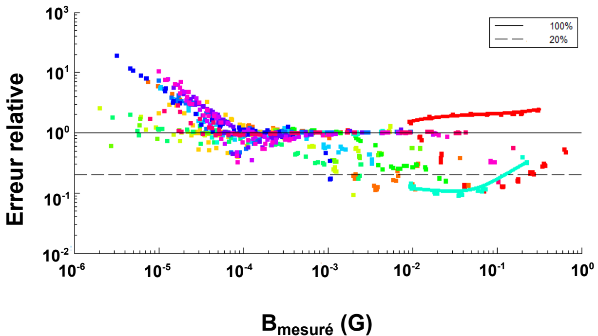
FIGURE 1.8 – Erreur relative après reconstruction du champ : La reconstruction n'est pas satisfaisante pour les longues distances, cependant pour les perturbations situées entre 10 et 50 cm nous pouvons obtenir une reconstruction pouvant atteindre une précision de 20%.
